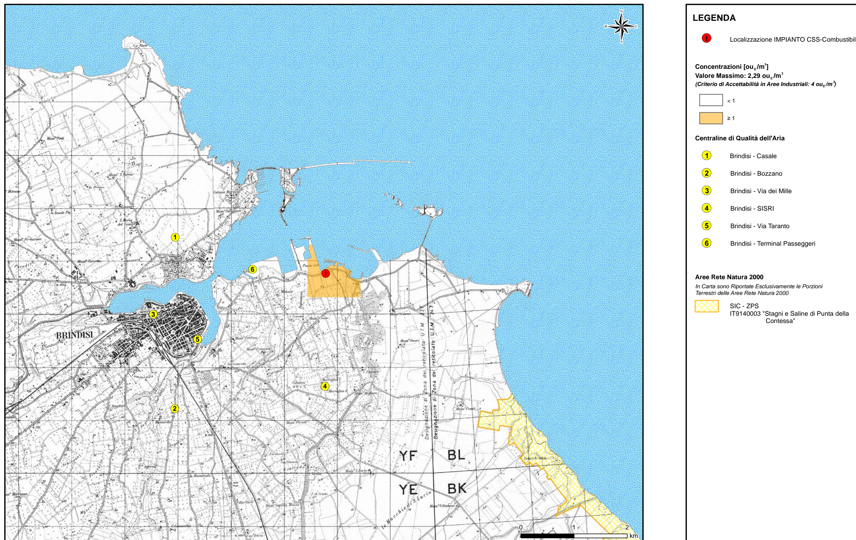
Figura A4.5.1b 98° Percentile delle Concentrazioni di Picco di Odore - Impianto di Produzione CSS-Combustibile + CTE Edipower in Assetto co-Combustione Carbone CSS-Combustibile - Scenario Portata Massima
