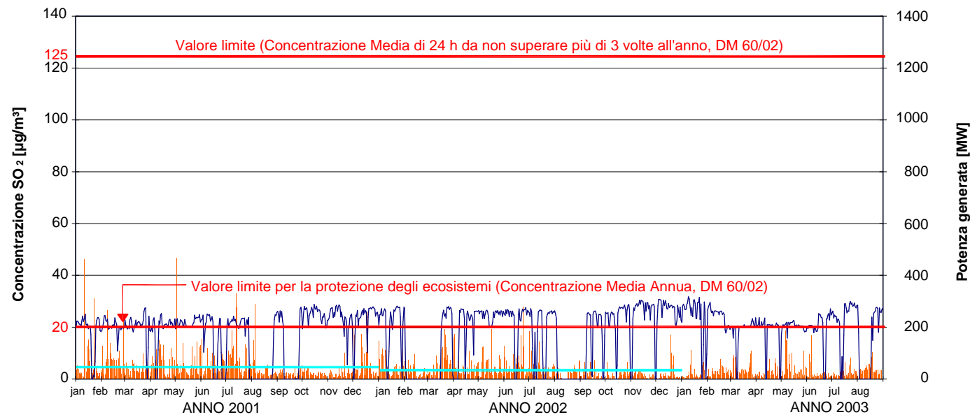
CONCENTRAZIONI MEDIE GIORNALIERE DI SO 2 Postazione No. 2 in località Tutturano
