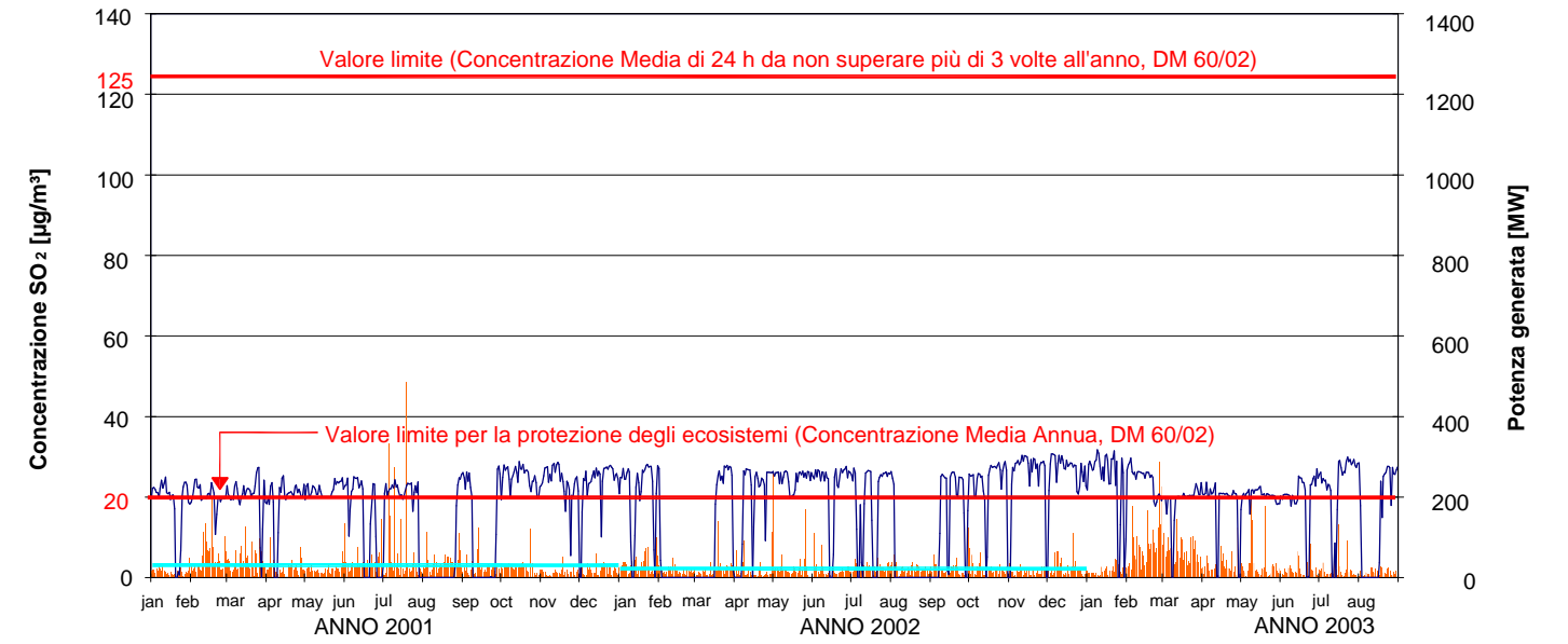
CONCENTRAZIONI MEDIE GIORNALIERE DI SO 2 Postazione No. 4 in località Centro
