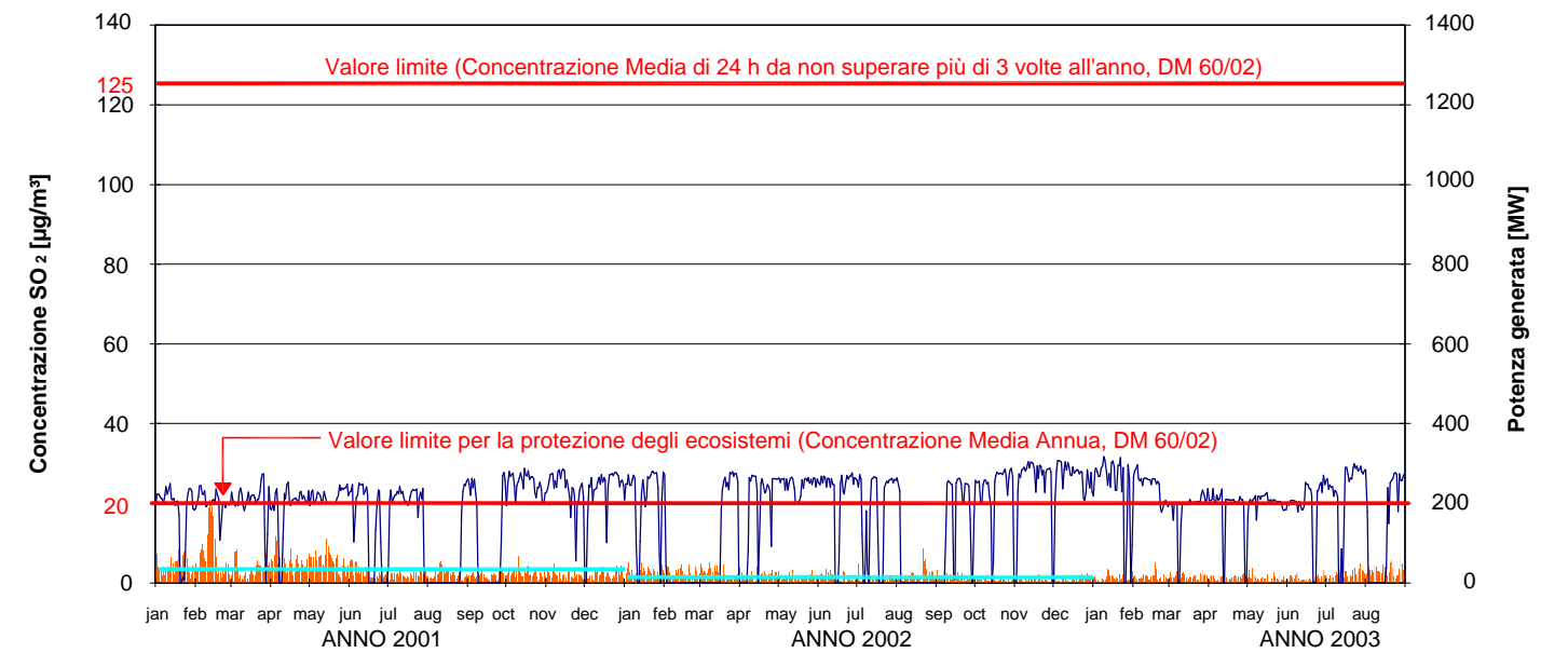
CONCENTRAZIONI MEDIE GIORNALIERE DI SO 2 Postazione No. 3 in località La Rosa
