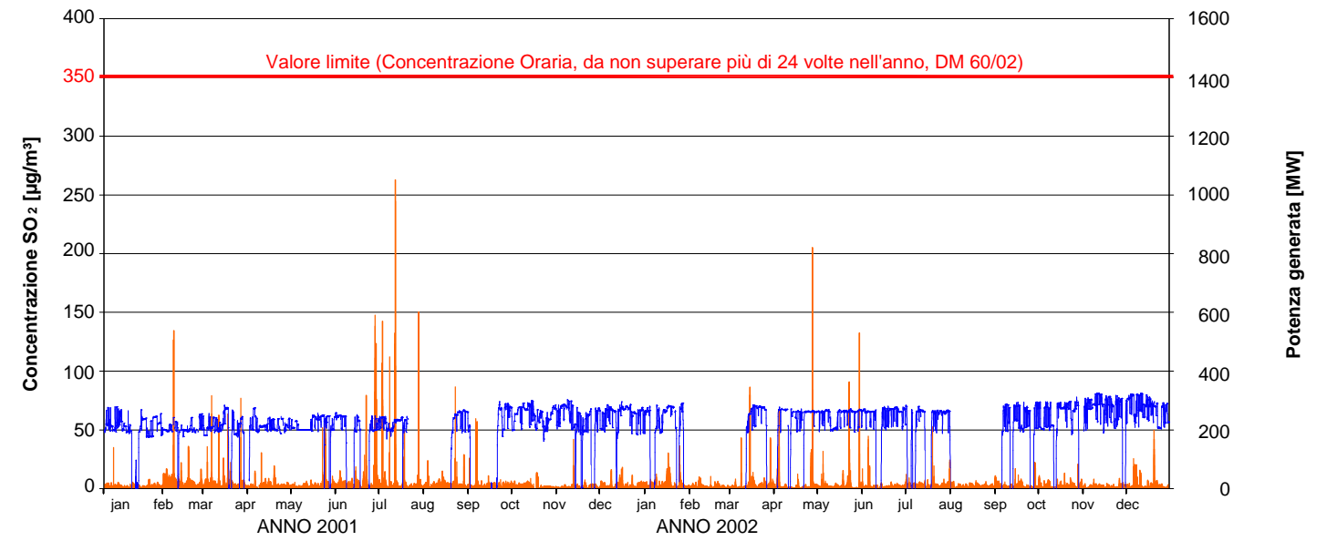
CONCENTRAZIONI ORARIE DI SO 2 Postazione No. 4 in località Centro
