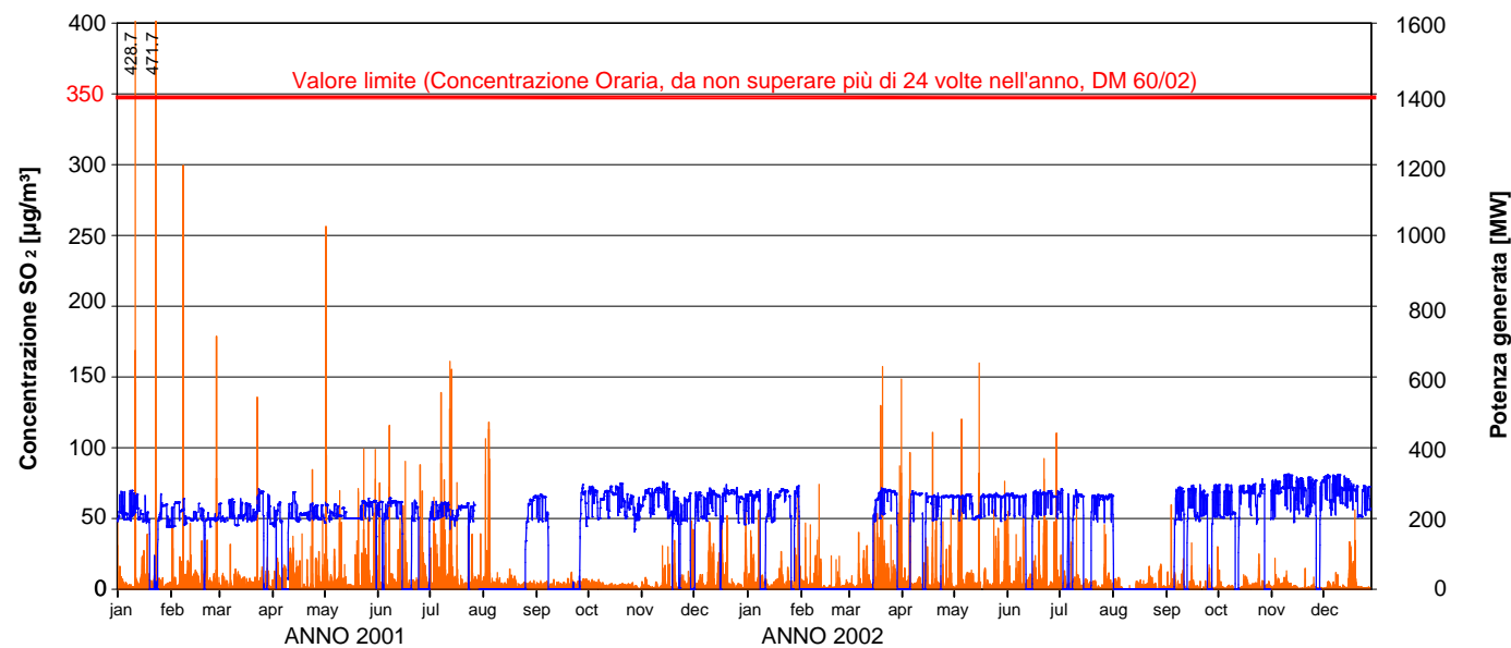
CONCENTRAZIONI ORARIE DI SO 2 Postazione No. 2 in località Tutturano
