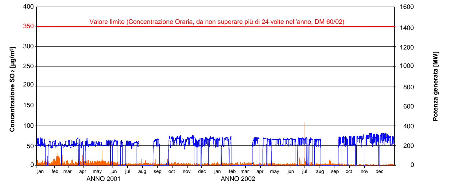
CONCENTRAZIONI ORARIE DI SO 2 Postazione No. 3 in località La Rosa
