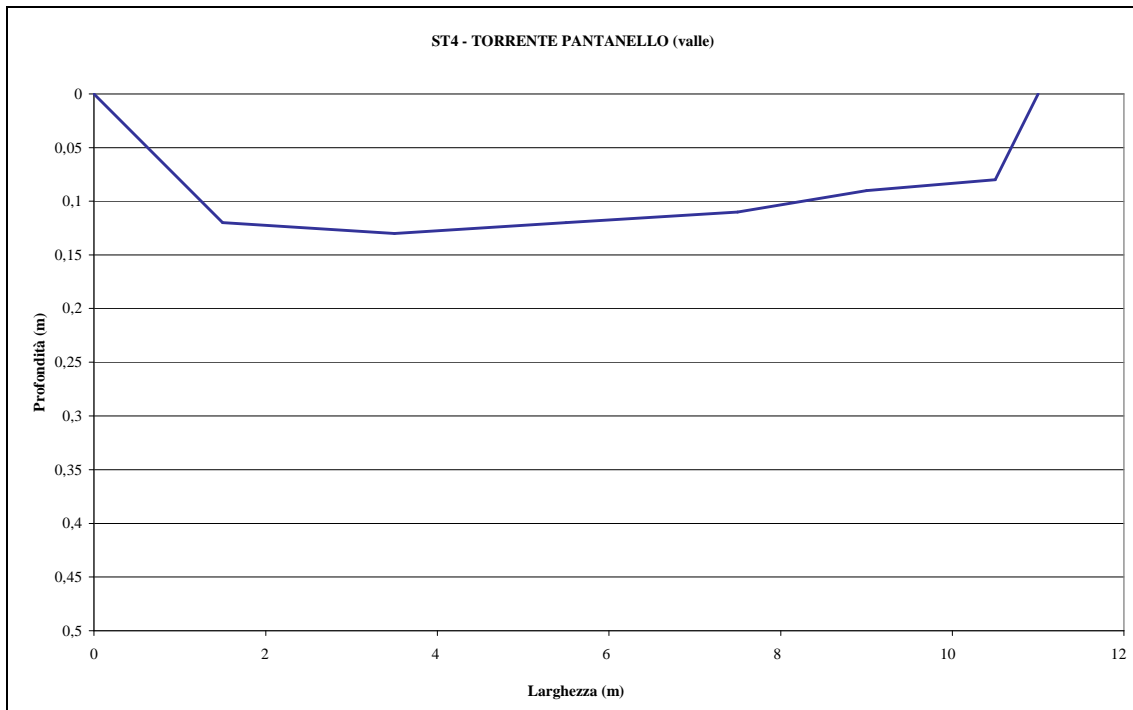
Figura 4.10 — Stazione ST_4 Torrente Pantanello – profilo della sezione di misura
