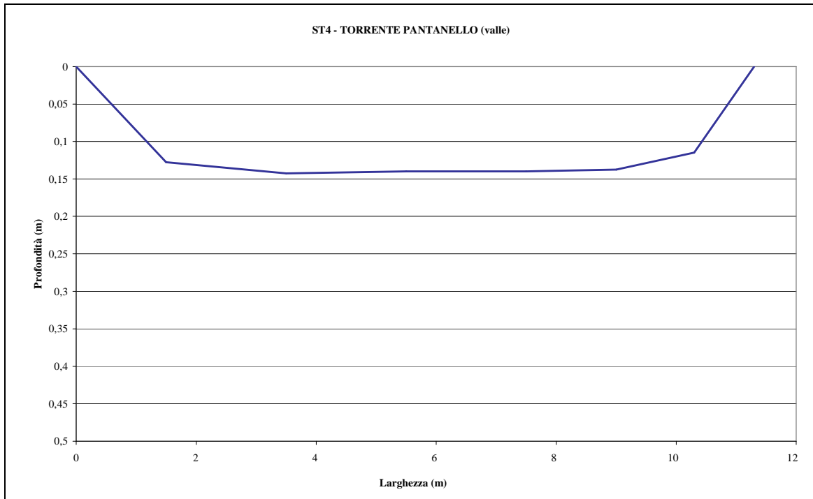
Figura 4.11 — Stazione ST_4 Torrente Pantanello – profilo della sezione di misura
