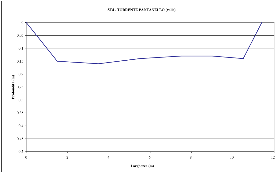
Figura 4.12 — Stazione ST_4 Torrente Pantanello – profilo della sezione di misura
