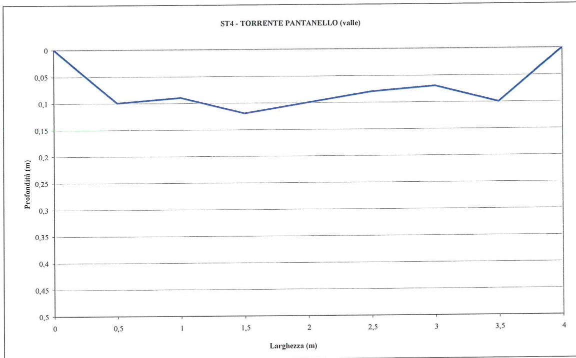
Figura 4.16 — Stazione ST_4 Torrente Pantanello – profilo della sezione di misura
