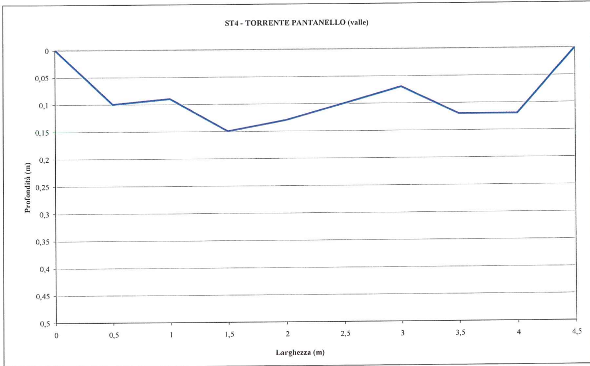
Figura 4.15 — Stazione ST_4 Torrente Pantanello – profilo della sezione di misura
