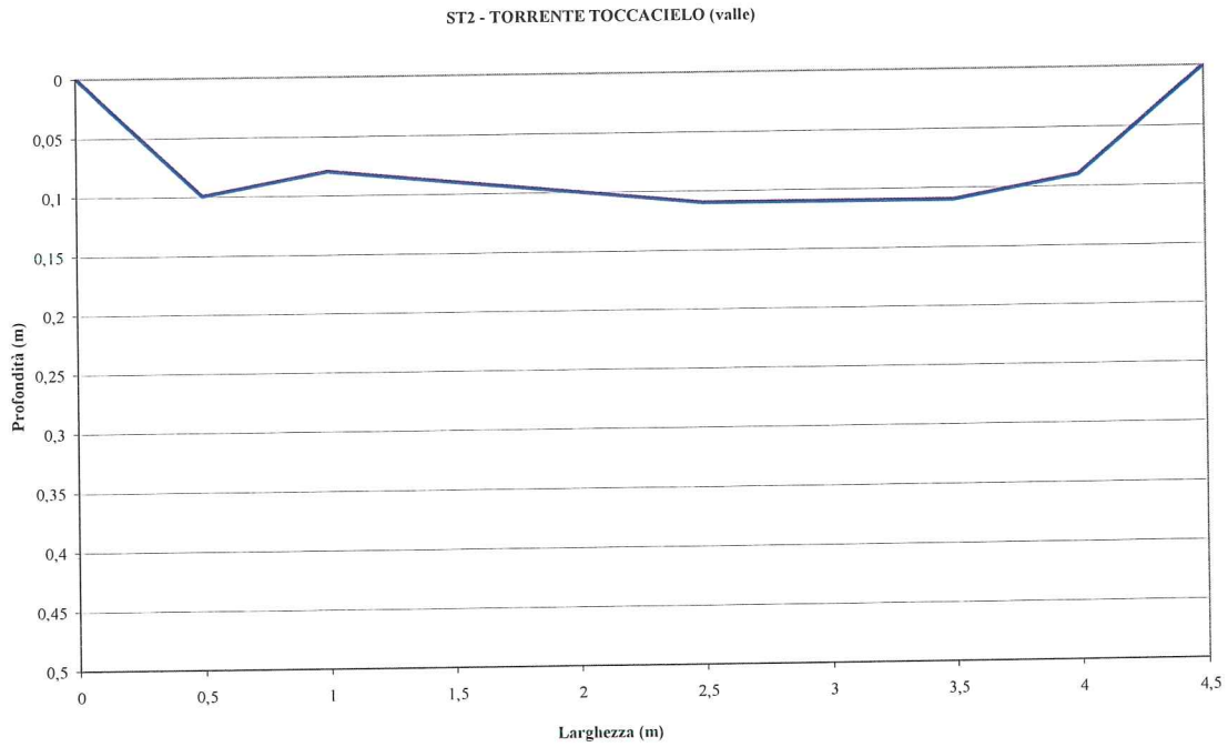
Figura 4.8 - Stazione ST_2 Torrente Toccacielo – profilo della sezione di misura
