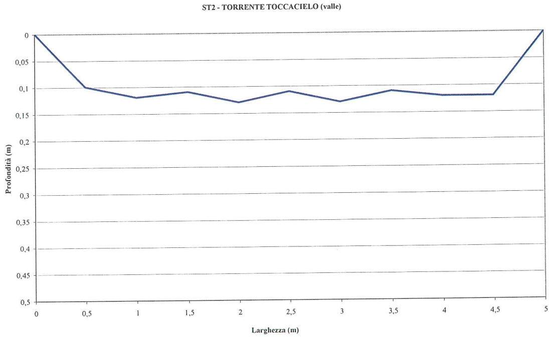
Figura 4.7 - Stazione ST_2 Torrente Toccacielo – profilo della sezione di misura
