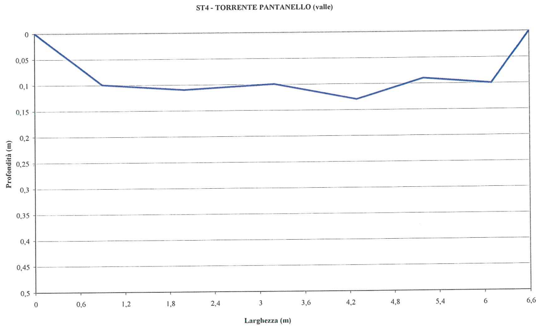
Figura 4.13 — Stazione ST_4 Torrente Pantanello – profilo della sezione di misura
