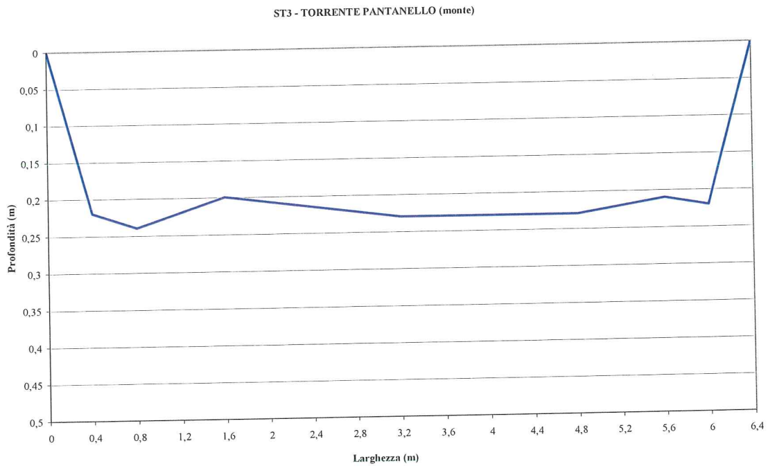
Figura 4.9 — Stazione ST_3 Torrente Pantanello – profilo della sezione di misura
