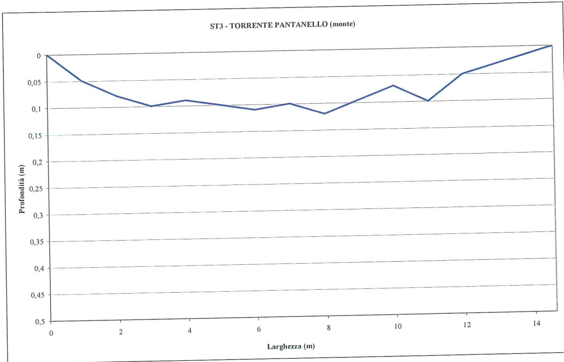
Figura 4.10 — Stazione ST_3 Torrente Pantanello – profilo della sezione di misura
