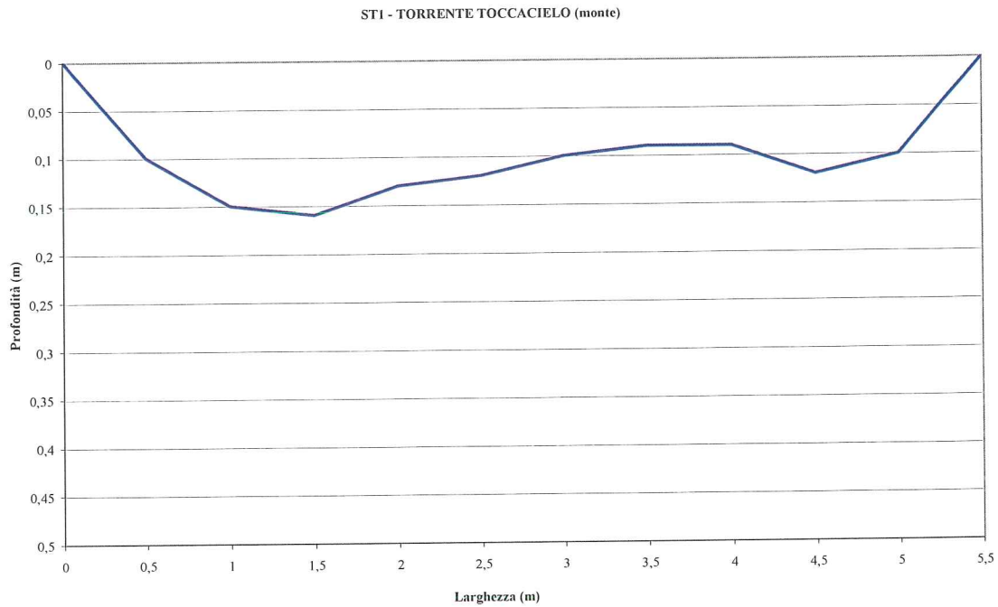
Figura 4.4 — Stazione ST_1 Torrente Toccacielo – profilo della sezione di misura
