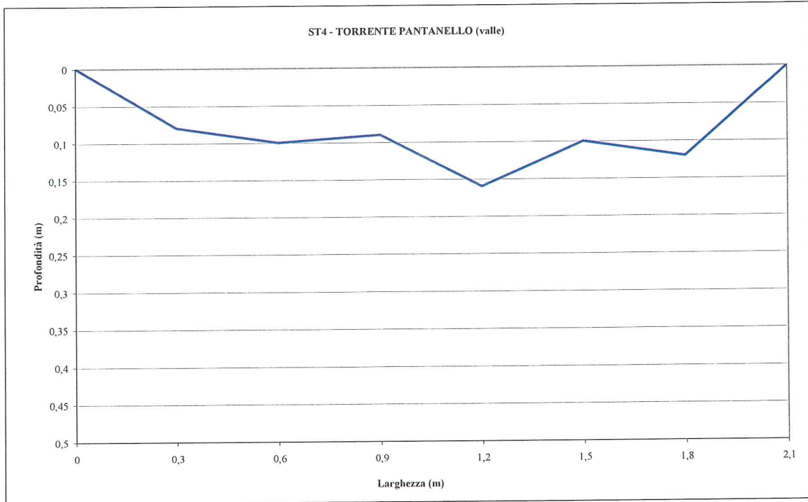
Figura 4.14 — Stazione ST_4 Torrente Pantanello – profilo della sezione di misura
