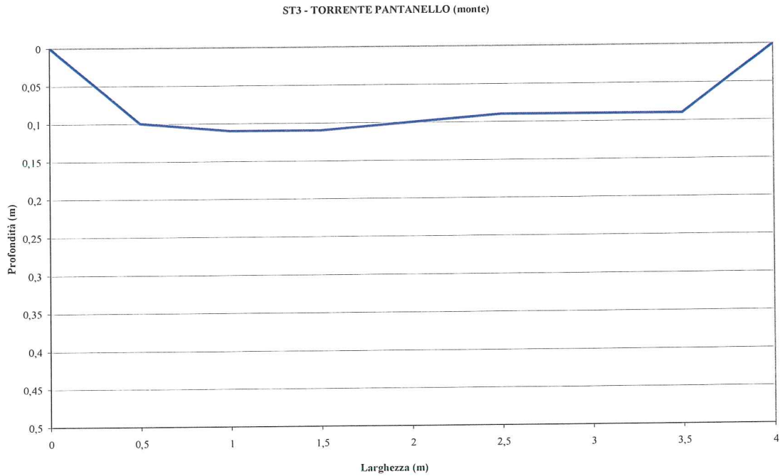
Figura 4.12 — Stazione ST_3 Torrente Pantanello – profilo della sezione di misura
