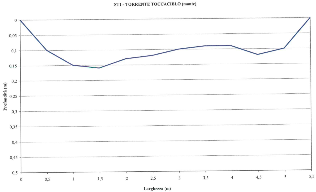
Figura 4.3 — Stazione ST_1 Torrente Toccacielo – profilo della sezione di misura
