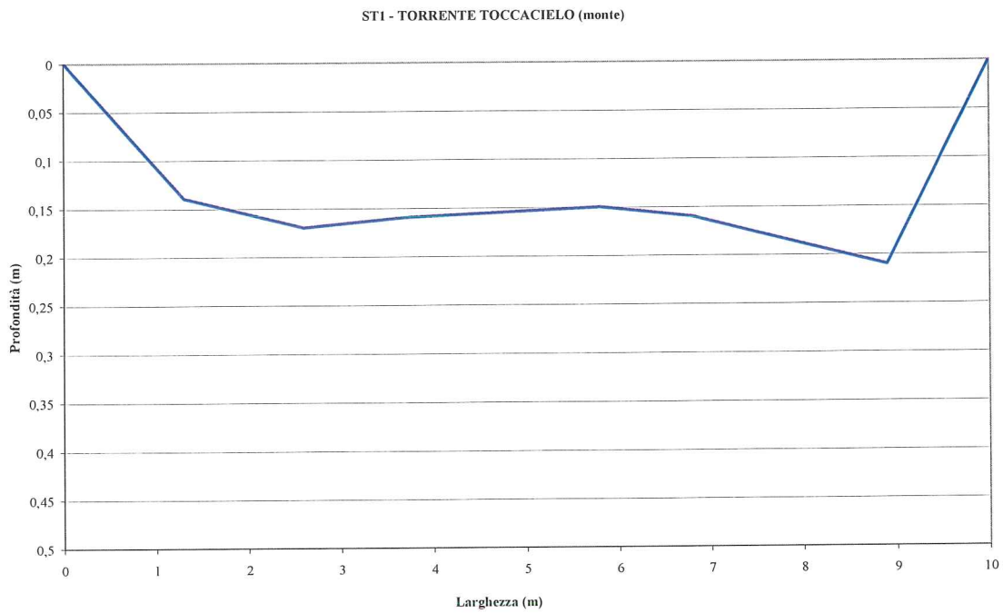
Figura 4.1 — Stazione ST_1 Torrente Toccacielo – profilo della sezione di misura
