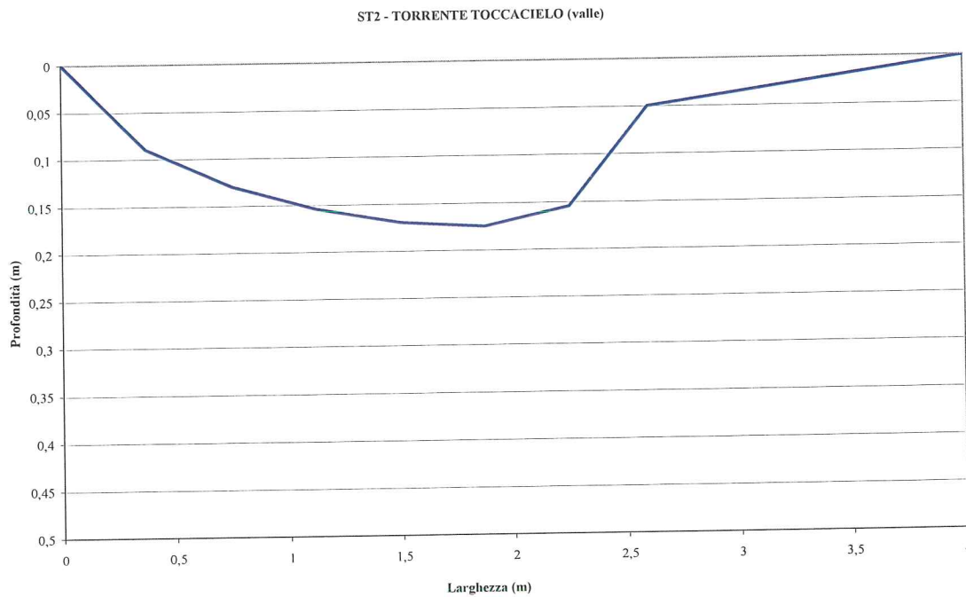
Figura 4.6 - Stazione ST_2 Torrente Toccacielo – profilo della sezione di misura
