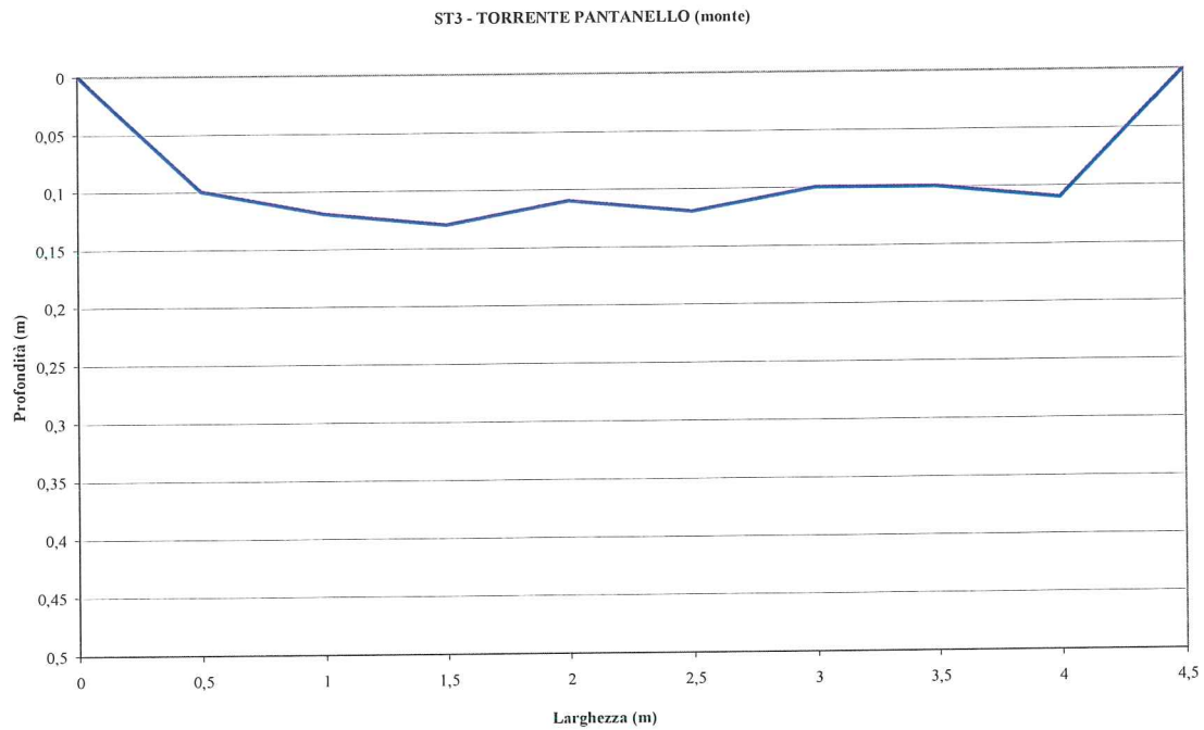
Figura 4.11 — Stazione ST_3 Torrente Pantanello – profilo della sezione di misura
