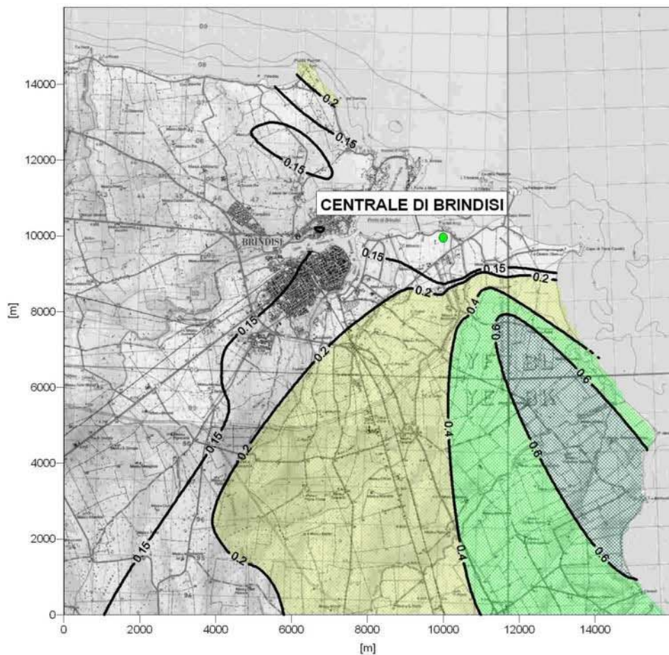
STATO ATTUALE (Gruppi No. 3 e No. 4: 400 mg/Nm 3 , 4000 ore/anno)
