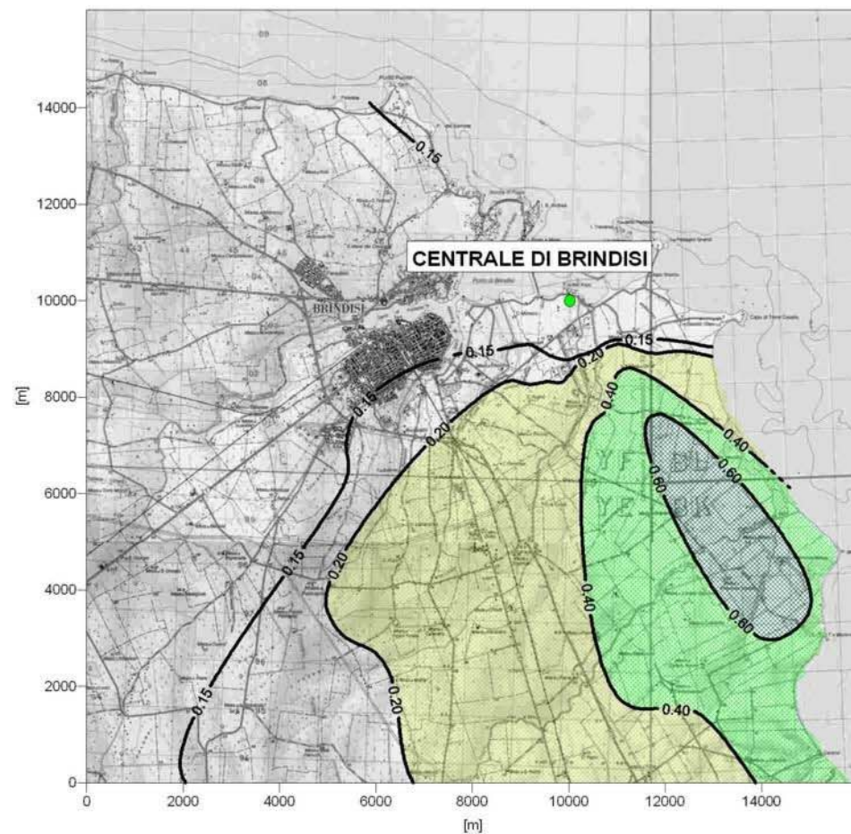
SCENARIO TEORICO CON LIMITI DI LEGGE (Gruppi No. 3 e No. 4: 200 mg/Nm 3 , 7200 ore/anno)
