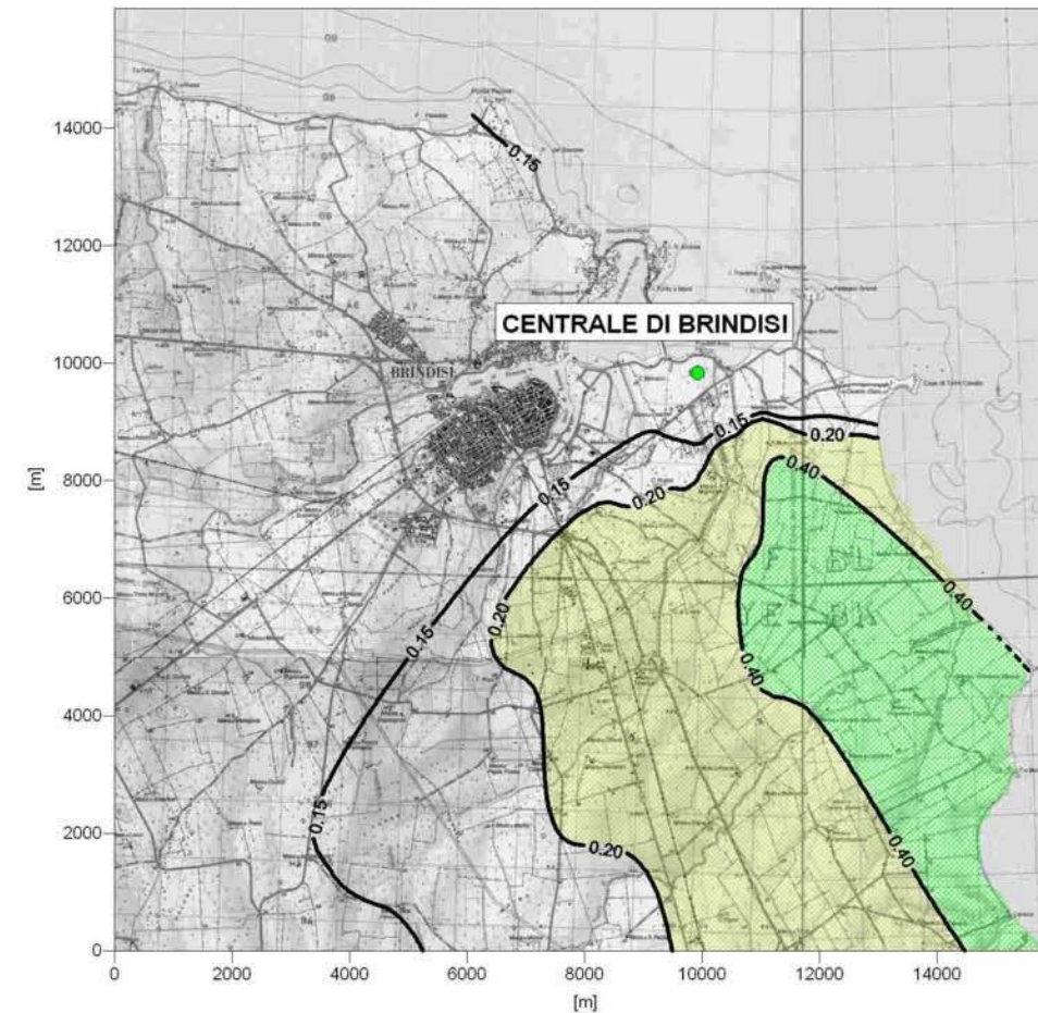
SCENARIO REALE DI ESERCIZIO (Gruppi No. 3 e No. 4: 200 mg/Nm 3 , 6300 ore/anno)
