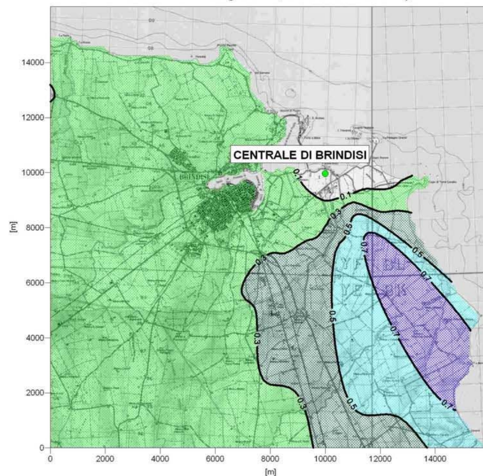
SCENARIO TEORICO CON I LIMITI DI LEGGE (Gruppi No. 3 e No. 4: 200 mg/Nm 3 , 7200 ore/anno CCGT: 50 mg/Nm 3 , 8000 ore/anno)
