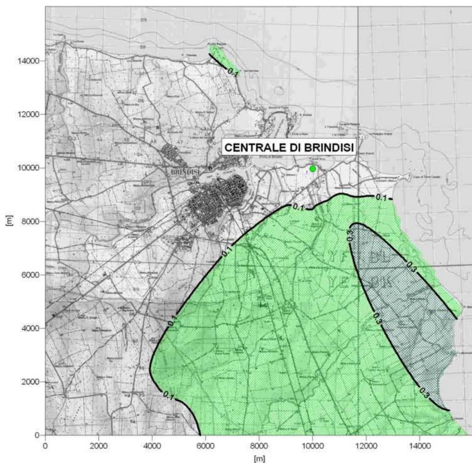
STATO ATTUALE (Gruppi No. 3 e No. 4: 200 mg/Nm 3 , 4000 ore/anno)
