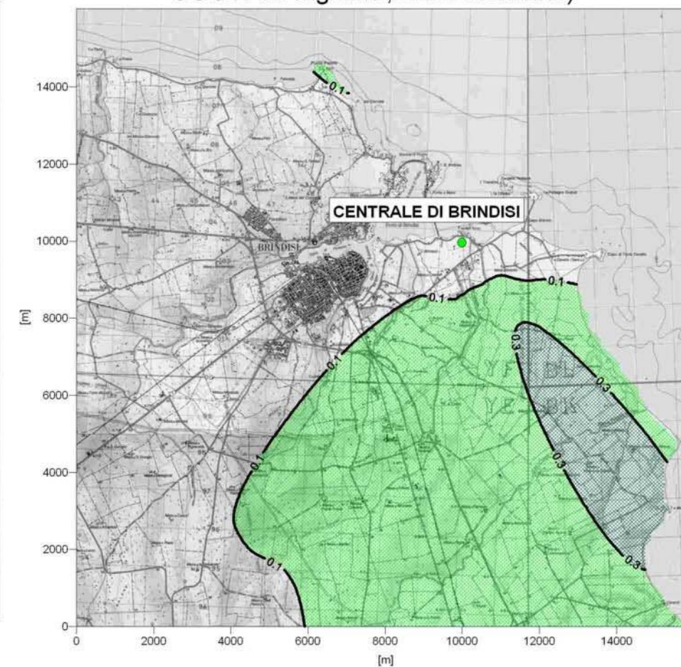
SCENARIO REALE DI ESERCIZIO (Gruppi No. 3 e No. 4: 100 mg/Nm 3 , 6300 ore/anno CCGT: 30 mg/Nm 3 , 5200 ore/anno)
