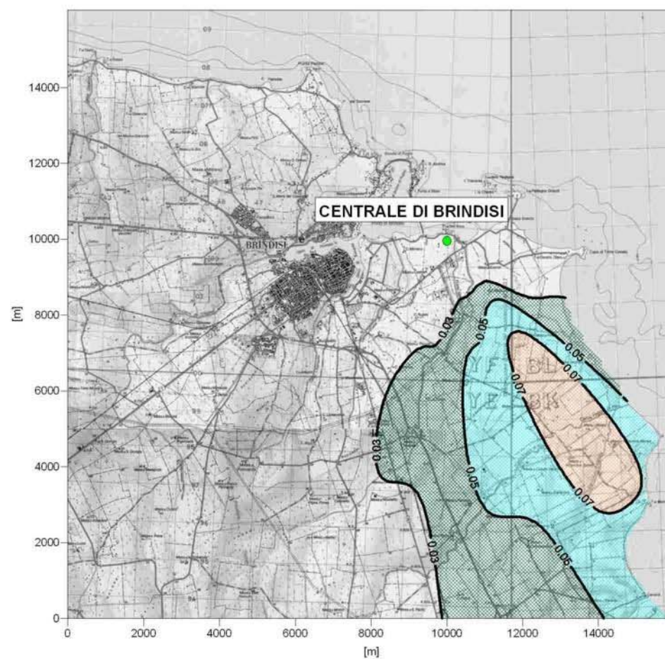
SCENARIO TEORICO CON I LIMITI DI LEGGE (Gruppi No. 3 e No. 4: 35 mg/Nm 3 , 7200 ore/anno)
