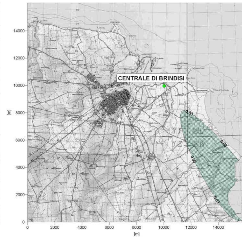
SCENARIO REALE DI ESERCIZIO (Gruppi No. 3 e No. 4: 20 mg/Nm 3 , 6300 ore/anno)
