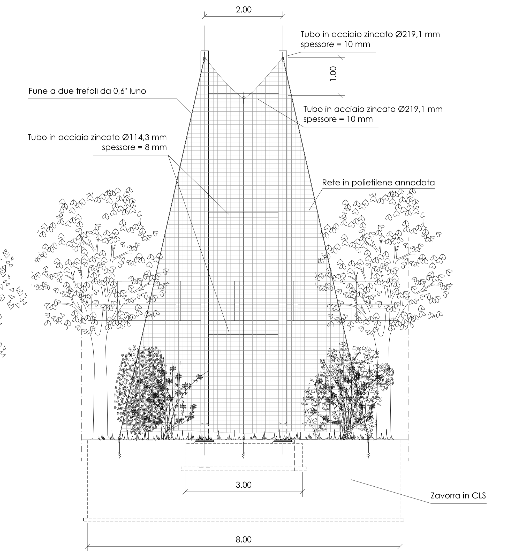
PROSPETTO B-B scala 1:50
