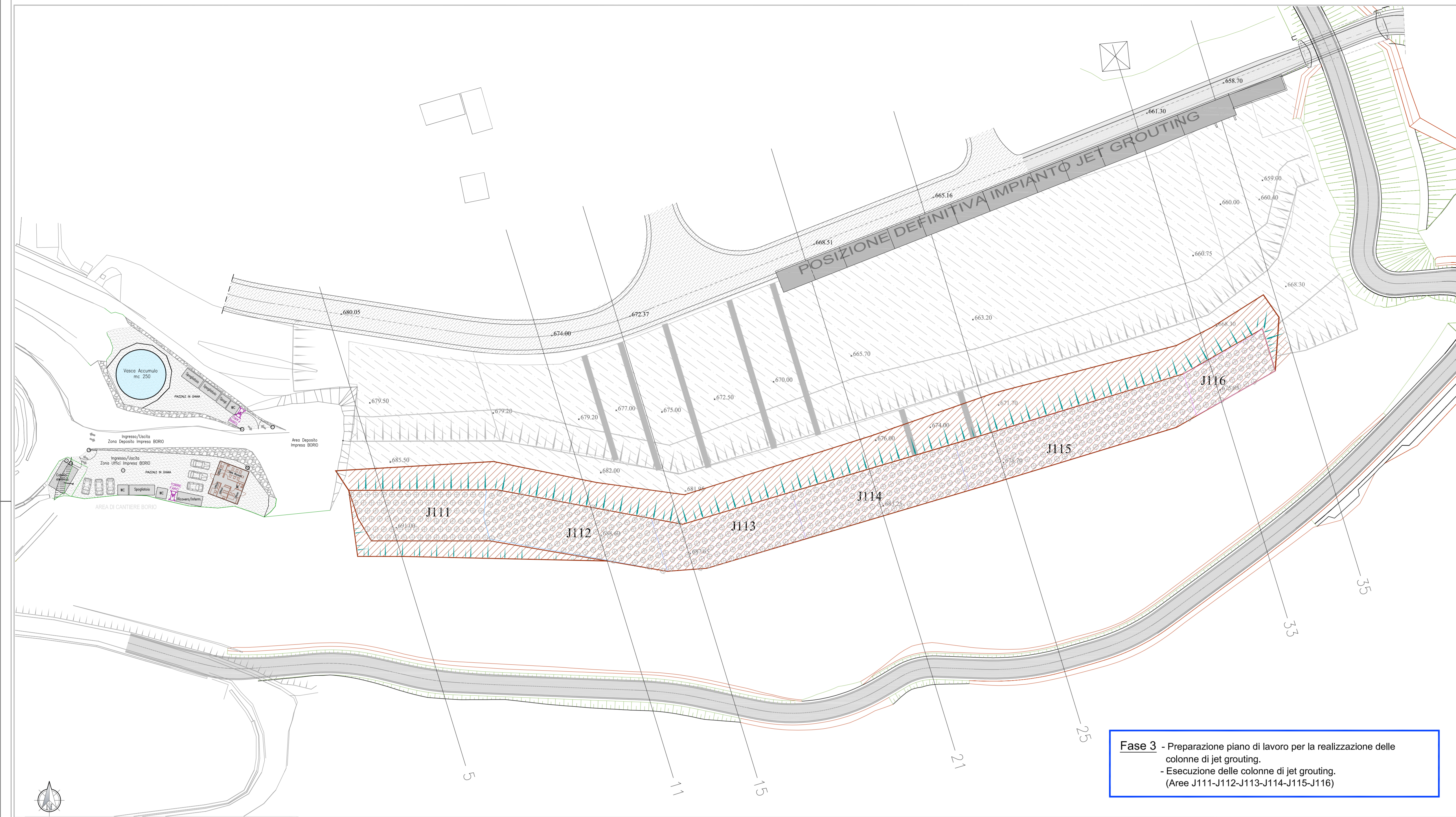
PLANIMETRIA JET (FASE 3) - scala 1:500
