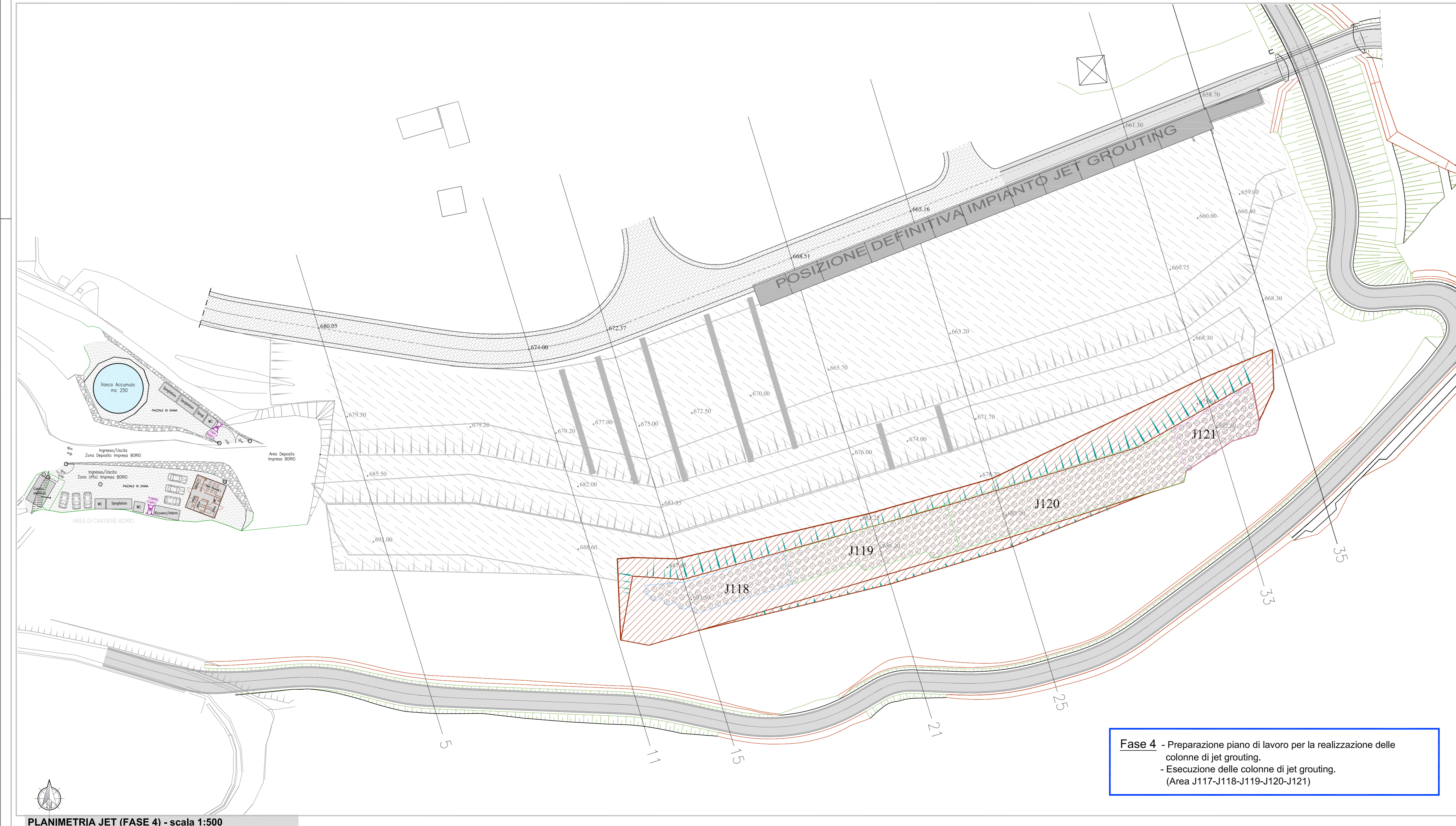
PLANIMETRIA JET (FASE 4) - scala 1:500
