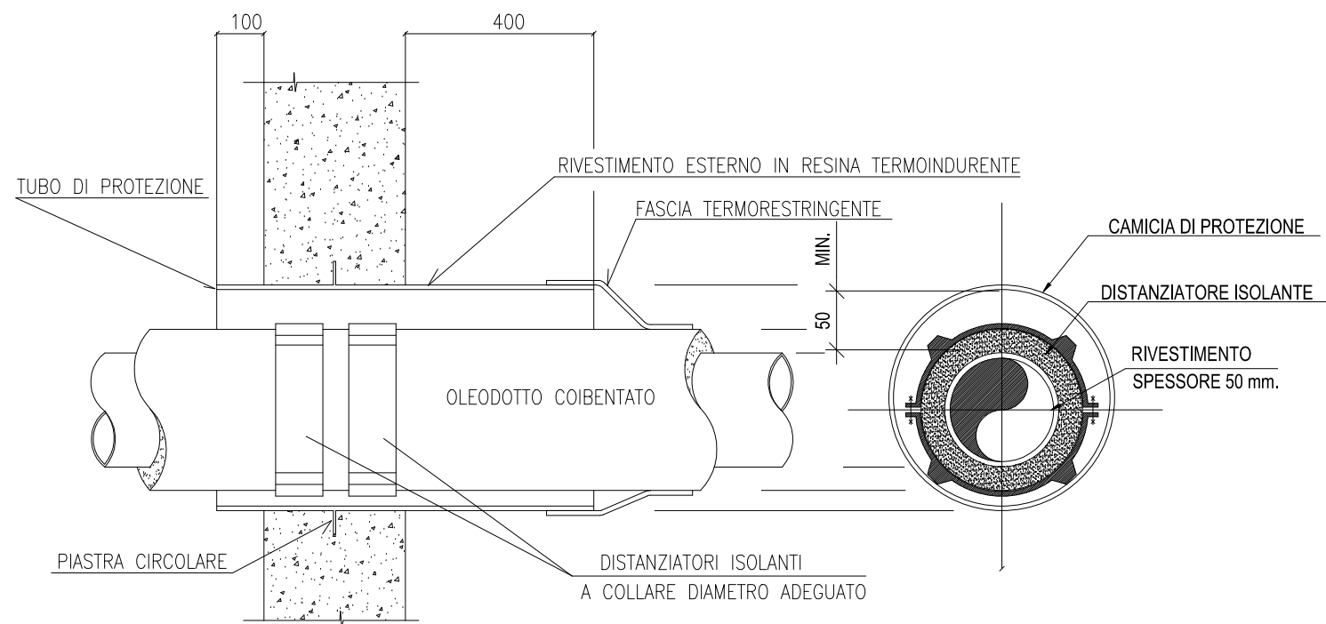
DETTAGLIO "A"
