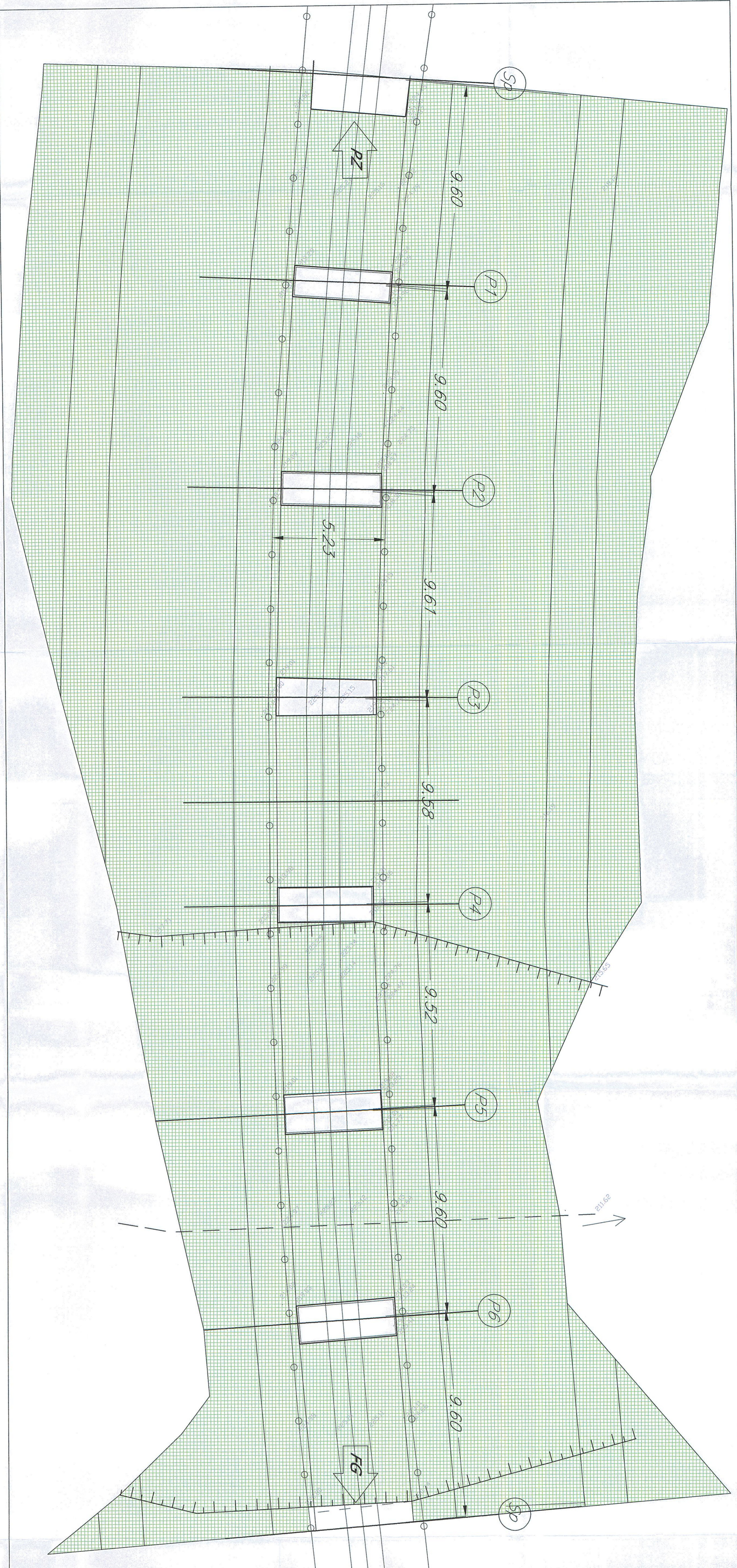
PLANIMETRIA BONIFICA ORDIGNI ESPLOSIONI SUPERFICIALE
