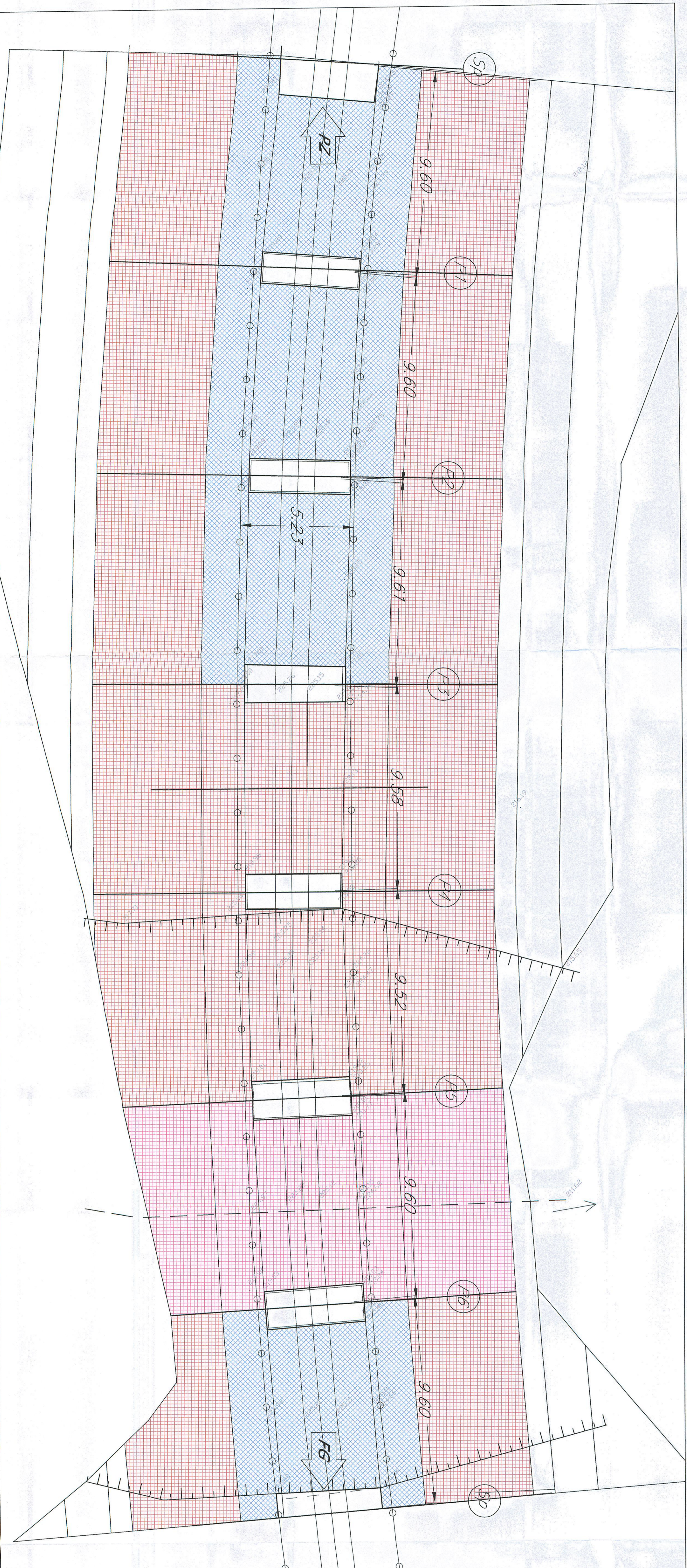
PLANIMETRIA BONIFICA ORDIGNI ESPLOSIONI PROFONDA A 5m, A 5m E A 7m
