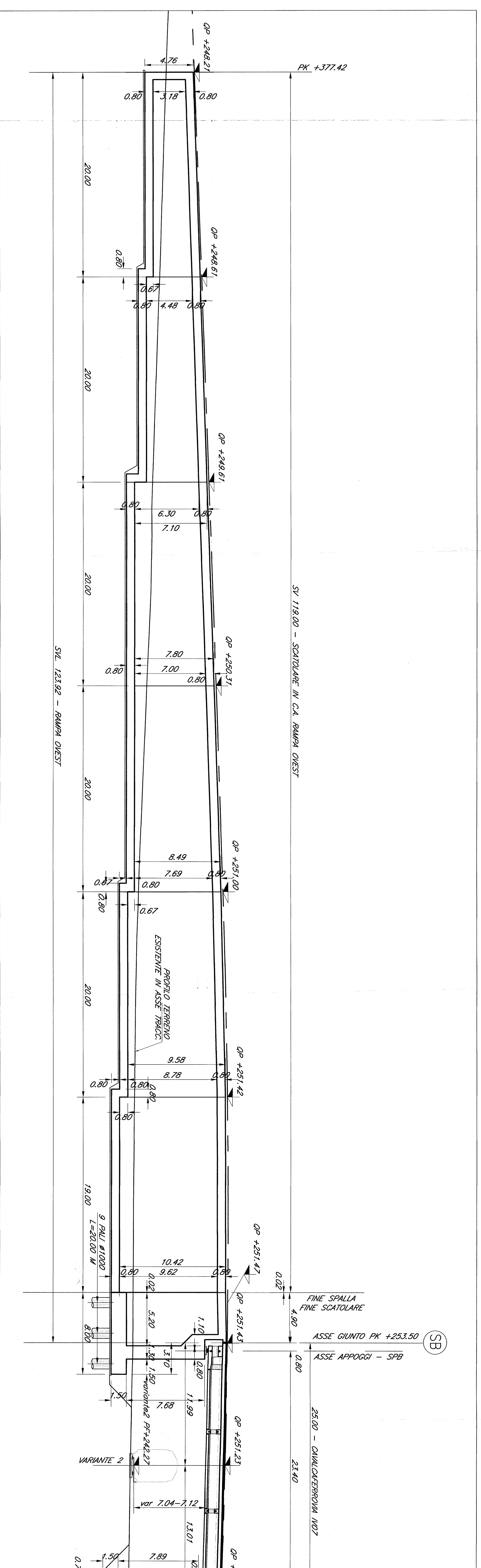
SEZIONE LONGITUDINALE (in asse) Scala 1:200
