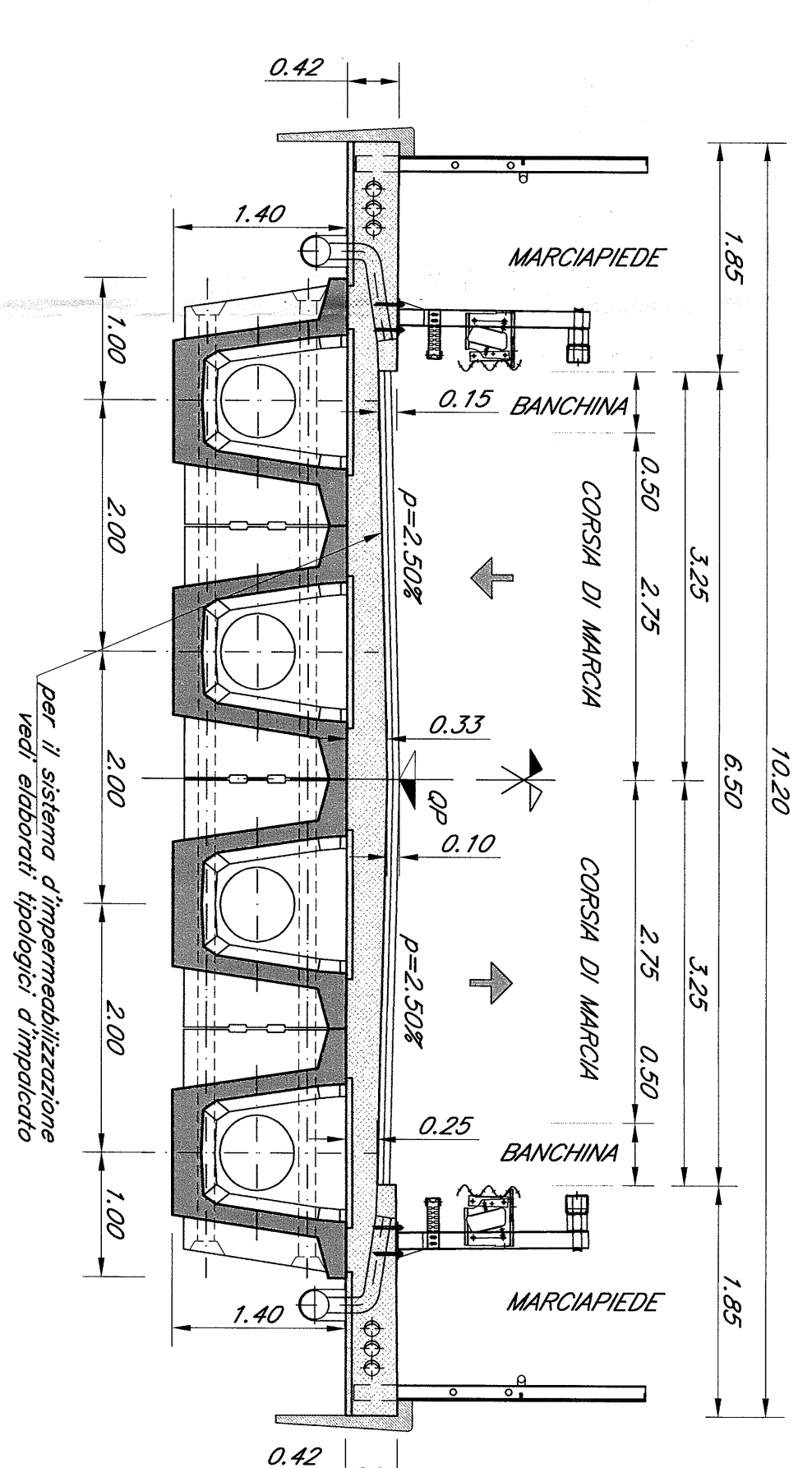
SEZIONE TRASVERSALE IMPALCATO Scala 1:50
