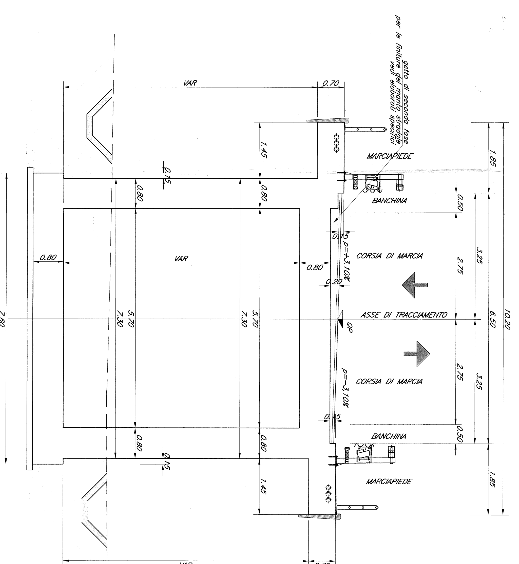
SEZIONE TRASVERSALE IMPALCATO Scala 1:50
