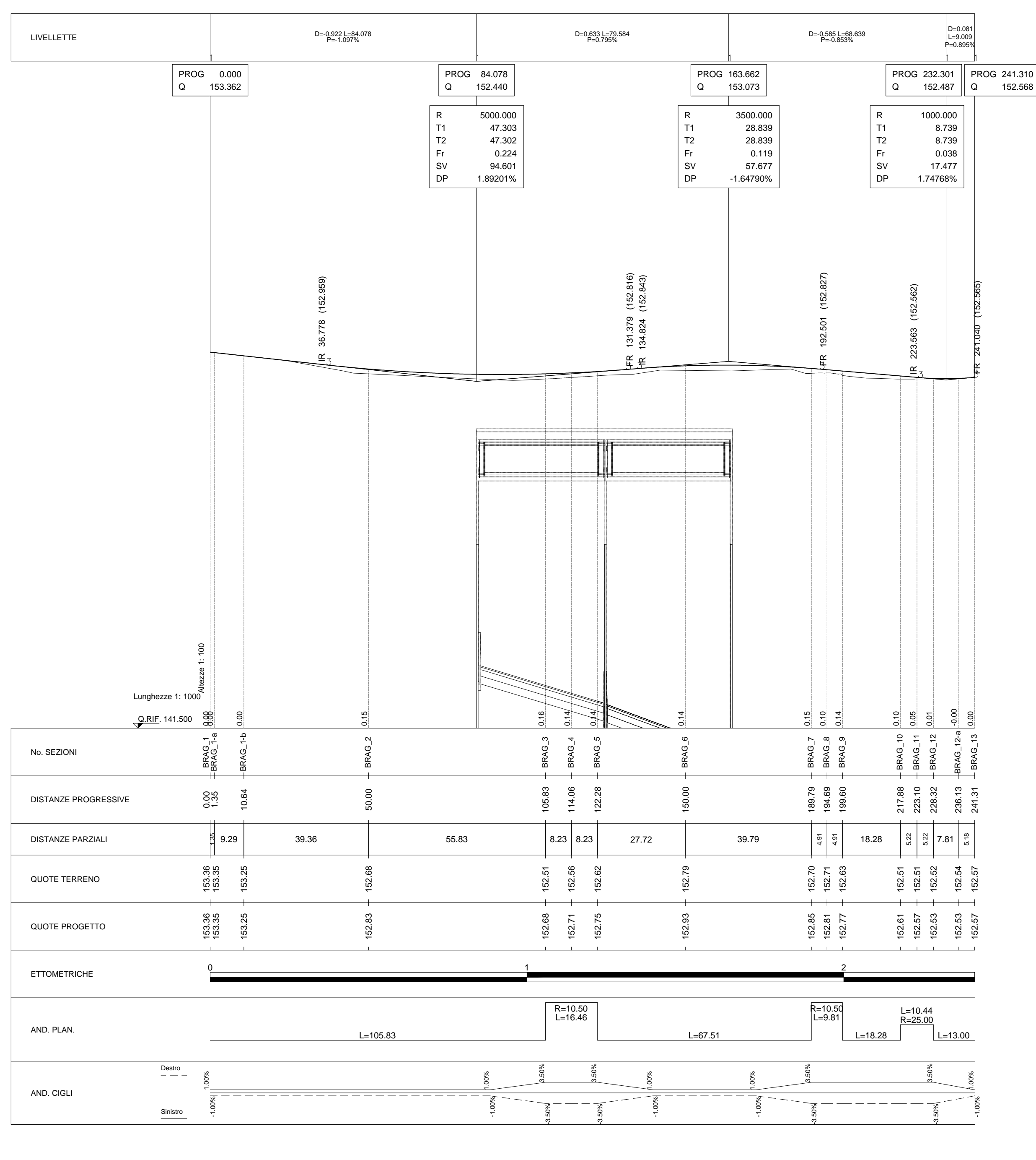
PROFILO LONGITUDINALE — Scala 1:1000/100
