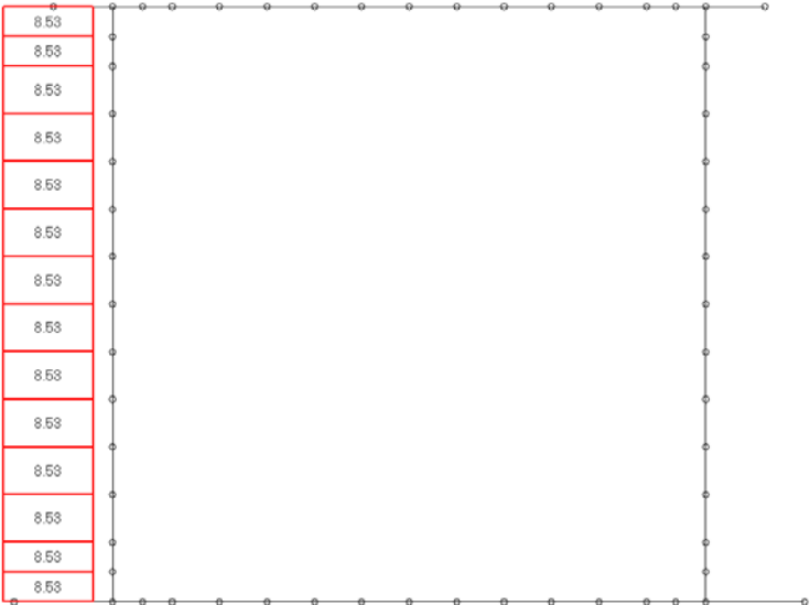
Loading di carico 16 : sovraspinta per q = 20 \text{ kN/mq} a sx - k = k_0
