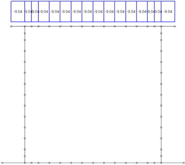
Loading di carico 2 : peso ricoprimento
