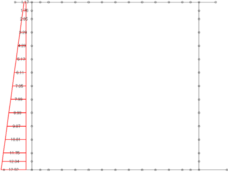
Loading di carico 36 : spinta falda esterna da sx - k = ka
