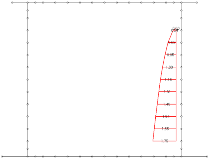
Loading di carico 39 : spinta idrodinamica in sisma
