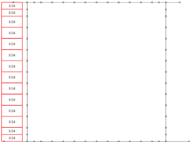
Loading di carico 30 : sisma orizzontale da sx - sovraspinta terre
