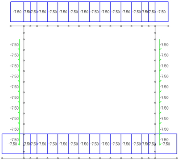
Loading di carico 1 : peso proprio
