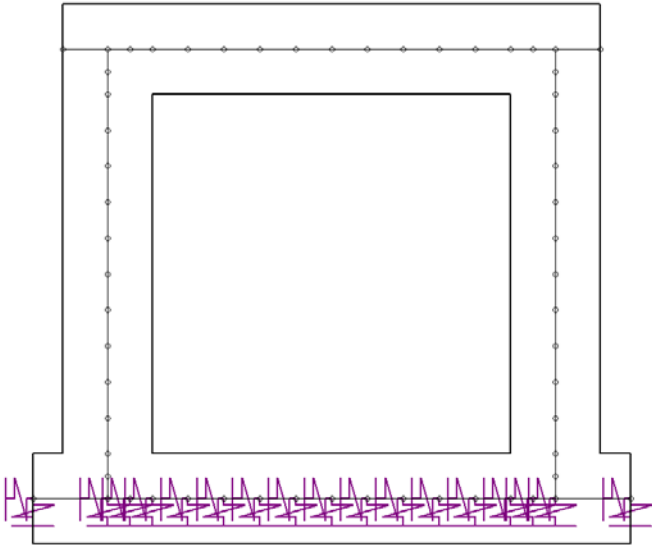
Immagine 4: molle elastiche simulanti il terreno
