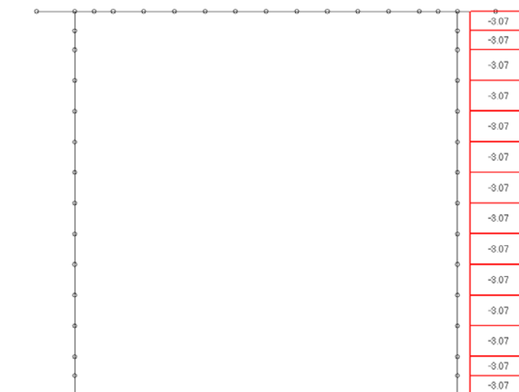
Loading di carico 21 : sovraspinta per q = 7.2 \text{ kN/mq} a dx - k = k0
