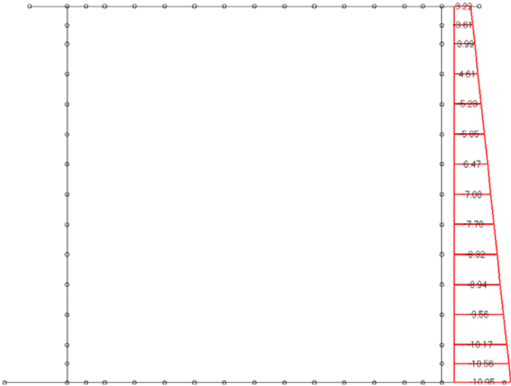
Loading di carico 6 : spinta terre su piedritto dx - k = k_a
