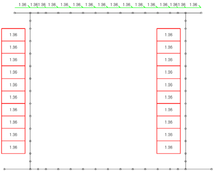
Loading di carico 28 : sisma orizzontale da sx - masse strutturali
