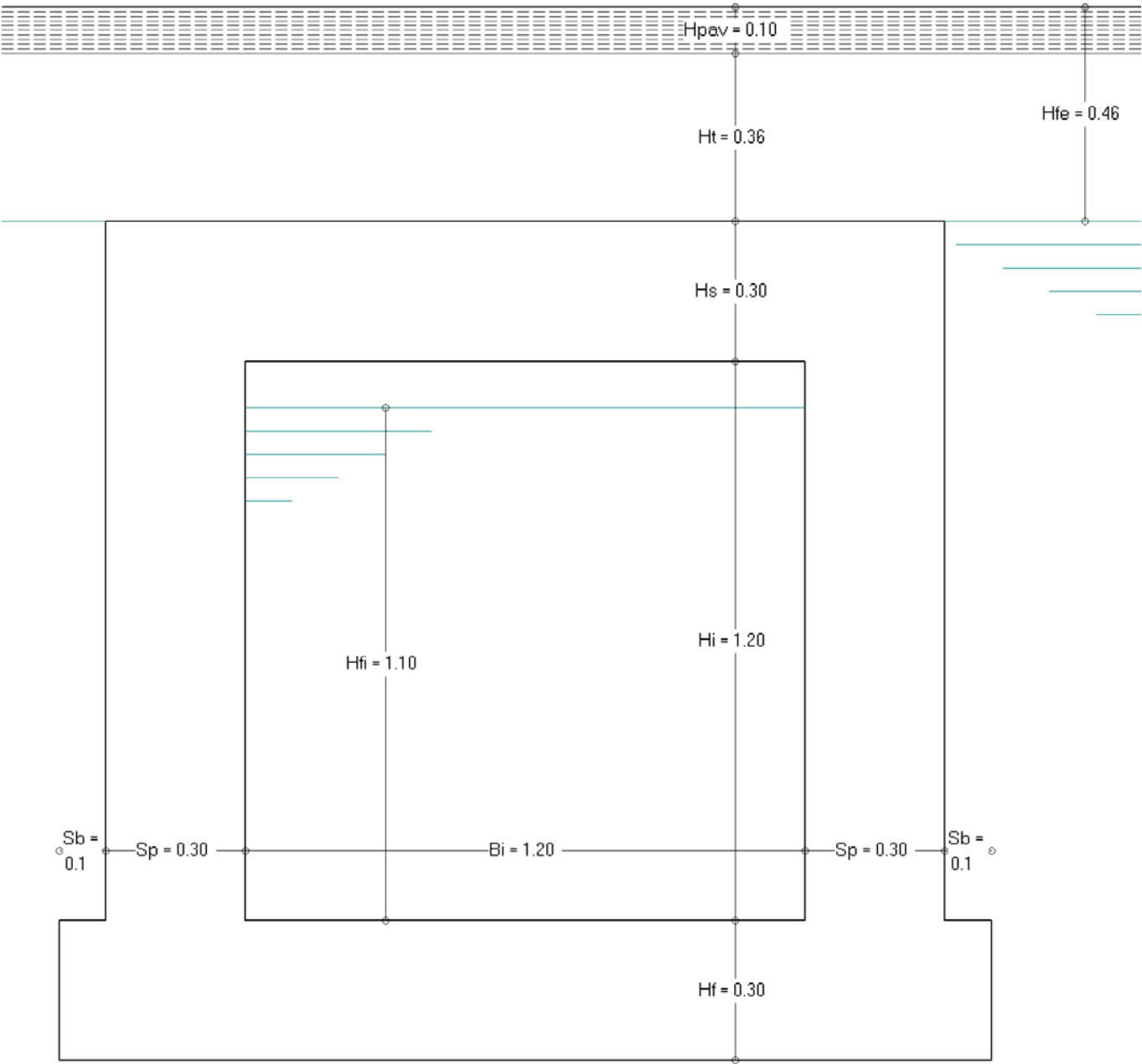
Immagine 1: geometria del tombino
