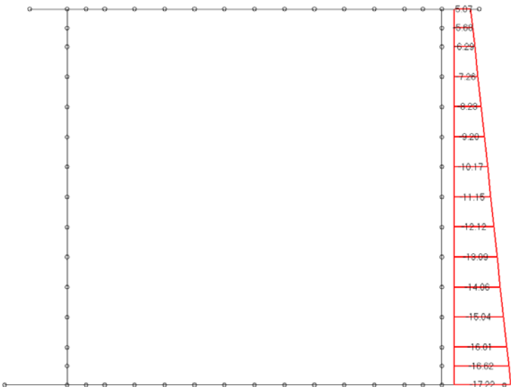
Loading di carico 4 : spinta terre su piedritto dx - k = k_0
