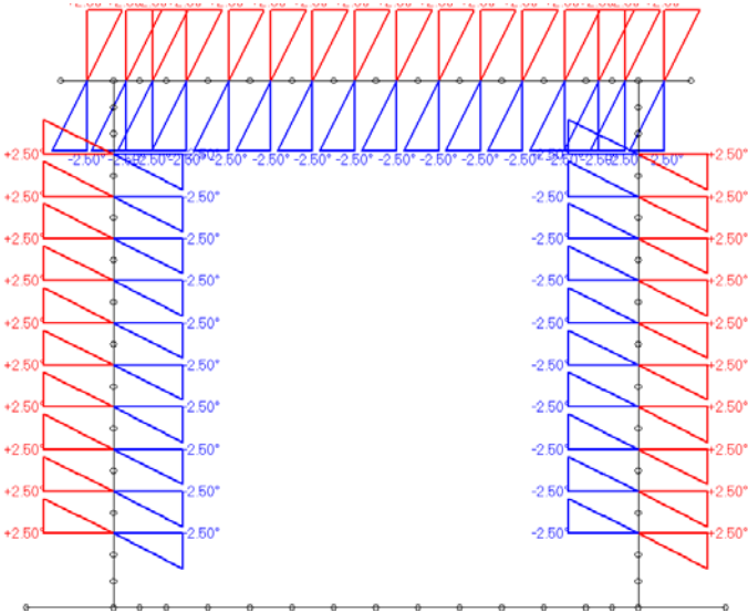
Loading di carico 27 : salto termico
