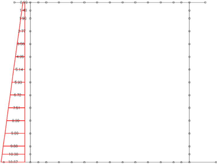
Loading di carico 34 : spinta falda esterna da sx - k = k0
