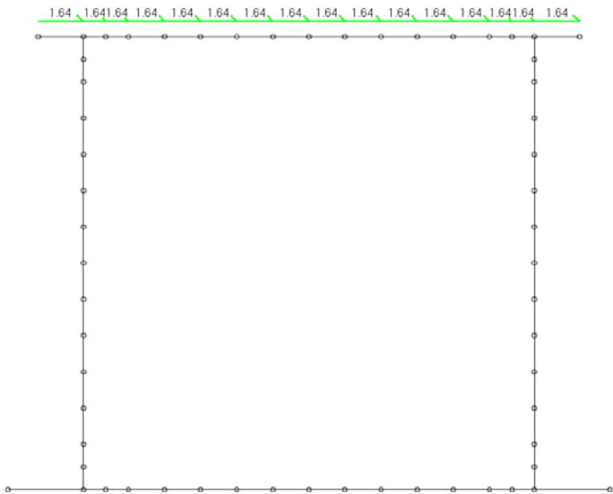
Loading di carico 29 : sisma orizzontale da sx - ricoprimento
