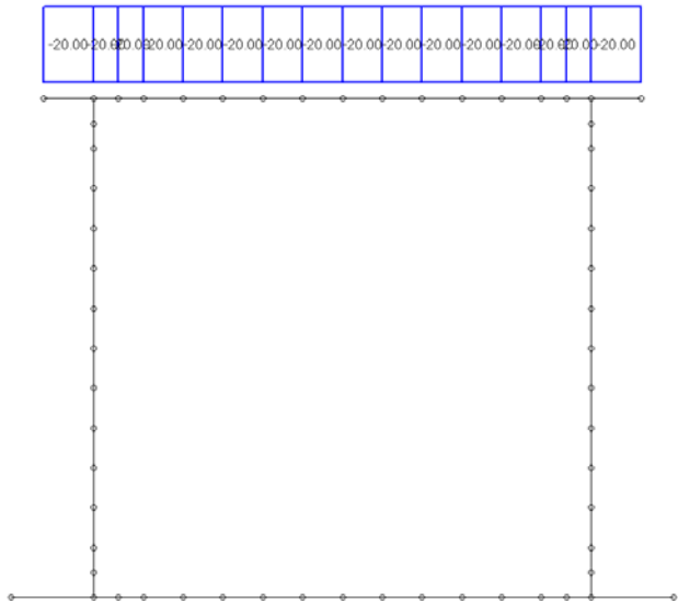
Loading di carico 11 : carico verticale 20 kN/mq
