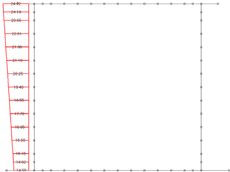
Loading di carico 12 : sovraspinta veicolari - tandem a sx - k = k0
