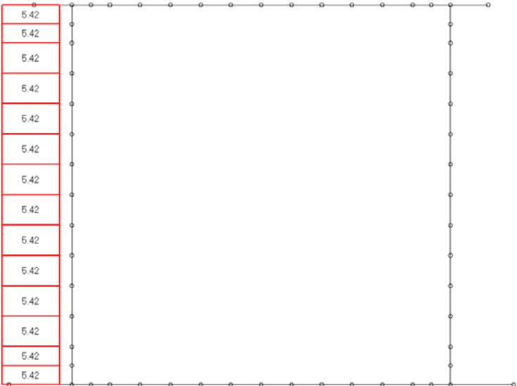
Loading di carico 18 : sovraspinta per q = 20 \text{ kN/mq} a sx - k = k_a
