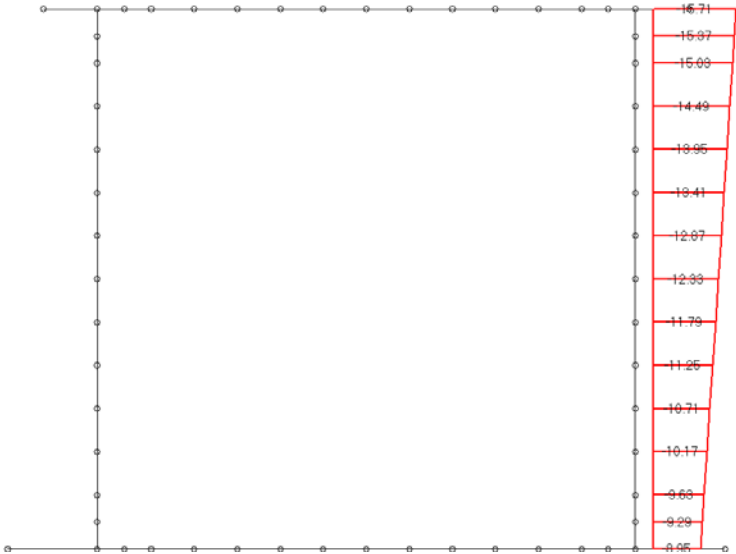
Loading di carico 15 : sovraspinta veicolari - tandem a dx - k = k_a
