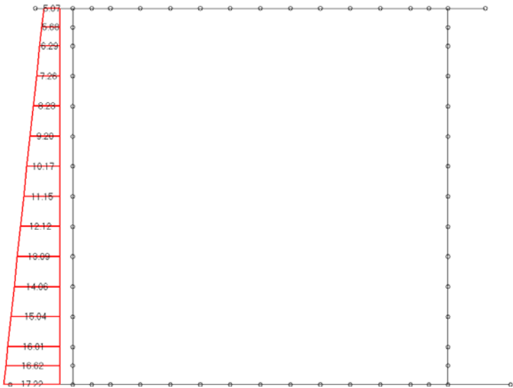
Loading di carico 3 : spinta terre su piedritto sx - k = k0
