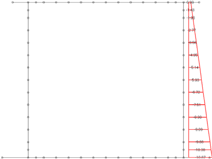
Loading di carico 35 : spinta falda esterna da dx - k = k0
