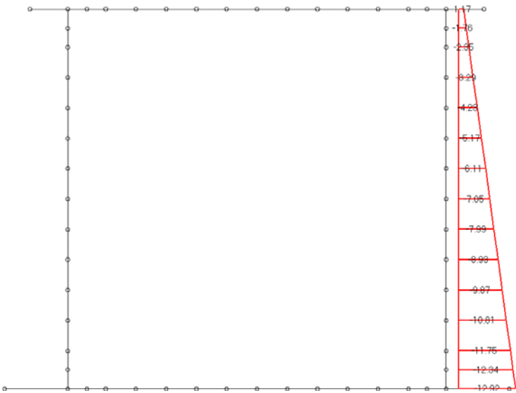
Loading di carico 37 : spinta falda esterna da dx - k = ka
