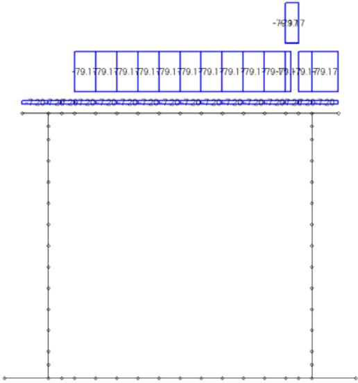
Loading di carico 8 : veicolari per max. taglio soletta (lato sx)
