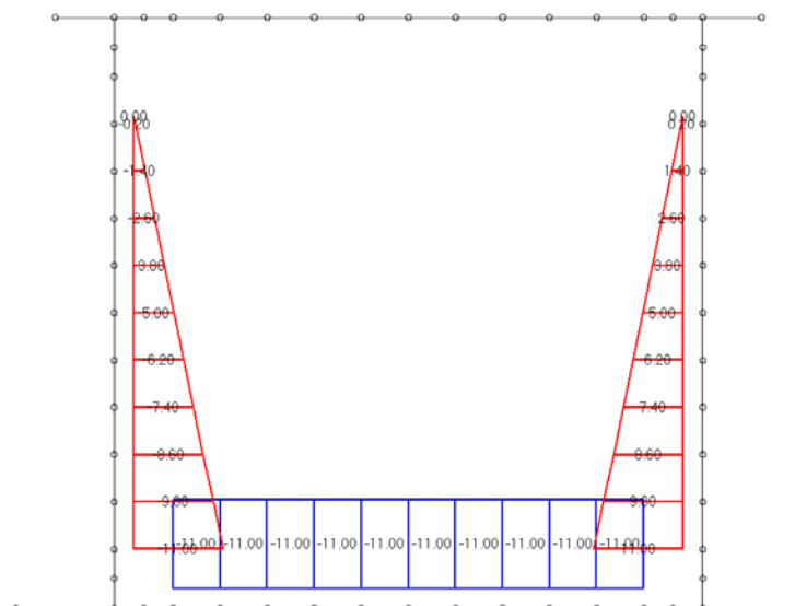
Loading di carico 33 : spinta idrostatica acque interne al tombino
