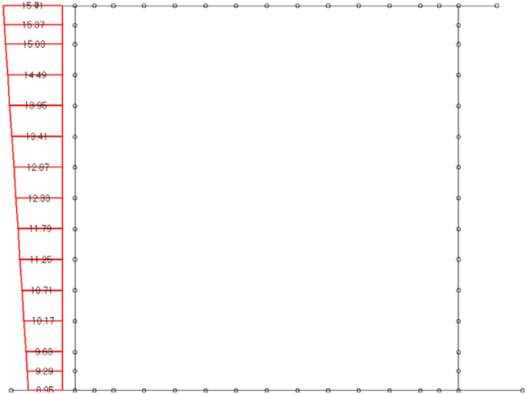
Loading di carico 14 : sovraspinta veicolari - tandem a sx - k = k_a
