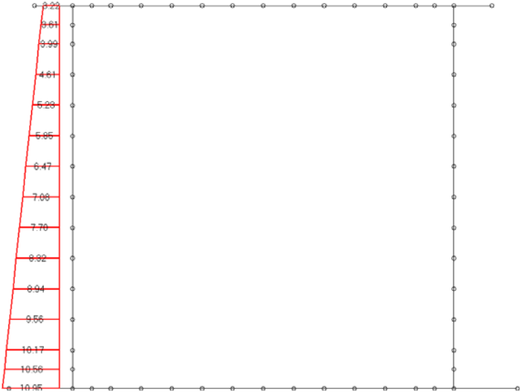
Loading di carico 5 : spinta terre su piedritto sx - k = k_a
