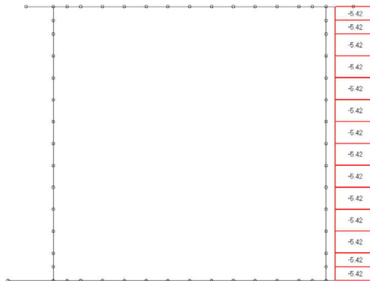
Loading di carico 19 : sovraspinta per q = 20 \text{ kN/mq} a dx - k = k_a
