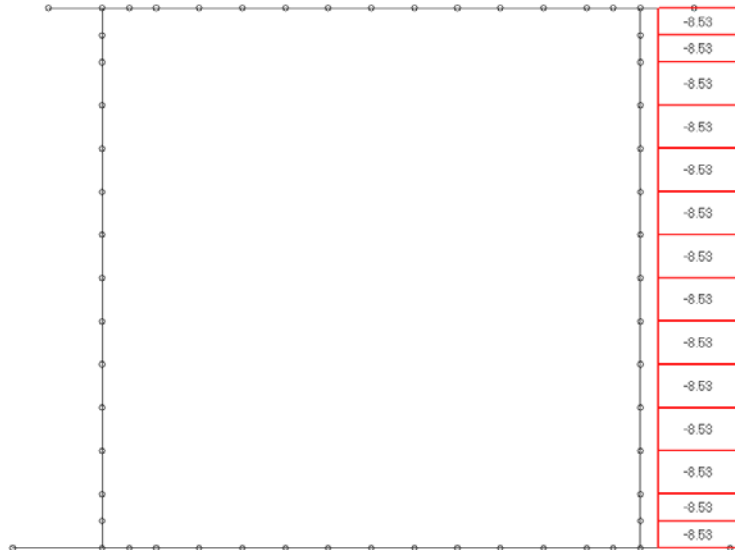
Loading di carico 17 : sovraspinta per q = 20 \text{ kN/mq} a dx - k = k_0
