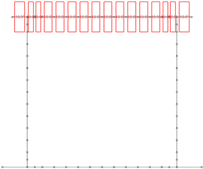
Loading di carico 25 : riscaldamento soletta superiore
