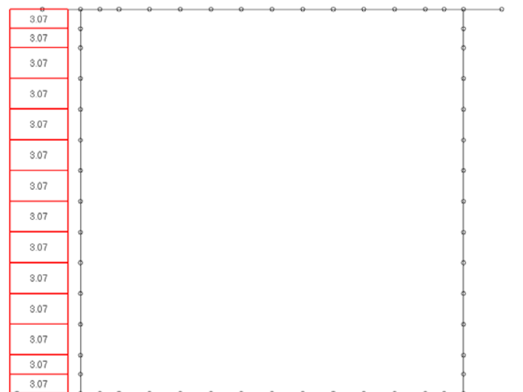
Loading di carico 20 : sovraspinta per q = 7.2 \text{ kN/mq} a sx - k = k_0
