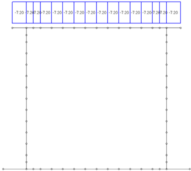
Loading di carico 10 : solo carico verticale qik (no tandem)
