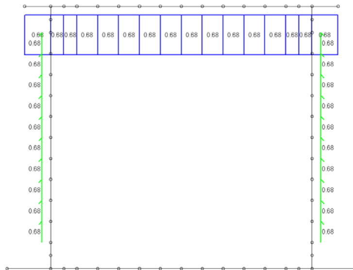
Loading di carico 31 : sisma verticale - masse strutturali
