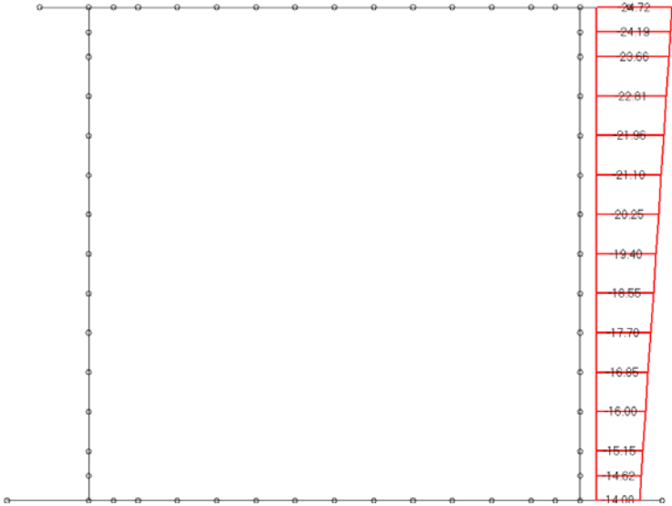
Loading di carico 13 : sovraspinta veicolari - tandem a dx - k = k_0
