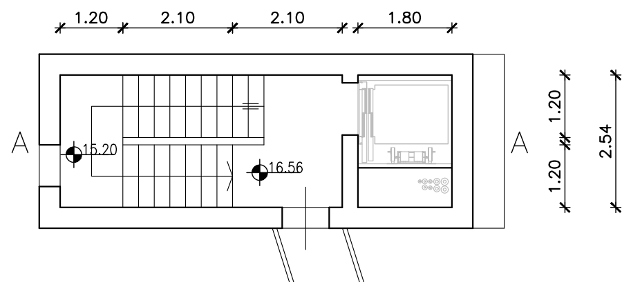
PIANTA COPERTURA
