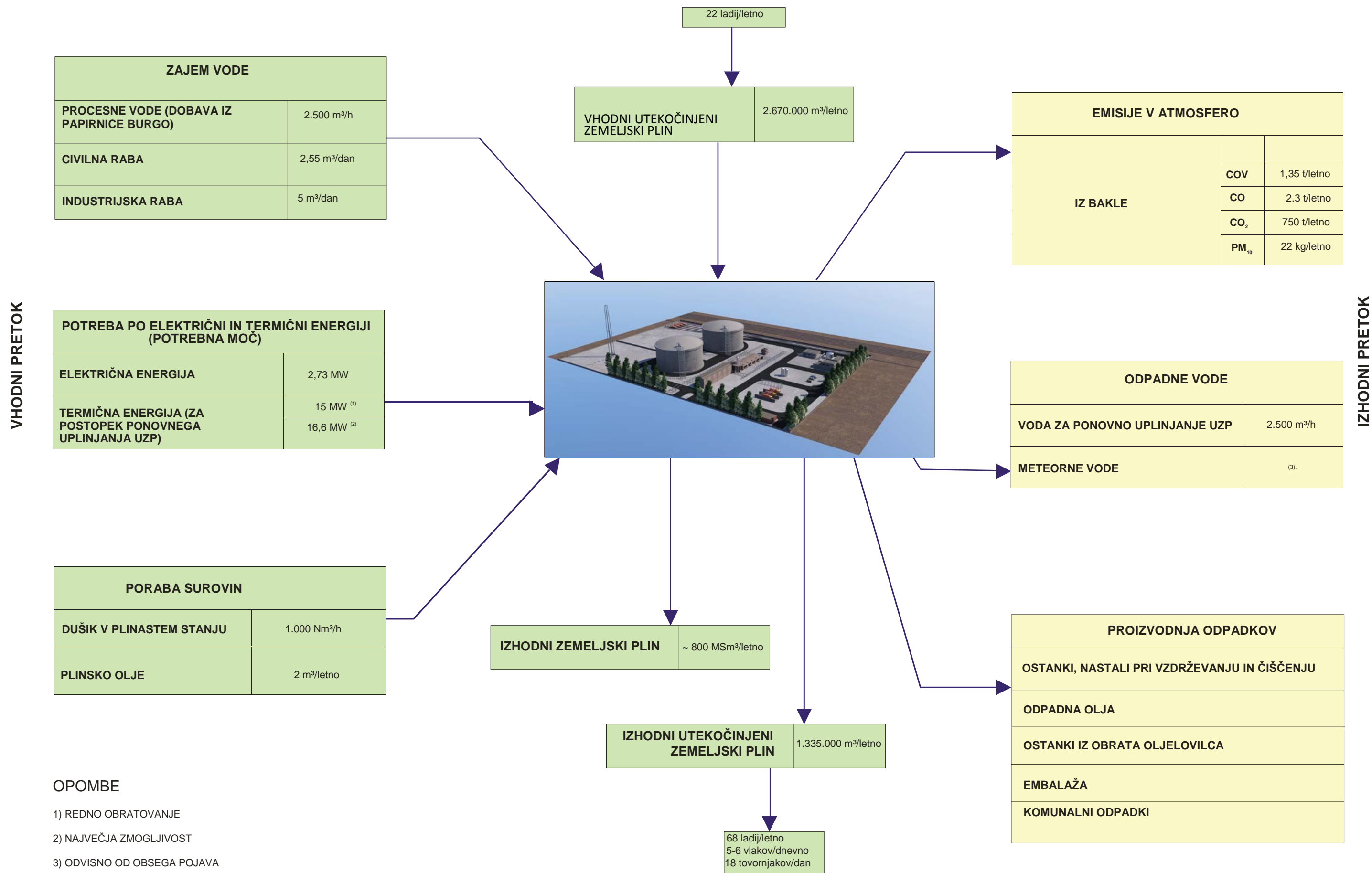
SLIKA 10.1 VHODNI IN IZHODNI PRETOKI
