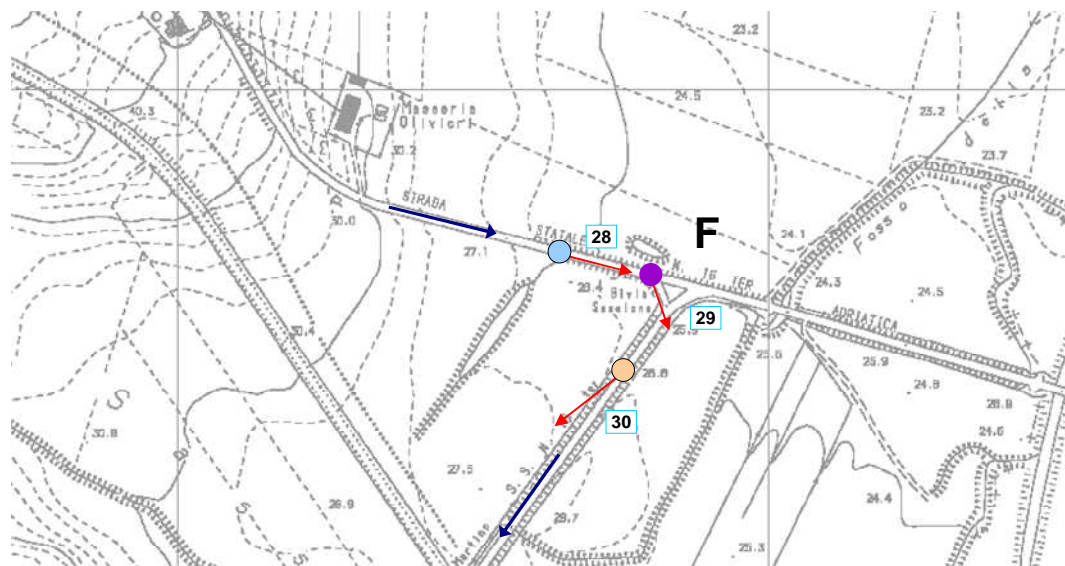
Fig. F6 Proposta progettuale - Punti di ripresa e percorso cavi nella zona del punto F (Bivio Saccione SP166-SP136)
