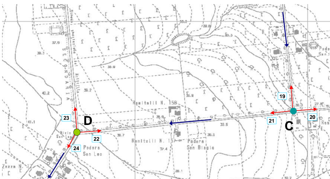
Fig. F4 Proposta progettuale - Punti di ripresa e percorso cavi nella zona dei punti C e D (bivio strada di bonifica-SP126 e bivio SP126-SP128)
