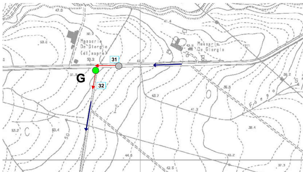
Fig. F7 Proposta progettuale - Punti di ripresa e percorso cavi nella zona del punto G (bivio SP136-sterrata presso Masseria De Giorgio)
