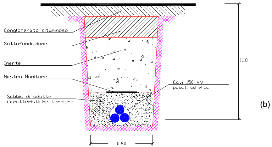
Fig. 15 Schemi di posa per cavi interrati:
