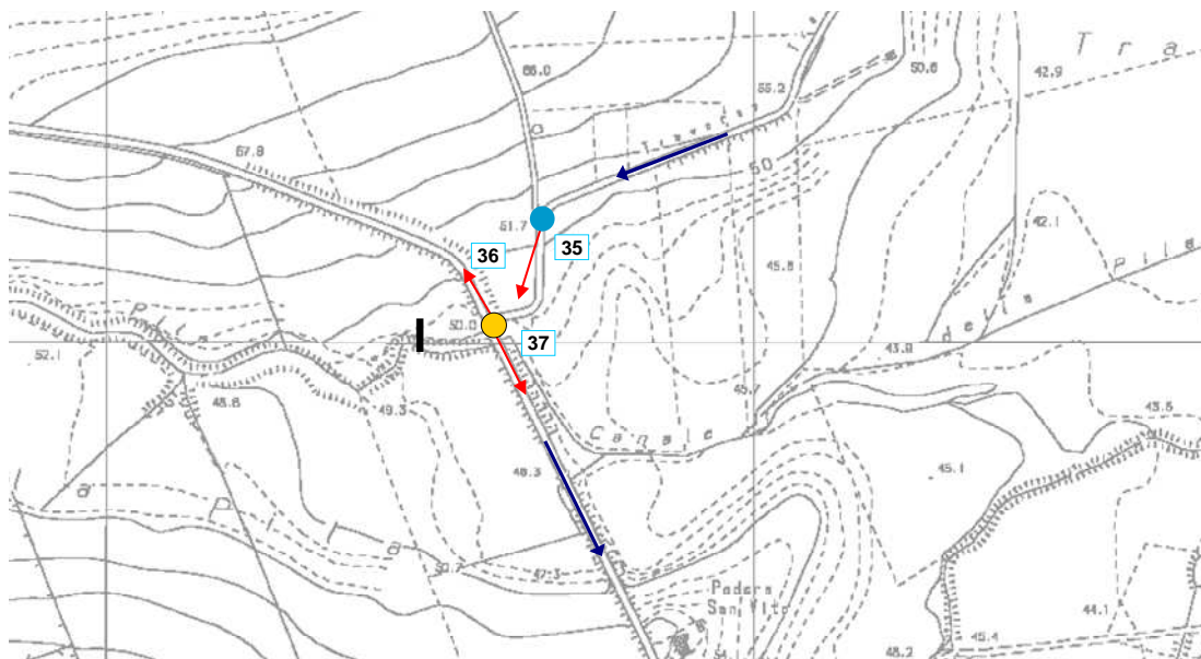
Fig. F9 Proposta progettuale - Punti di ripresa e percorso cavi nella zona del punto I (bivio per la strada comunale di Transure)
