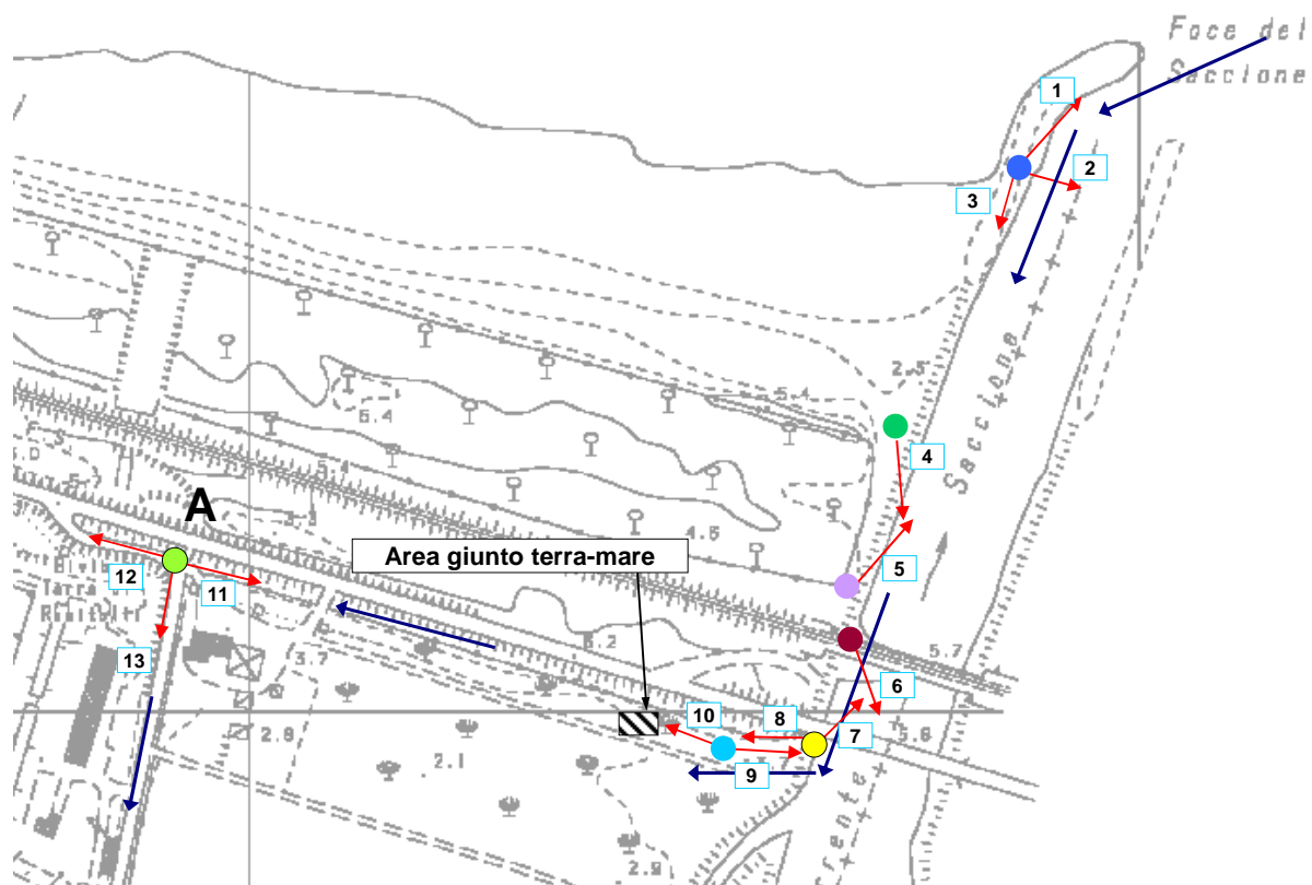
Fig. F1 Proposta progettuale - Punti di ripresa e percorso cavi nella zona d'approdo e punto A
