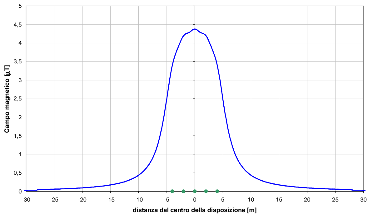
Fig. 21 Andamento del campo magnetico per i collegamenti della rete interna sottomarina a 30 kV : n°5 cavi t ripolari alla profondità di 1 m distanziati di 2 m.
