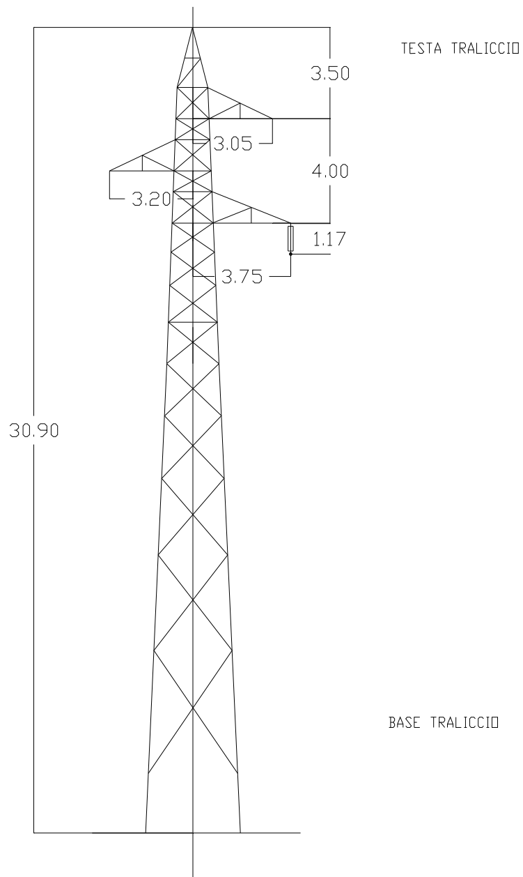
Fig. 18 Traliccio per linea aerea su palificata a 150 kV singola tema destra.
