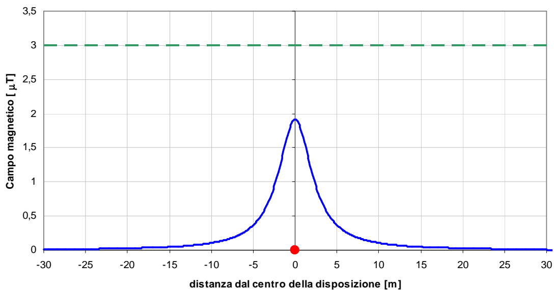
Fig. 20 Andamento del campo magnetico sulla battigia (n°1 cavo tripolare alla profondità di 1,5 m).
