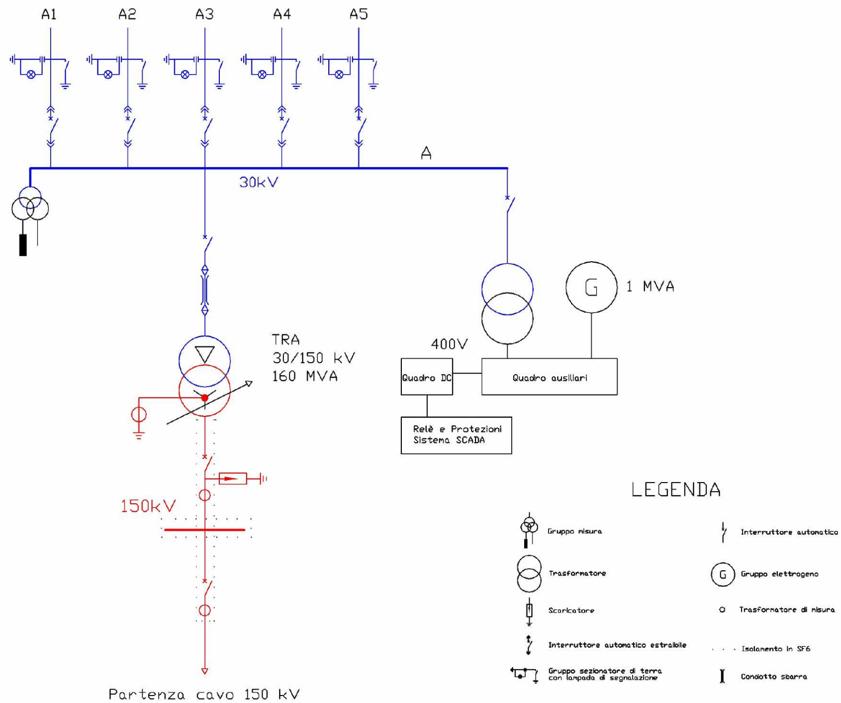
Fig. 13 Schema unifilare di massima della cabina 30/150 kV su piattaforma marina.
