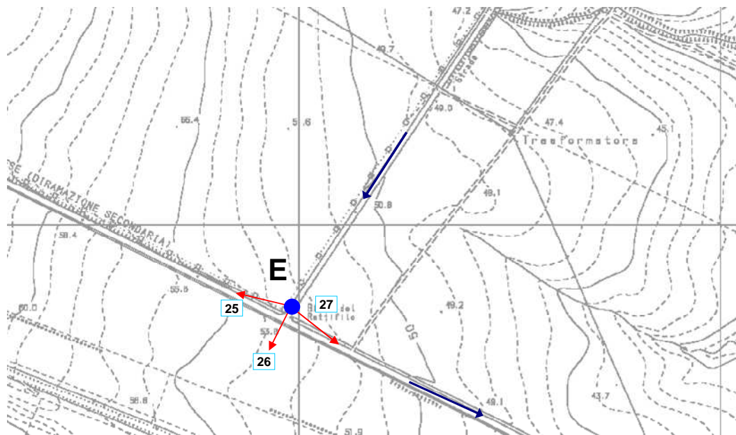
Fig. F5 Proposta progettuale - Punti di ripresa e percorso cavi nella zona del punto E (Bivio del Rettifilo SP128-SP166)
