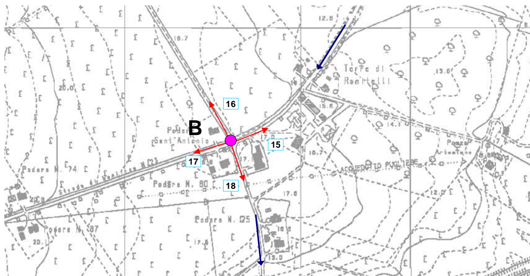
Fig. F3 Proposta progettuale - Punti di ripresa e percorso cavi nella zona Torre di Ramitelli (punto B)
