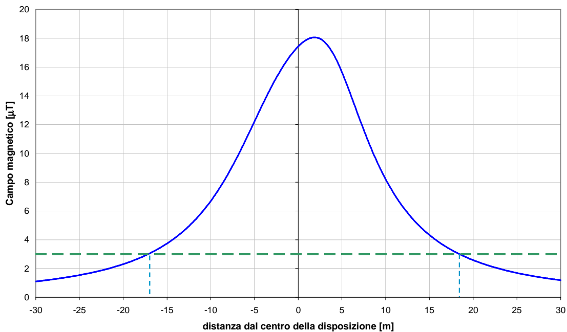
Fig. 23 Andamento del campo magnetico prodotto dalla linea aerea a 150 kV nella sezione di franco minimo da terra (6,4 m).
