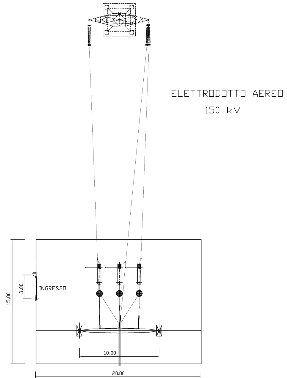
TRANSIZIONE CAVO-AEREO PIANTA
