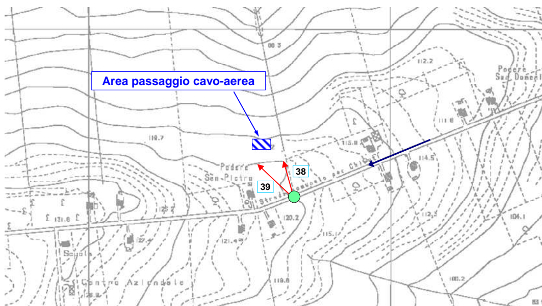
Fig. F10 Proposta progettuale - Punti di ripresa e percorso cavi nella zona di passaggio da cavi interrati a linea aerea
