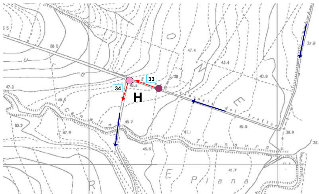
Fig. F8 Proposta progettuale - Punti di ripresa e percorso cavi nella zona del punto H (bivio tra le due strade sterrate)
