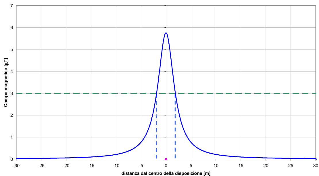
Fig. 22 Andamento del campo magnetico lungo il percorso dei cavi terrestri a 150 kV (n°1 terna di cavi unipolari in piano).
