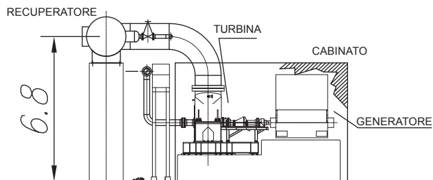
VISTA B-B
