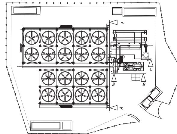
PIANTA CHIAVE
