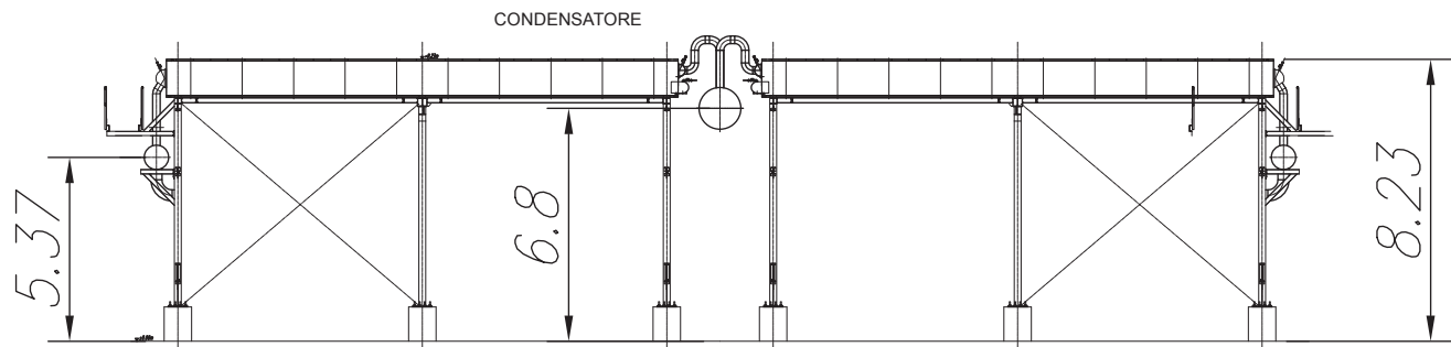
VISTA A-A
