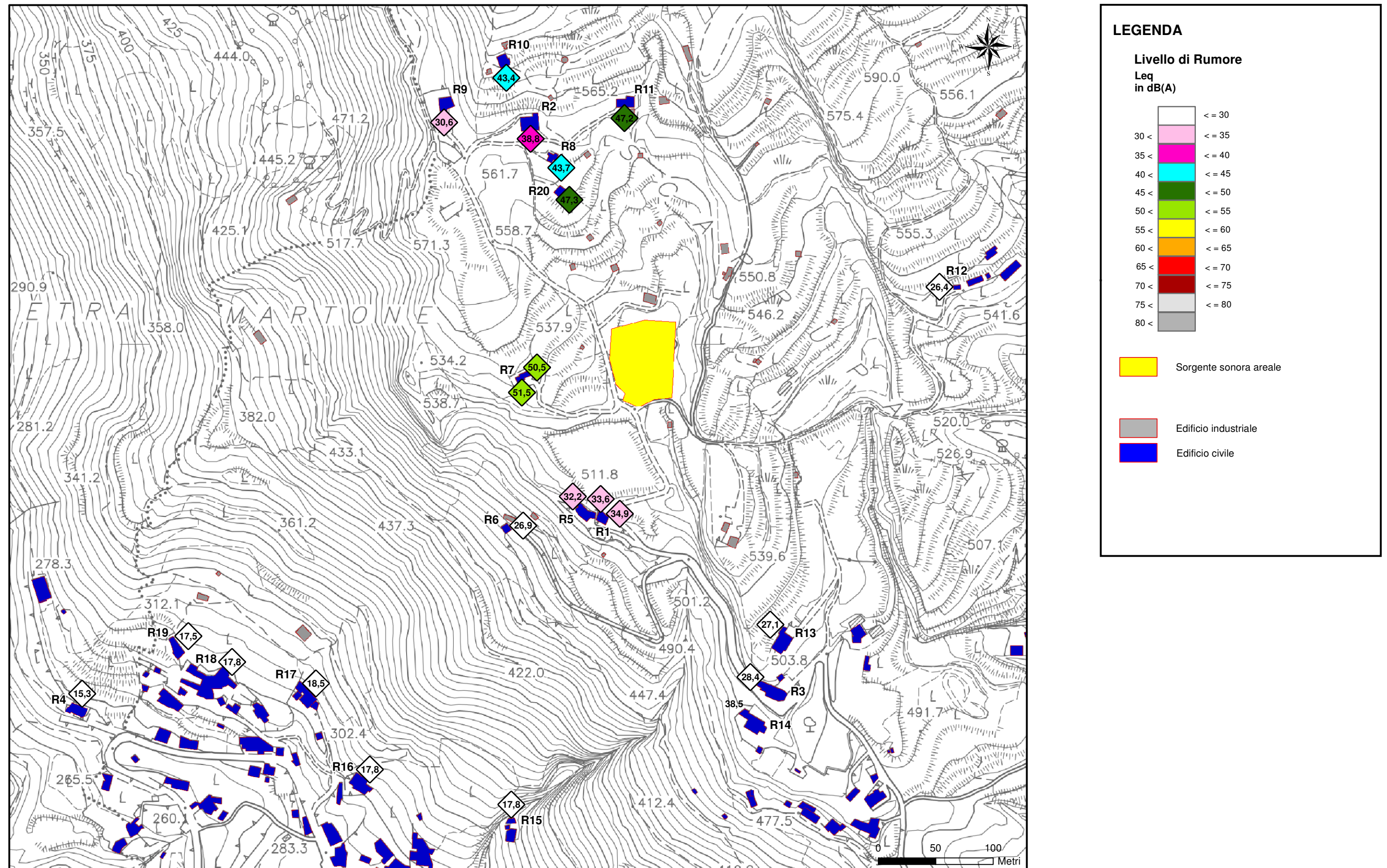
Figura 5.4.2a Laeq durante le Attività di Cantiere per la Realizzazione dell'Impianto ORC - Periodo Diurno
