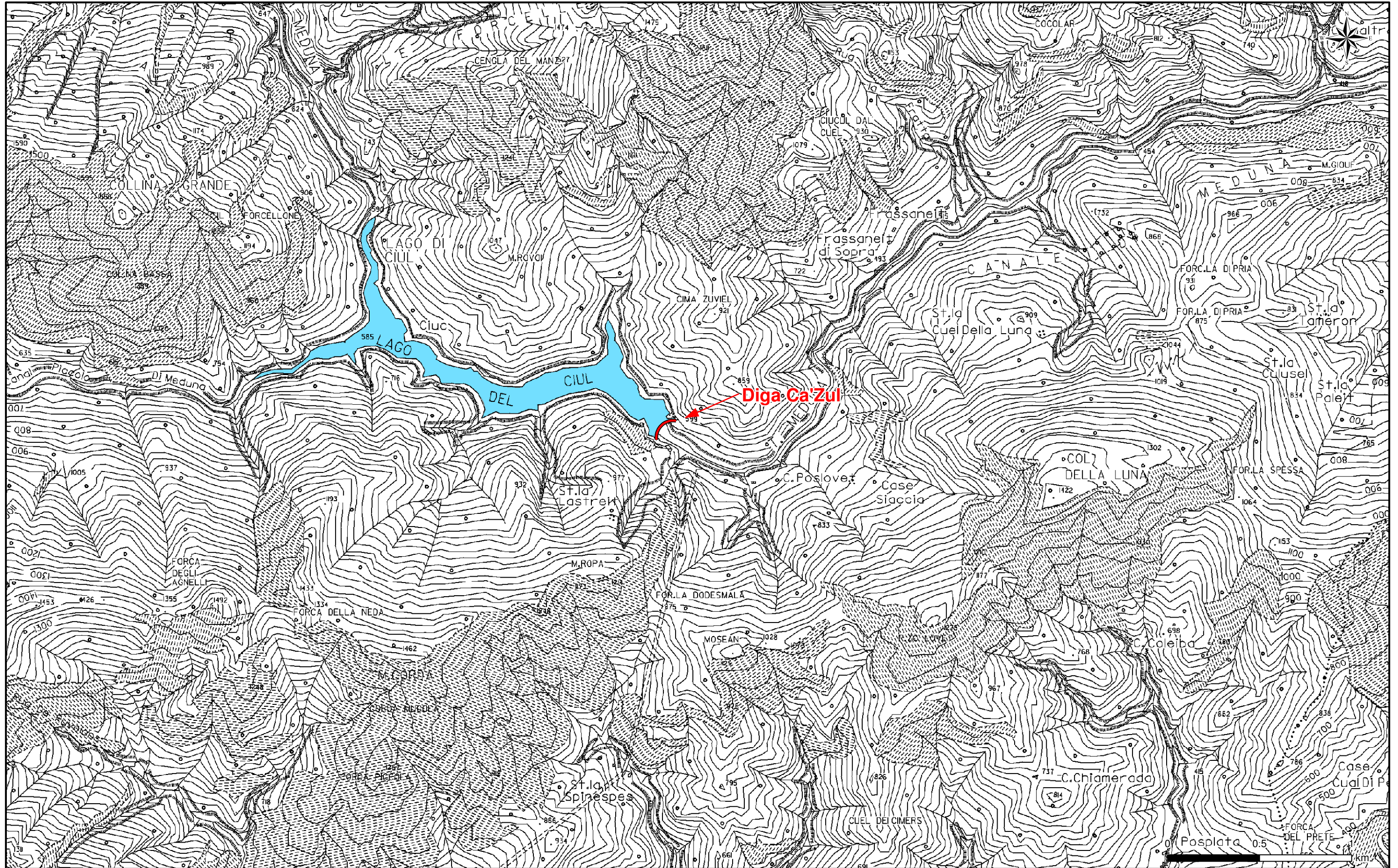
Figura 3.1a Localizzazione diga Ca 'Zul (Scala 1:20.000)
