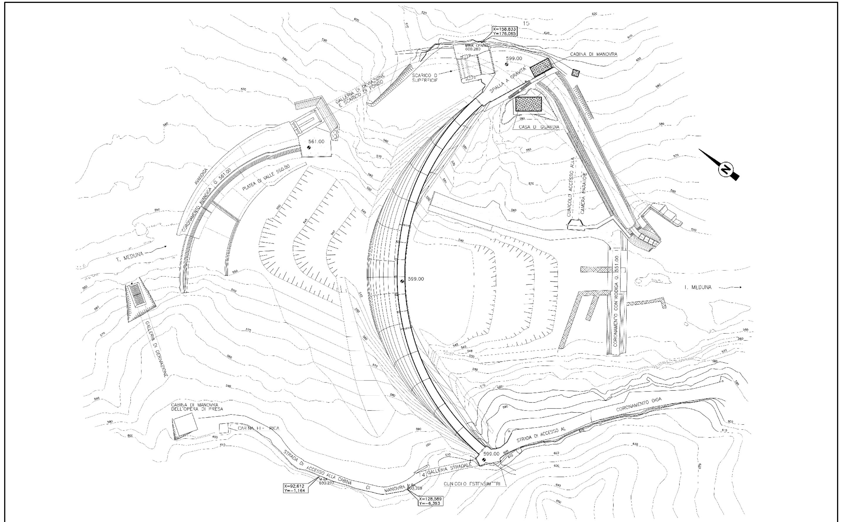
Figura 3a Diga Ca 'Zul - Stato di fatto
