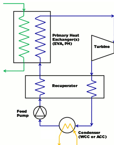
Figura 1 - Tipico diagramma di flusso per ORC
