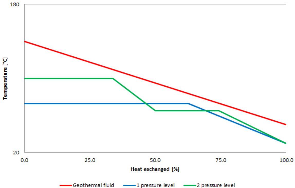
Figura 2 – Diagramma Temperatura – Calore scambiato di confronto tra cicli ottimizzati a 1 e 2 livelli di pressione
