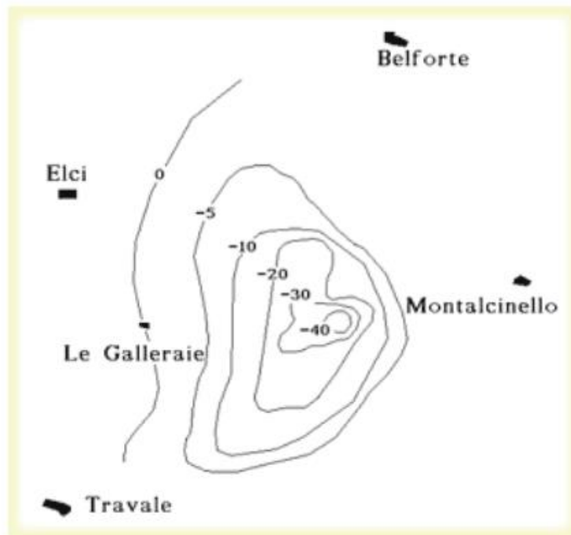
Figura 6-1. Subsidenza nel campo di vapore di Travale-Radicondoli per il periodo 1973-1991 (Di Filippo et al., 1995).
