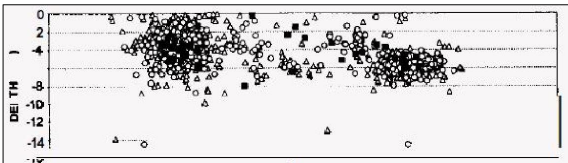
Figura 5-3. Mappa degli ipocentri per l'area di Larderello-Travale per il periodo 1977-1993 secondo la sezione AA' di Figura 5-2 (Batini et al., 1995).
