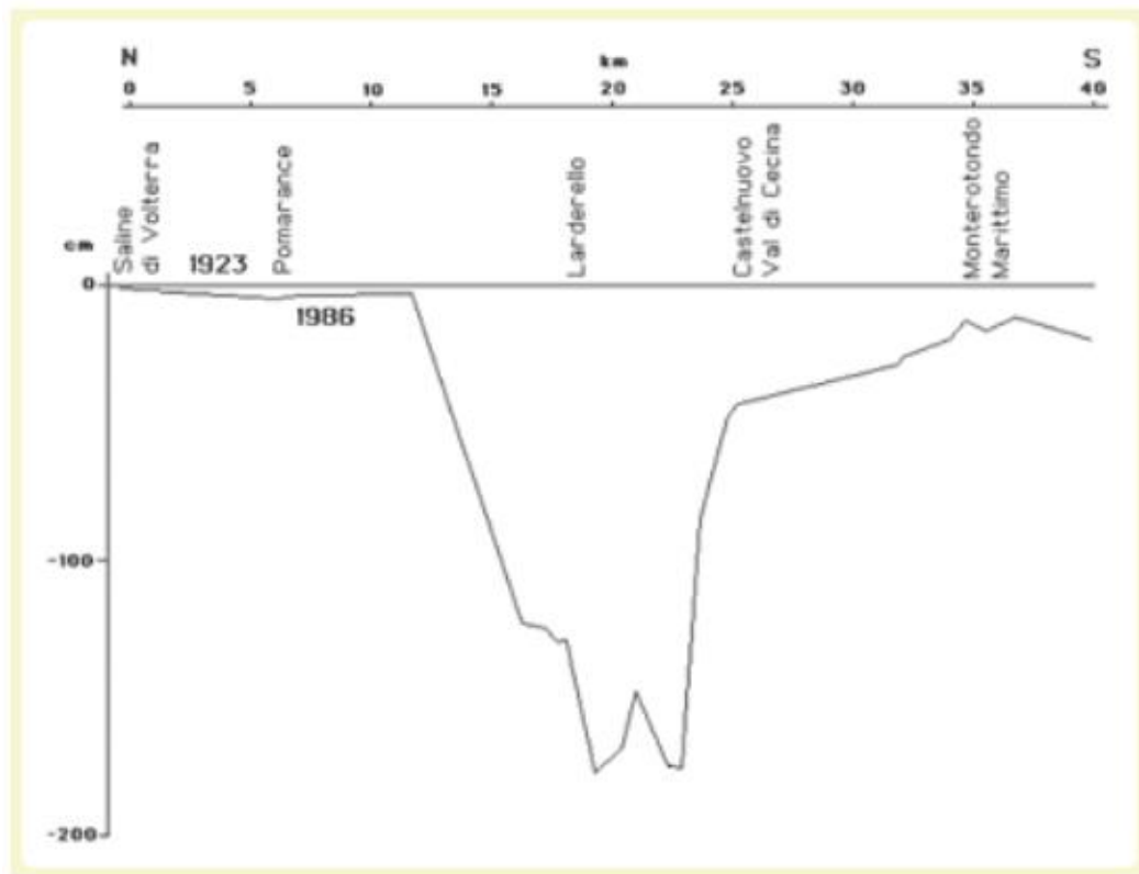
Figura 6-2. Subsidenza nell'area di Larderello tra il 1923 ed il 1986 (ENEL, 1995).
