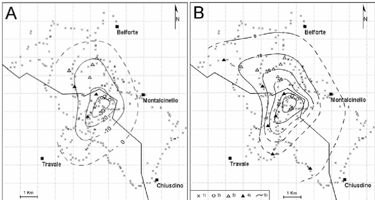
Figura 6-3. Andamento della variazione di quota (cm): A) durante il periodo 1973-1988; B) durante il periodo 1973-2003 (Ciulli et al., 2005).
