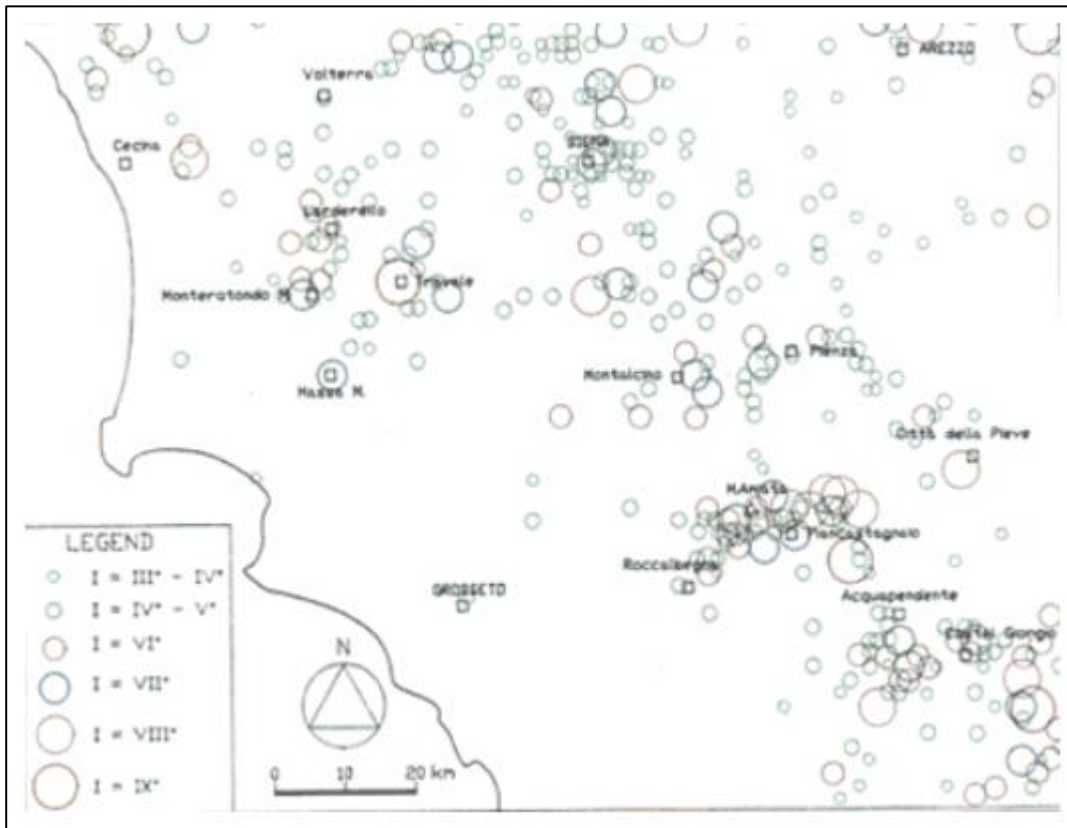
Figura 5-1. Sismicità storica locale della Toscana meridionale nel periodo 1900-1990: distribuzione degli epicentri ed intensità degli eventi (scala MCS) (ENEL, 1995, http://www.arpat.toscana.it/temi-ambientali/aria/aree-geotermiche/geotermia/progetto-geotermia-sismicita ).
