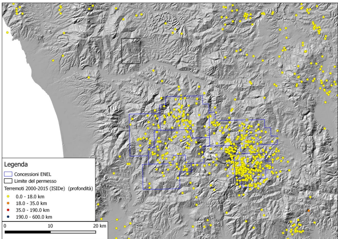
Figura 5-6. Ubicazione dei terremoti per le aree geotermiche di Larderello e Travale nel periodo 2000-2015 suddivisi per profondità (ISIDE-Italian Seismological Instrumental and Parametric Data-Base).
