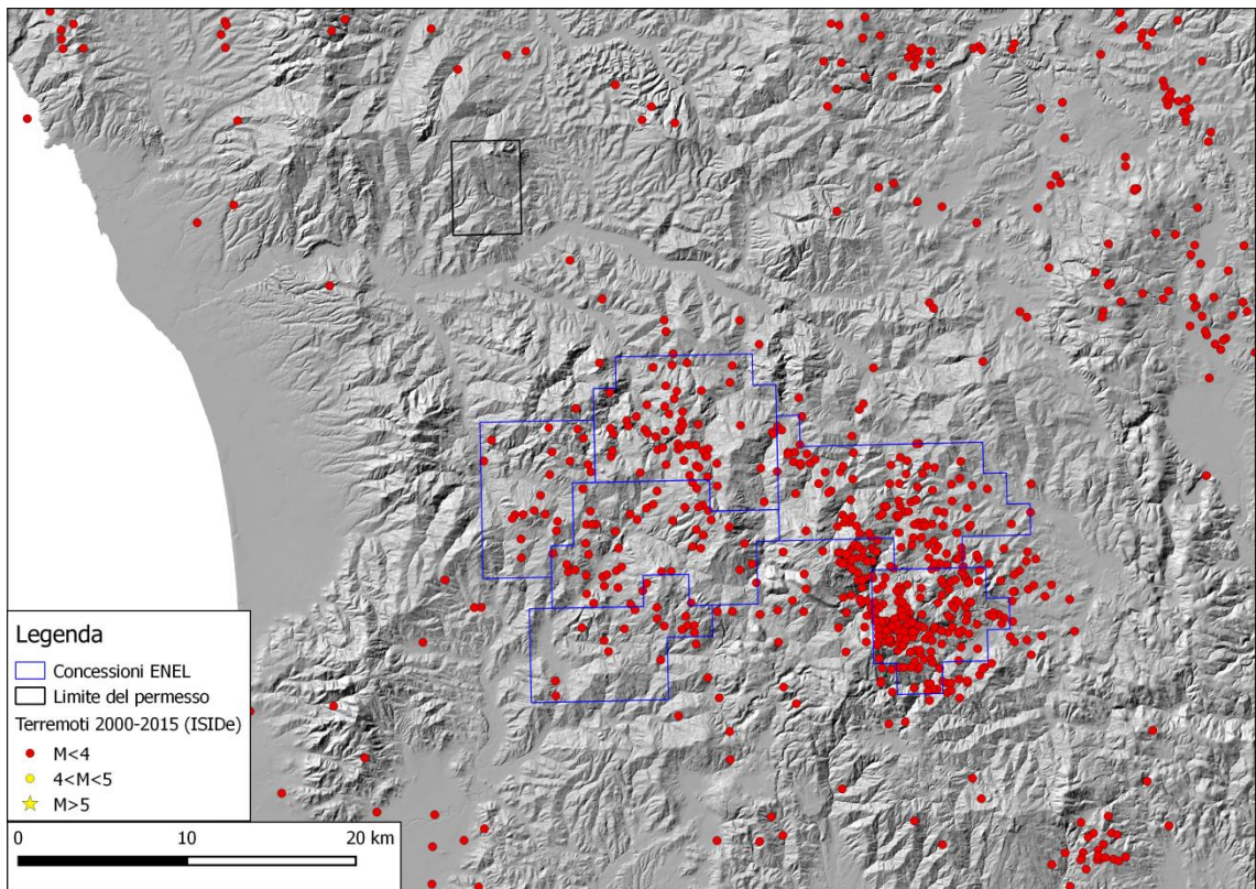
Figura 5-5. Ubicazione dei terremoti per le aree geotermiche di Larderello e Travale nel periodo 2000-2015 suddivisi per magnitudo (ISIDE-Italian Seismological Instrumental and Parametric Data-Base).
