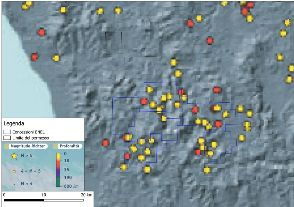
Figura 5-4. Ubicazione dei terremoti per le aree geotermiche di Larderello e Travale nel periodo 1982-2002 (Carta della sismicità in Italia, INGV 2004).
