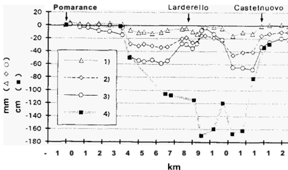
Figura 6-5. Variazione di quota lungo il profilo Pomarance-Larderello-Castelnuovo V.C.. Periodo: 1) 1989-89; 2) 1991-86; 3) 1993-86; 4) 1986-23 (Dini et al., 1995)
