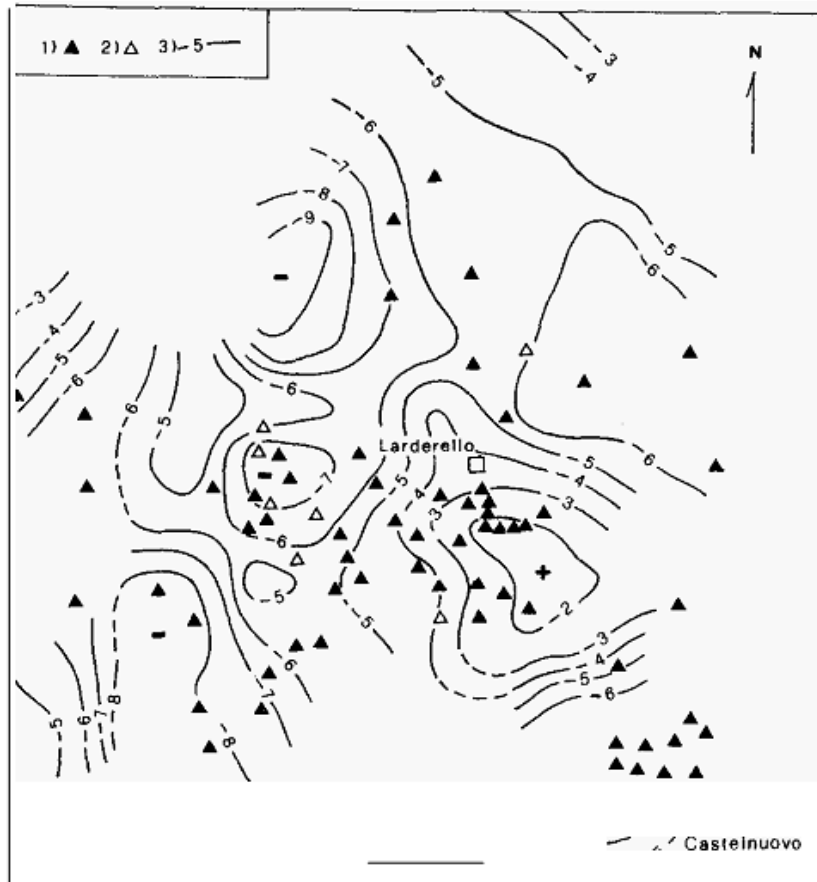
Figura 6-4. Variazioni di quota durante il periodo di rilevamento 1986-1993. 1) pozzi di produzione; 2) pozzi di reiniezione; 3) linee di variazione di quota (Dini et al., 1995).
