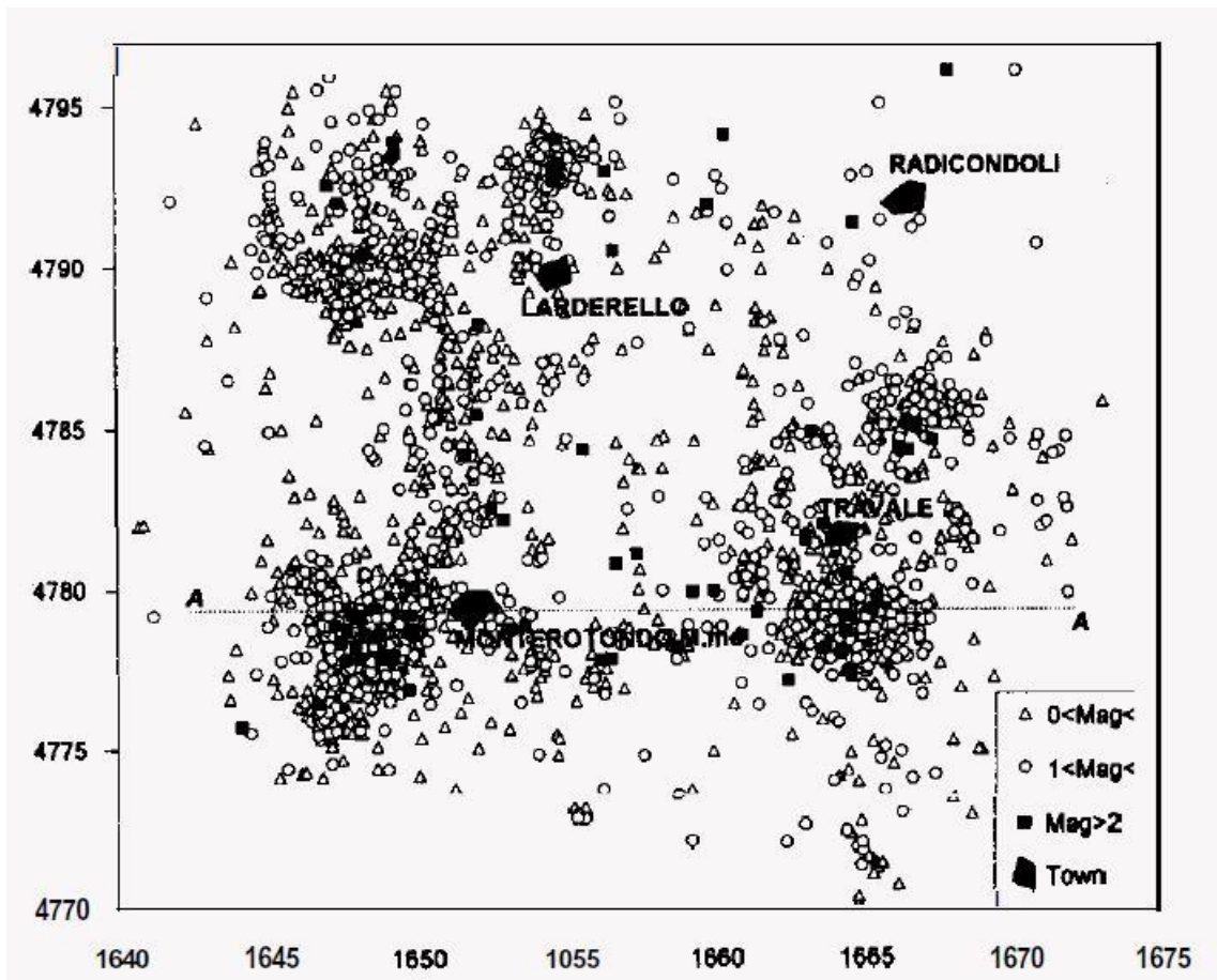
Figura 5-2. Mappa degli epicentri per l'area di Larderello-Travale per il periodo 1977-1993 (Batini et al., 1995).
