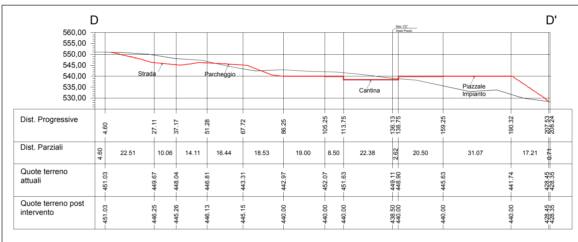
SEZIONE DD' (SE-NW) 1:1000
