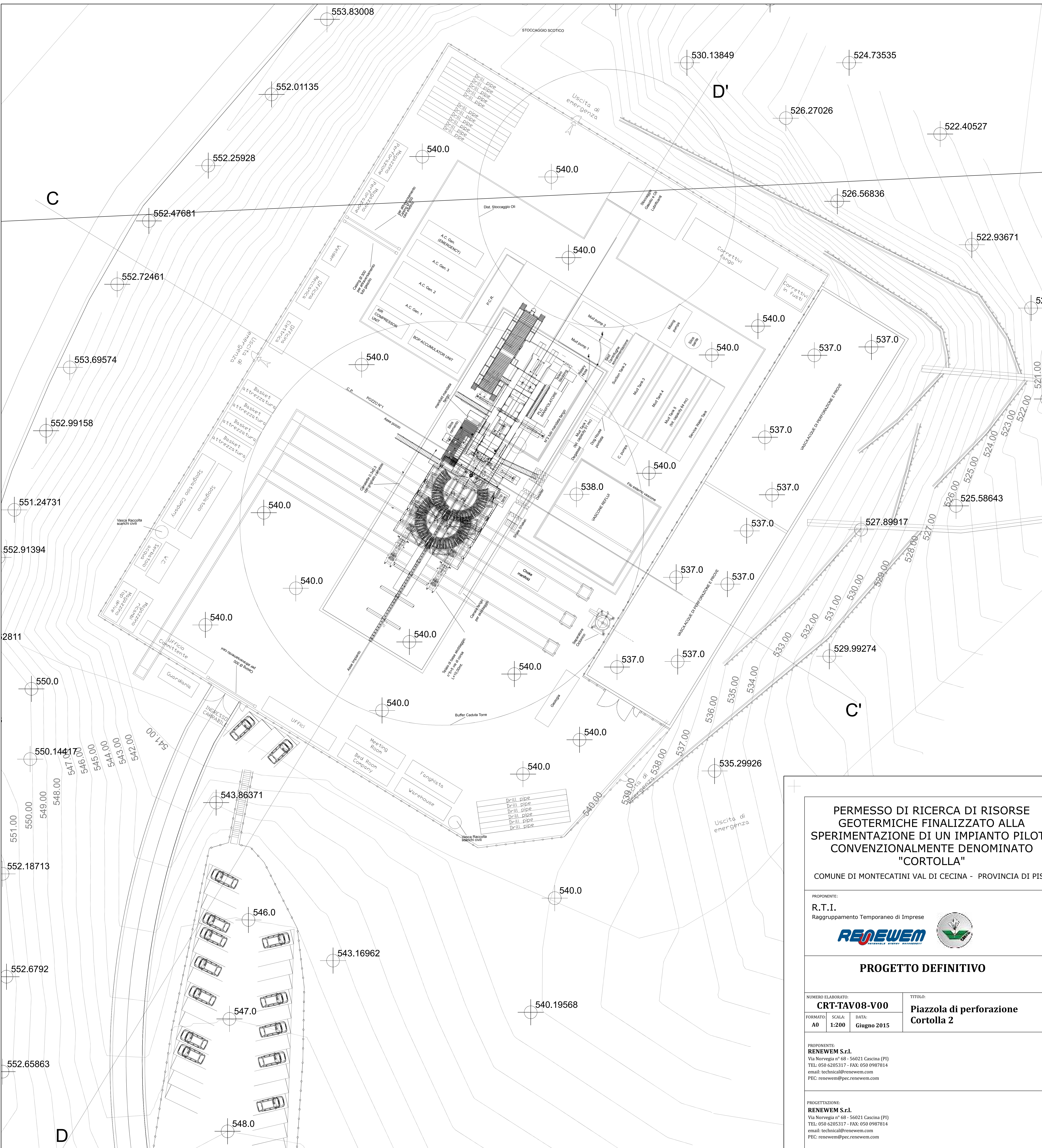
PIAZZOLA DI PERFORAZIONE CORTOLLA 2 - 1:200
