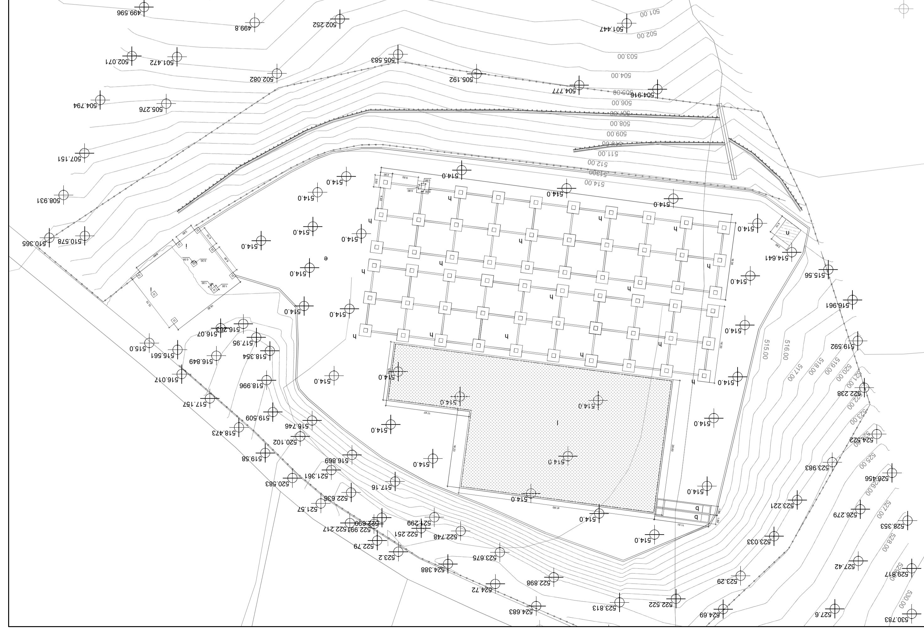
OPERE CIVILI PIAZZALE IMPIANTO - 1:500
