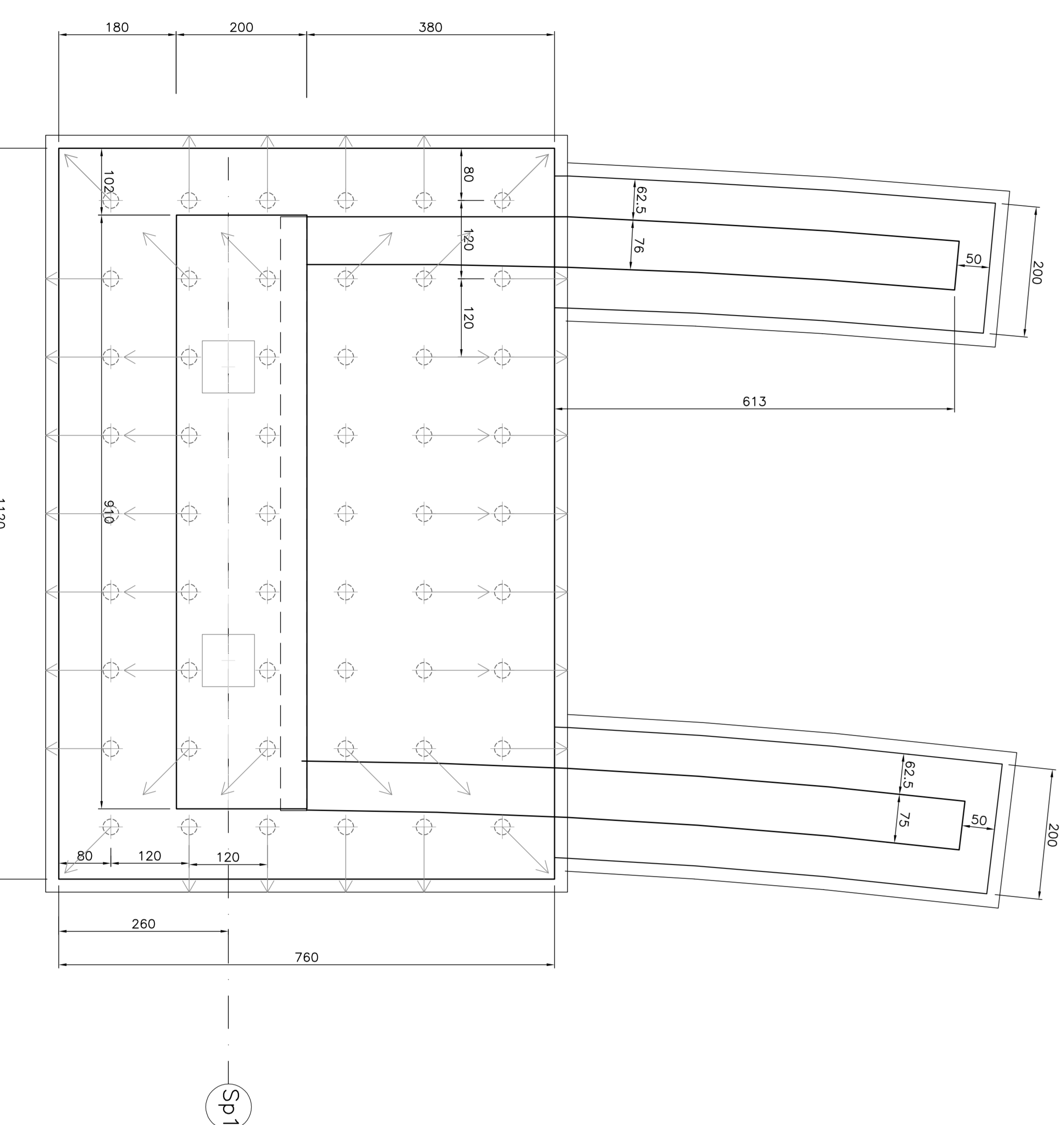
PIANTA FONDAZIONE SPALLA "SP1"
