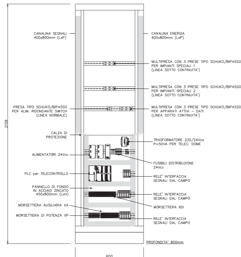
SEZIONE (FONDO TELAIO)
