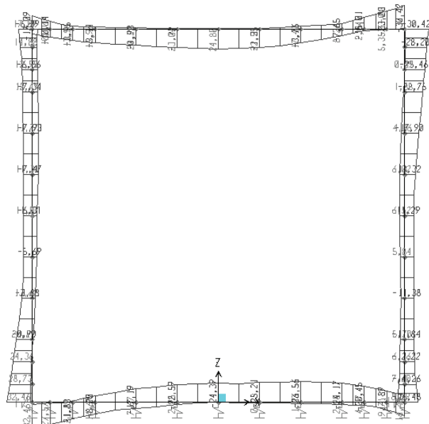
Figura 30 – Azioni flettenti – INVRARA
