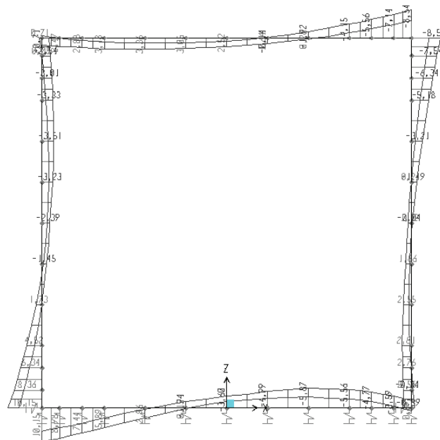
Figura 33 – Azioni flettenti – INVSISMICA
