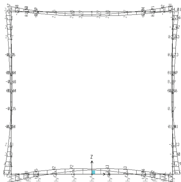
Figura 32 – Azioni flettenti – INVQUASIPERMANENTE
