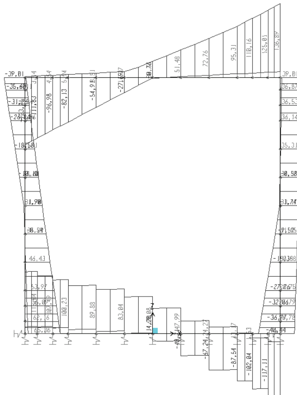
Figura 29 – Azioni taglianti – INVSTRU
