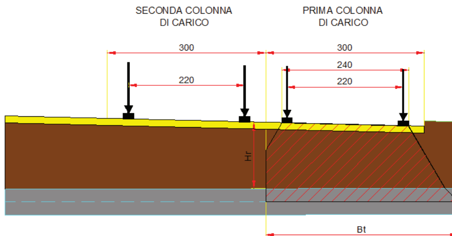
Figura 4 – Diffusione trasversale del carico mobile
