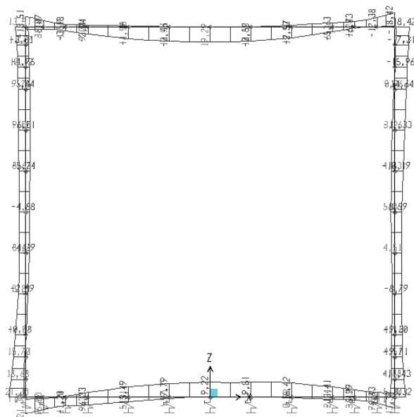
Figura 31 – Azioni flettenti – INVFREQUENTE
