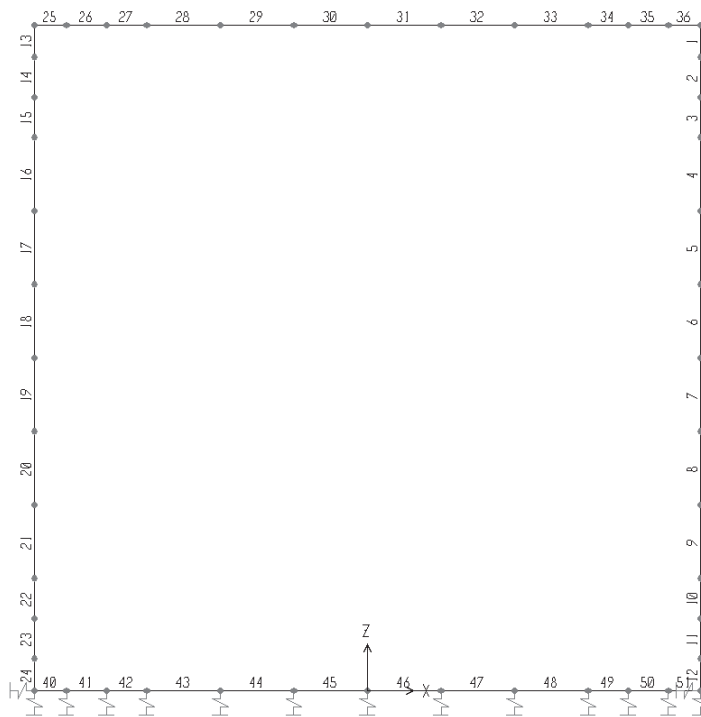
Figura 2 – Numerazione delle aste
