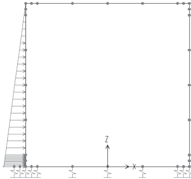
Figura 8 – SPINTA DELLE TERRE ST2S: spinta a riposo
