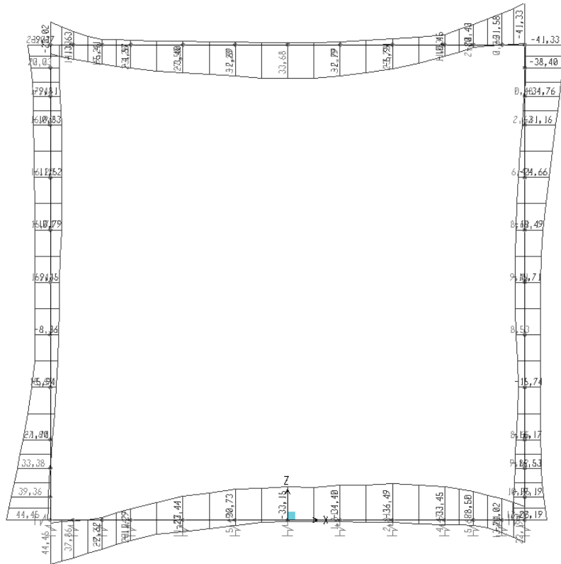
Figura 28 – Azioni flettenti – INVSTRU
