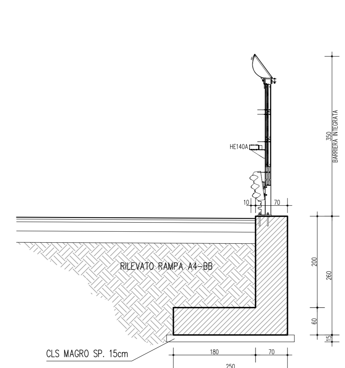
MURO TIPO -2- SEZIONE TRASVERSALE 1:50
