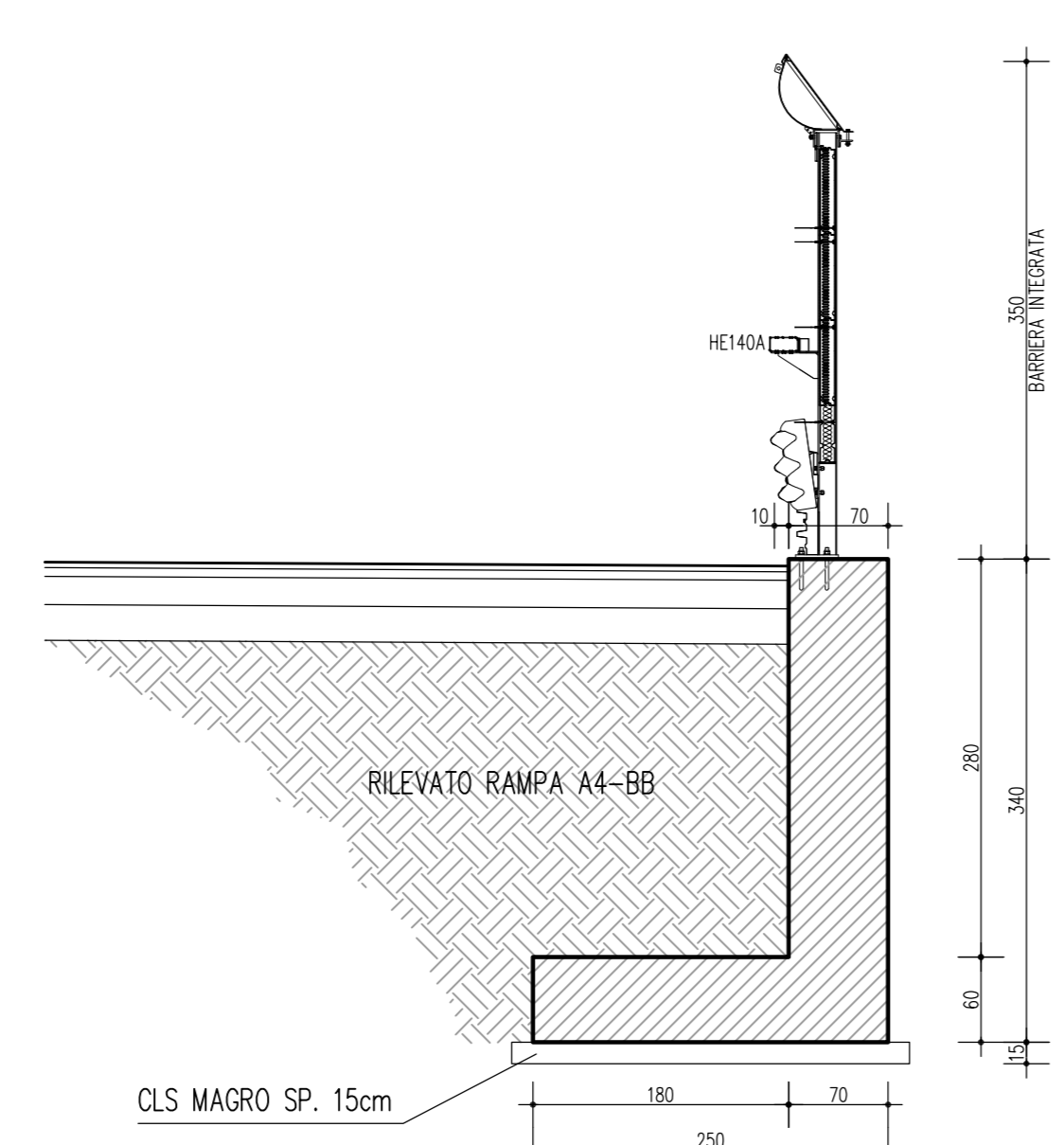
MURO TIPO -1- SEZIONE TRASVERSALE 1:50
