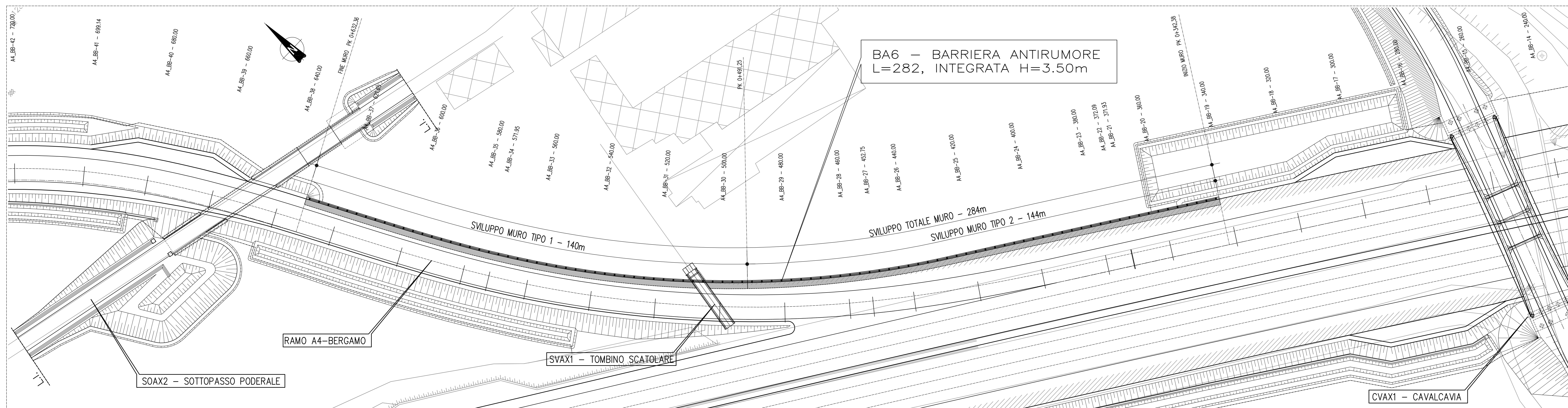
MURO TIPO -1- PIANTA 1:200
