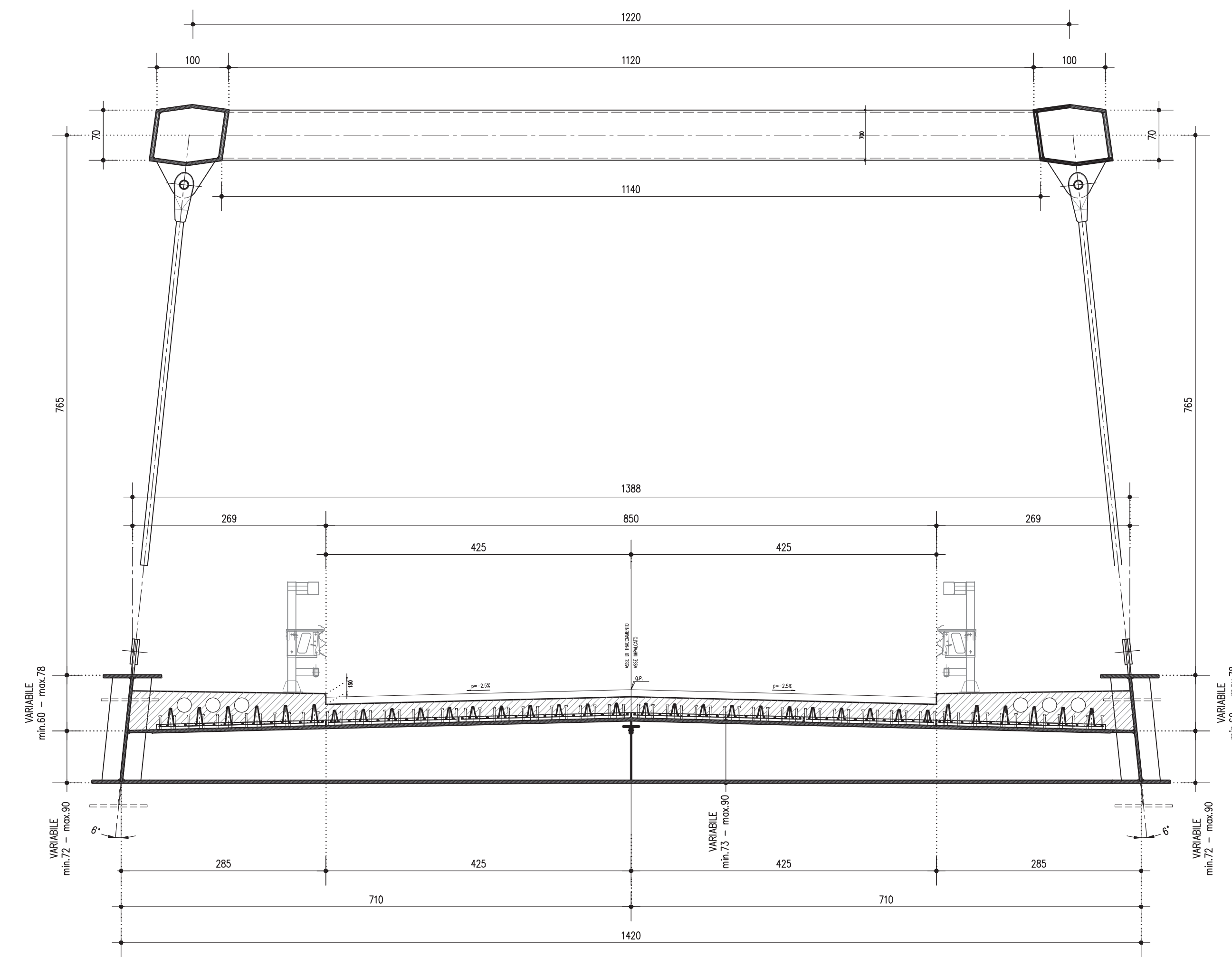
SEZIONE TRASVERSALE A-A 1:50
