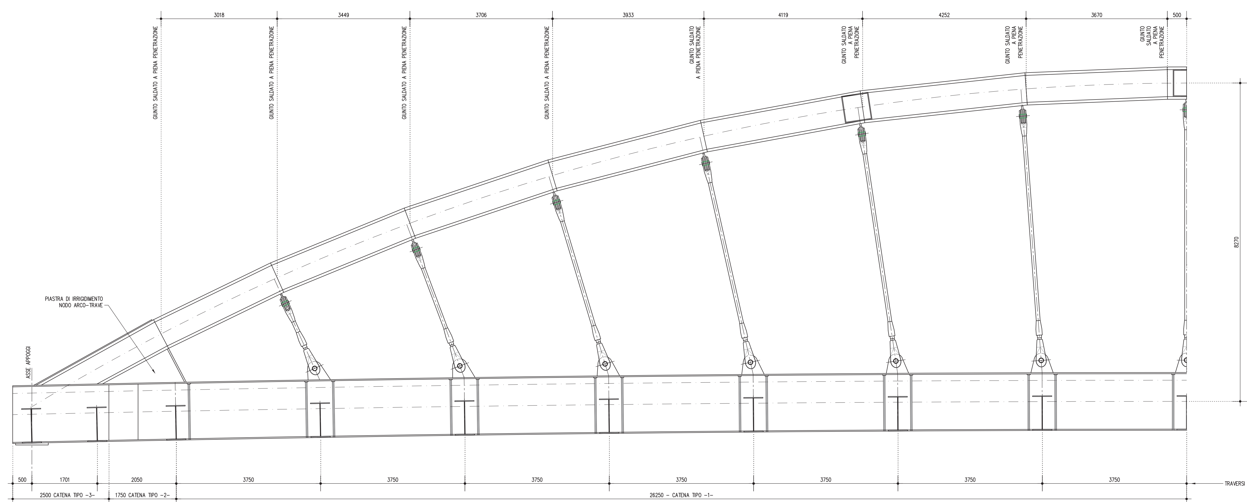
1/2 SEZIONE LONGITUDINALE scala 1:50
