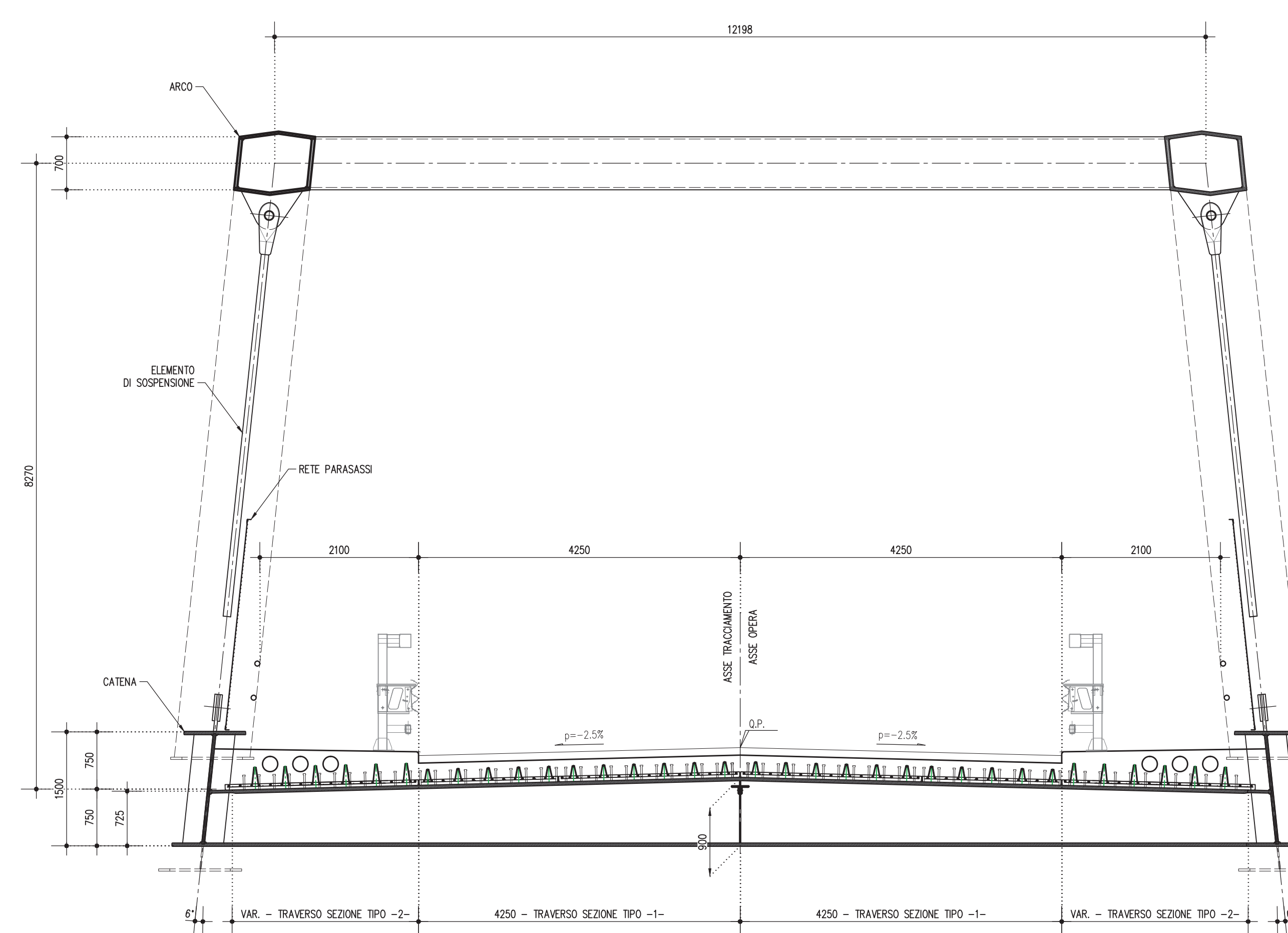
SEZIONE TRASVERSALE DI MEZZERIA scala 1:50
