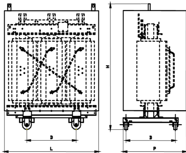
Esecuzione con armadio di protezione
