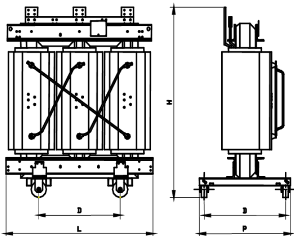
Esecuzione giorno IP00
