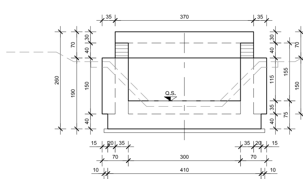
SEZIONE B-B Scala 1:50
