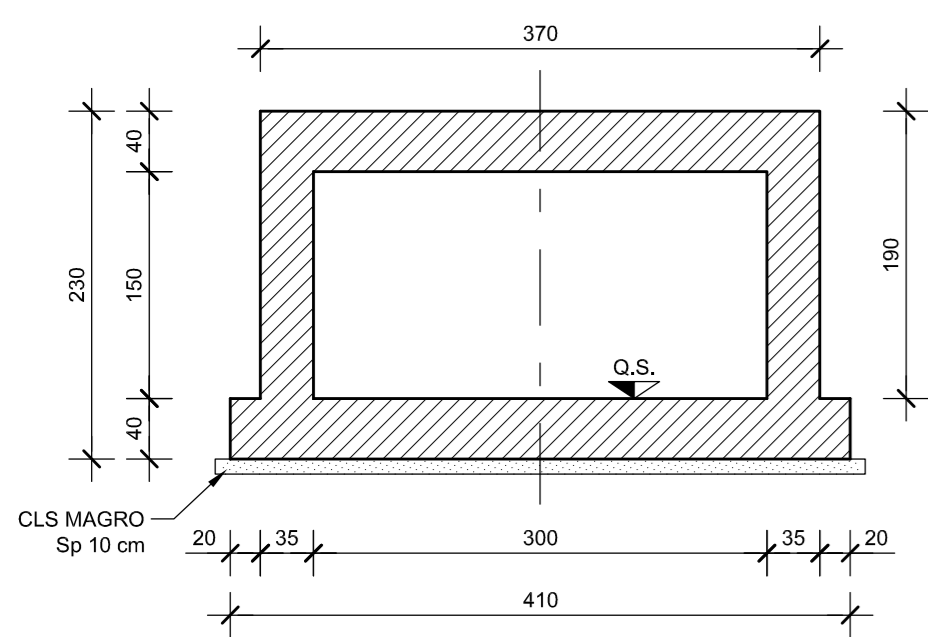
SEZIONE A-A Scala 1:50
