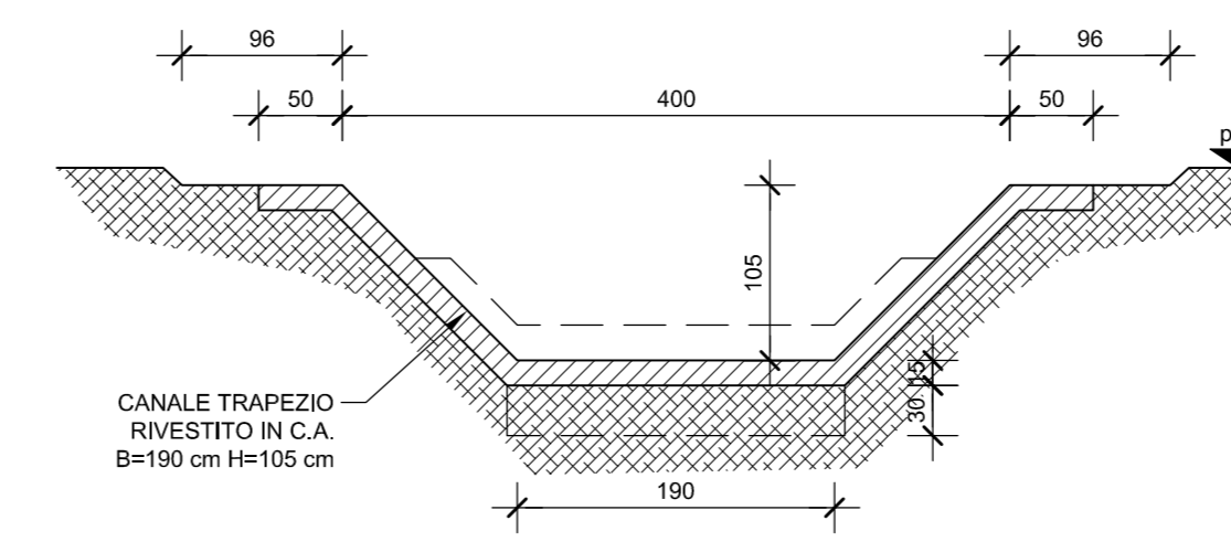
SEZIONE C-C CANALE RIVESTITO IN C.A. Scala 1:50
