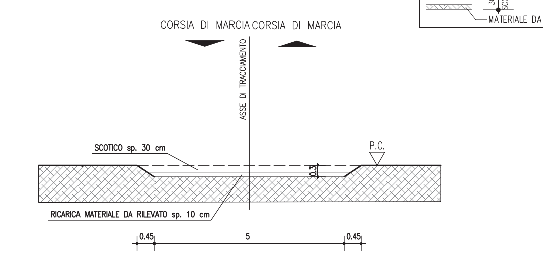
SEZIONE PISTA DI CANTIERE PROVVISORIA (TIPO C) SCALA 1:100
