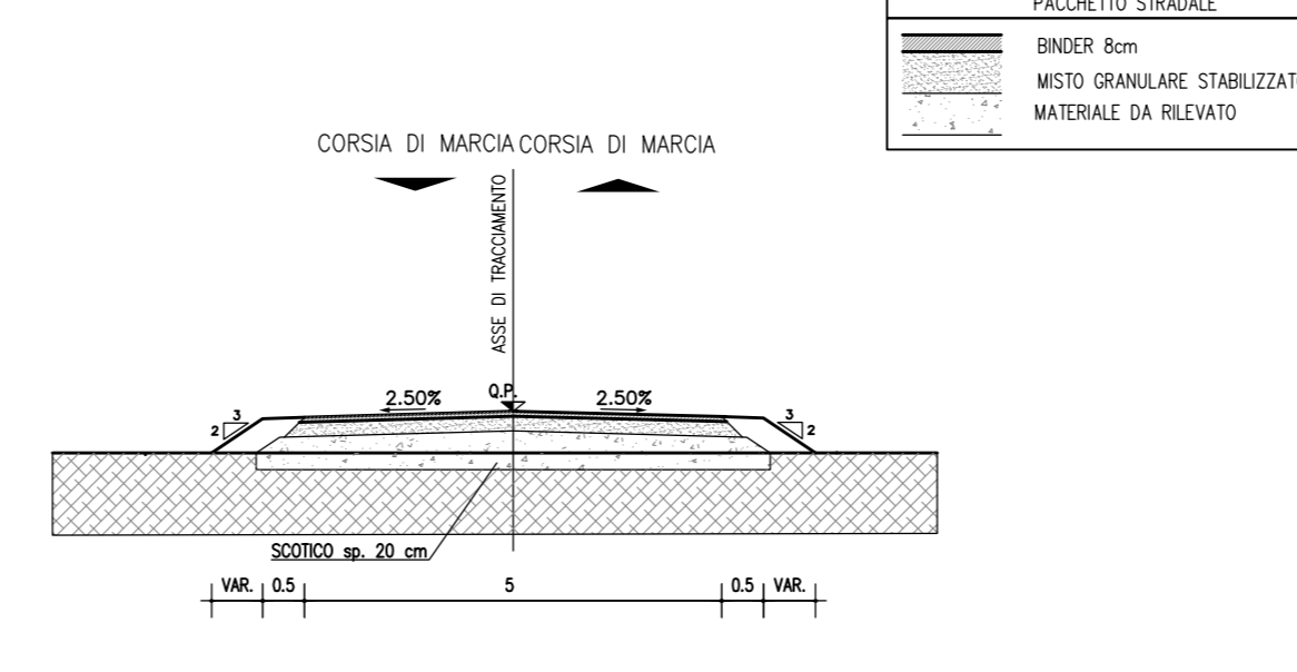
SEZIONE PISTA DI CANTIERE PAVIMENTAZIONE BITUMATA (TIPO B) SCALA 1:100
