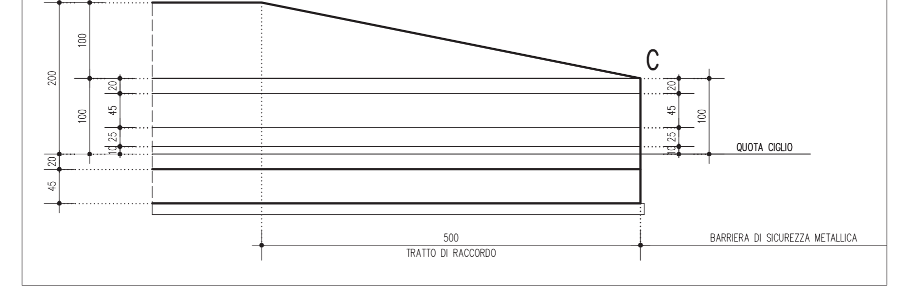
SEZIONE TRASVERSALE TRATTO B-C 1:50
