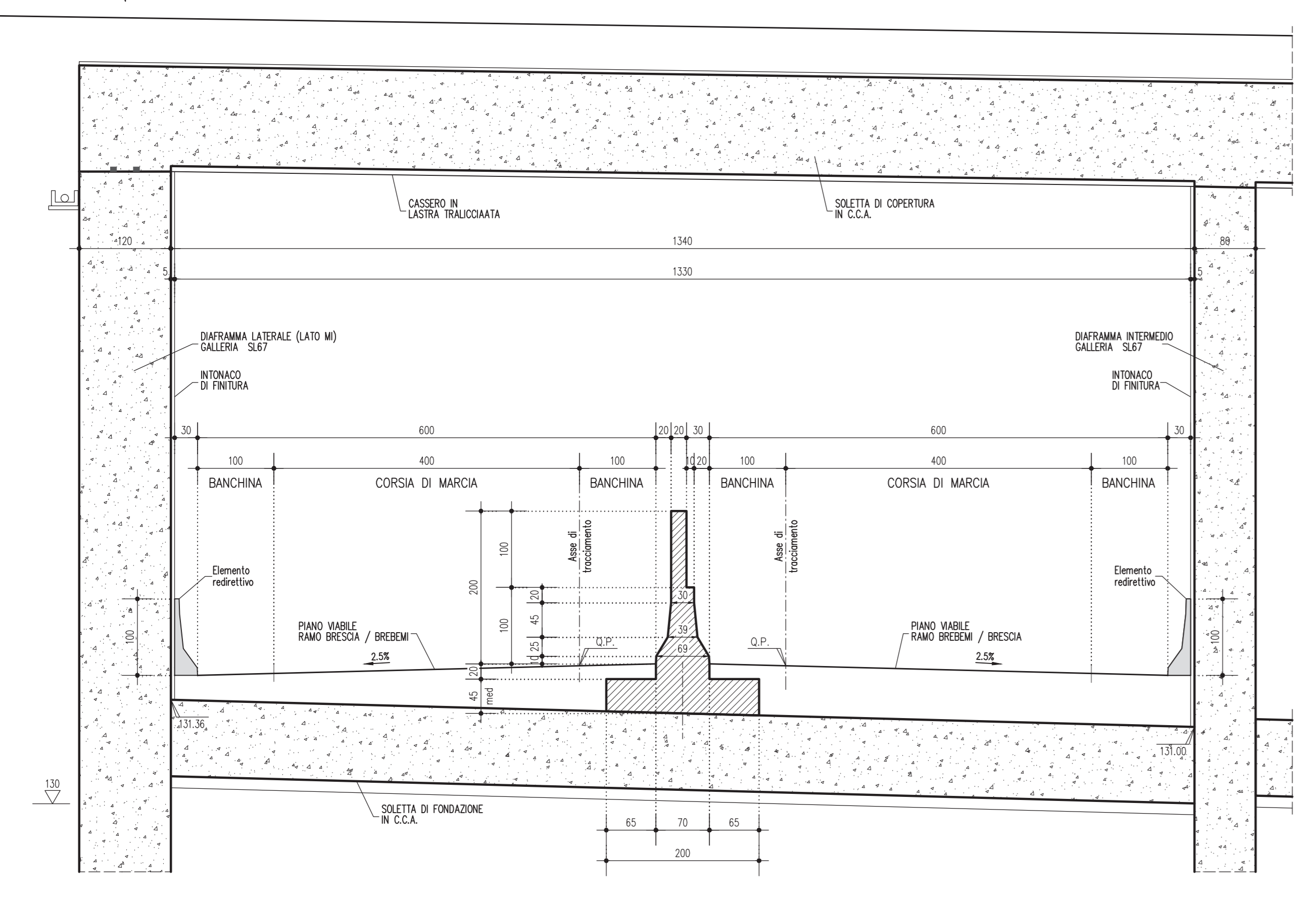
SEZIONE TRASVERSALE TRATTO A-B 1:50
