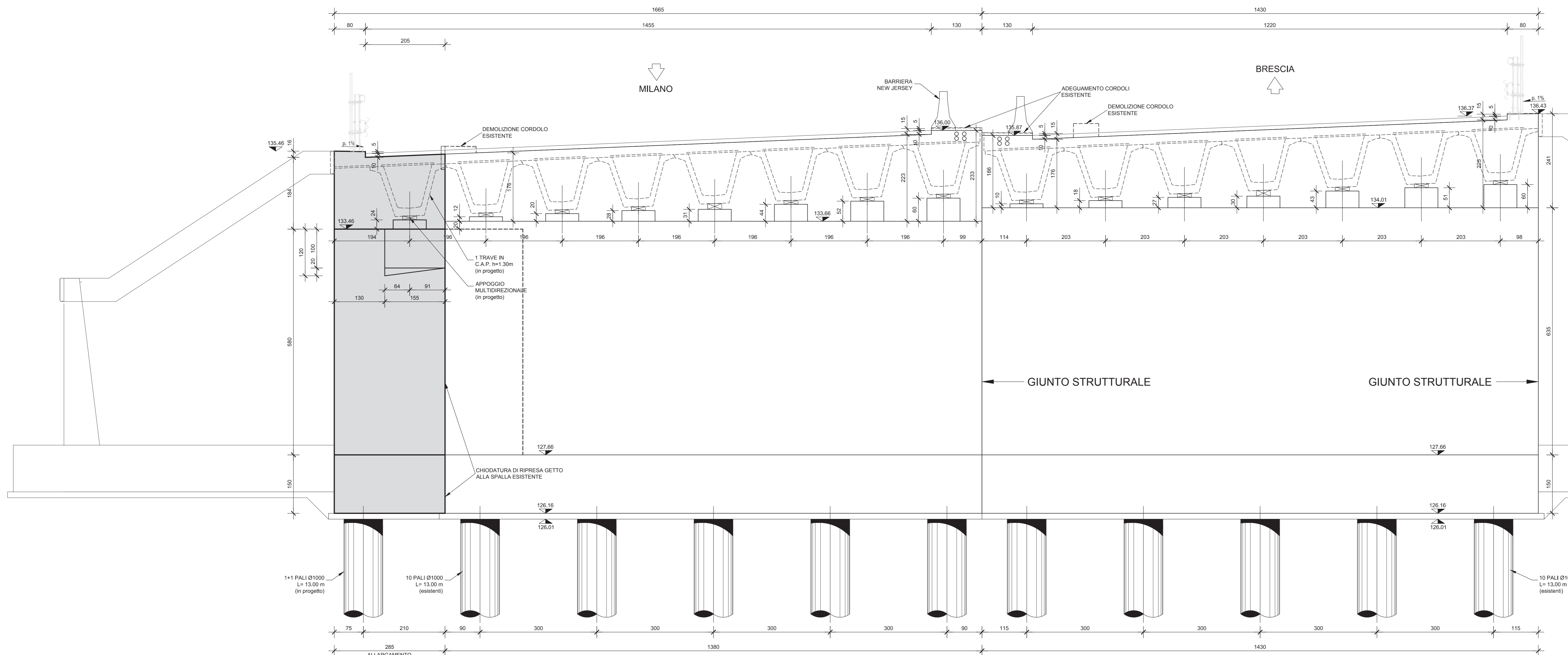
PROSPETTO SPALLA 4 Scala 1:50
