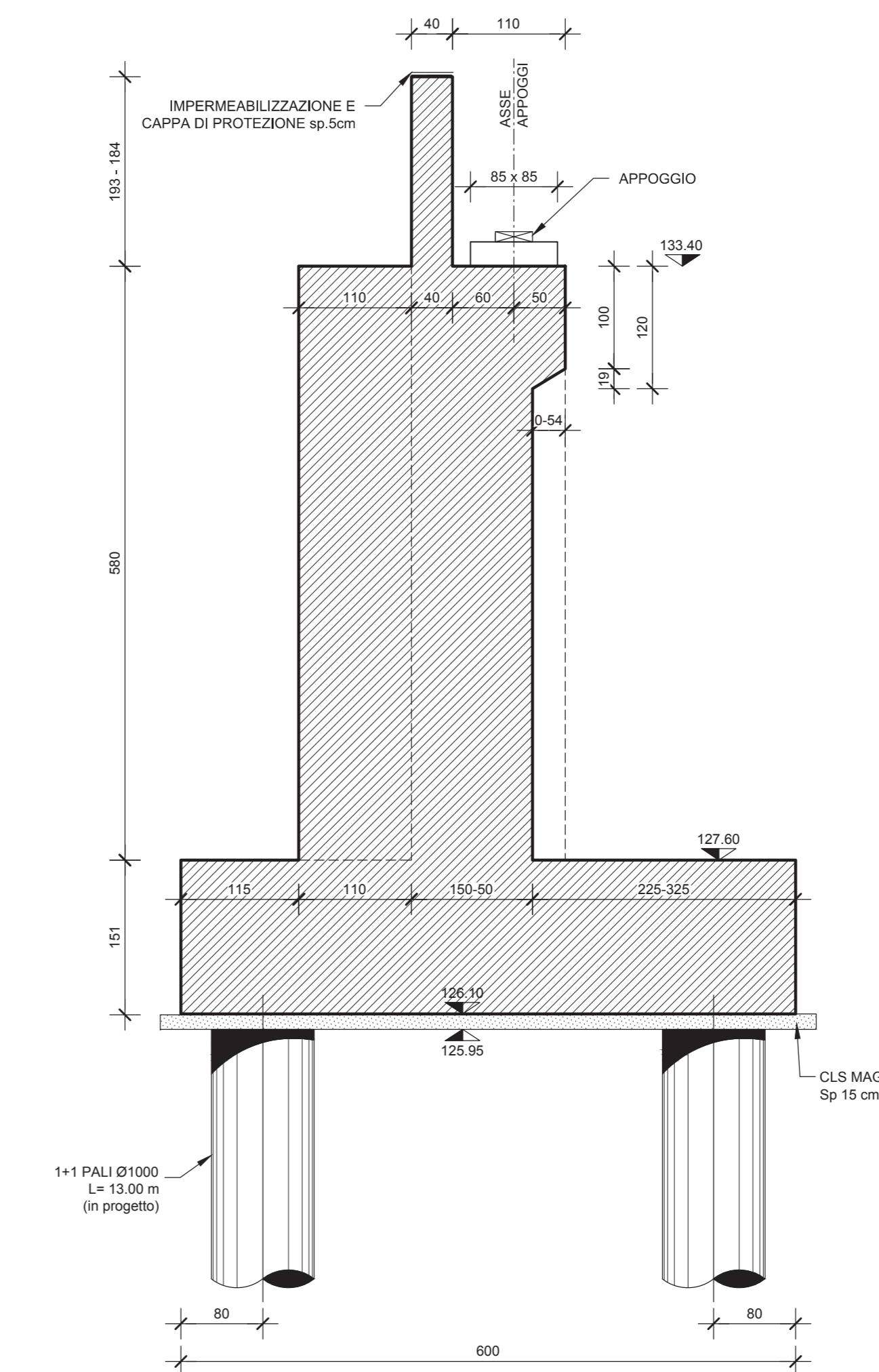
SEZIONE TRASVERSALE ALLARGAMENTO Scala 1:50
