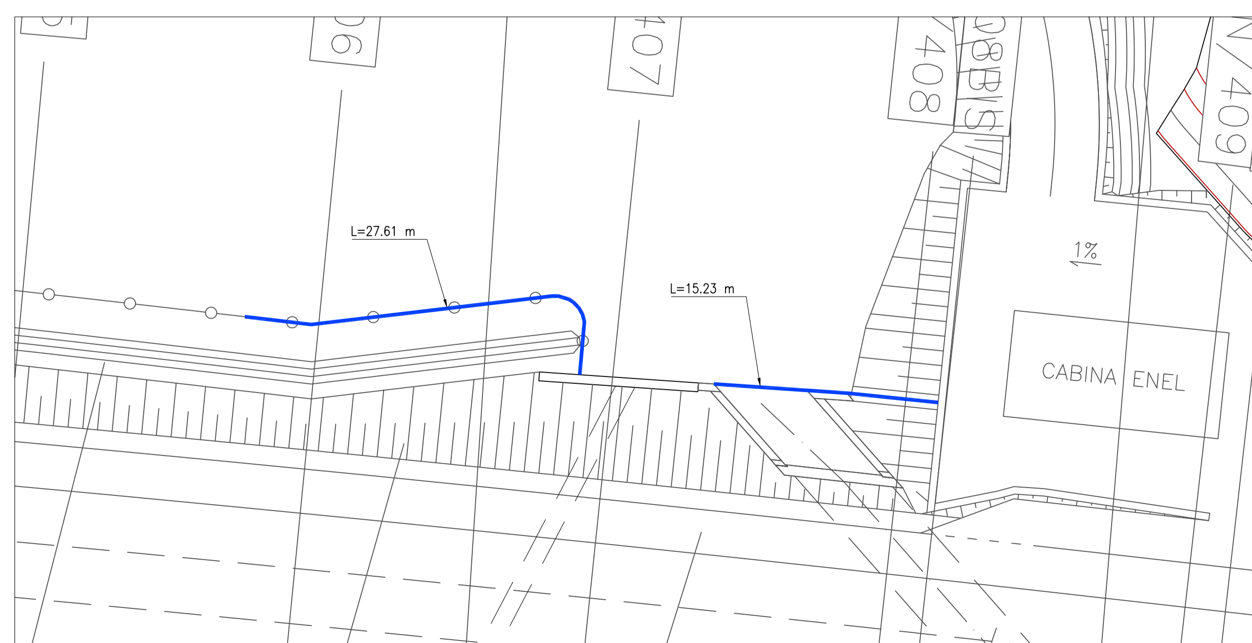
OPERE DI MITIGAZIONE AMBIENTALE TOMBINO D=1,20 m (Opera 50) Progr. km 222+129 Scala 1:250
