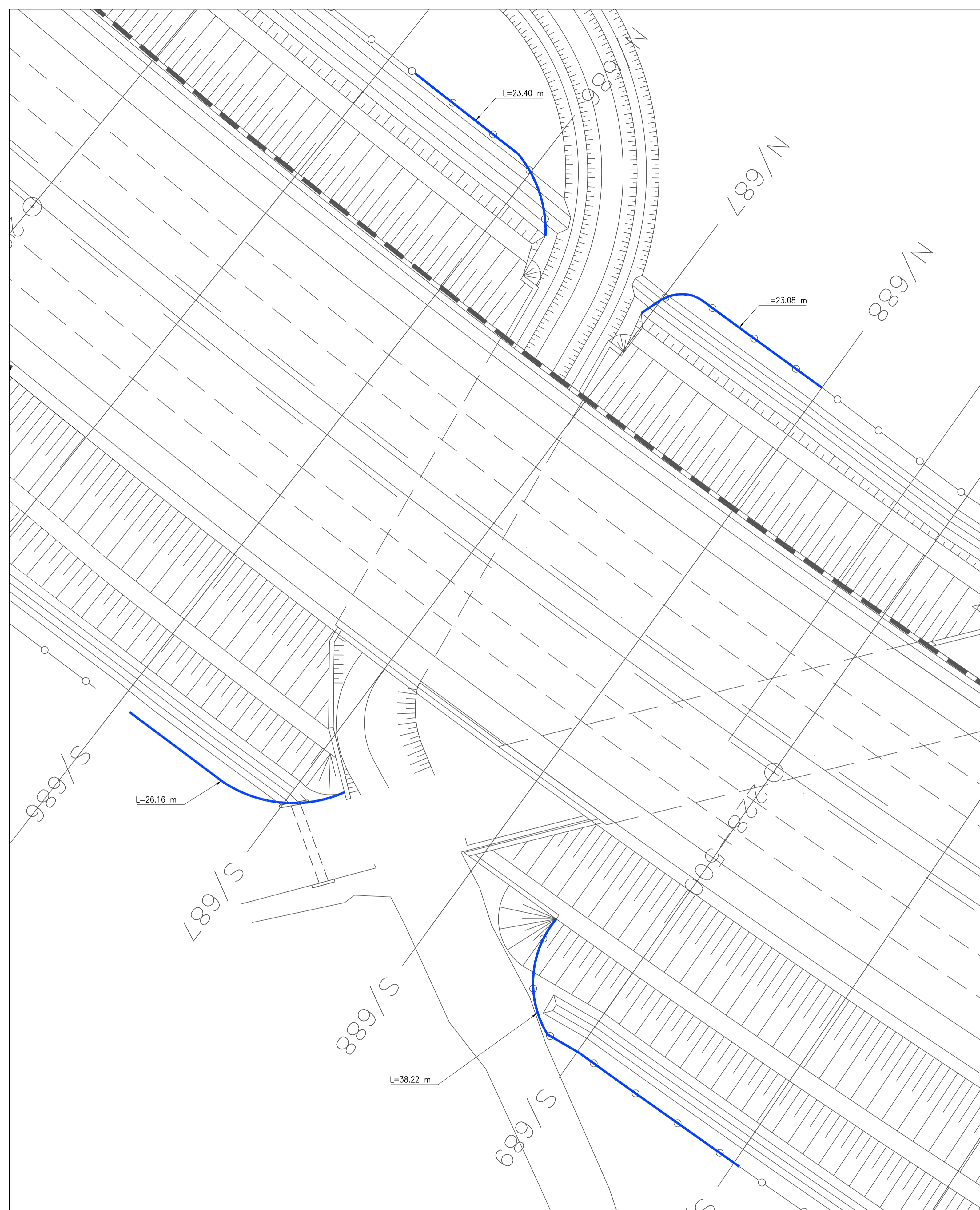
OPERE DI MITIGAZIONE AMBIENTALE TOMBINO D=1,20 m (Opera 50) Progr. km 222+129 Scala 1:250
