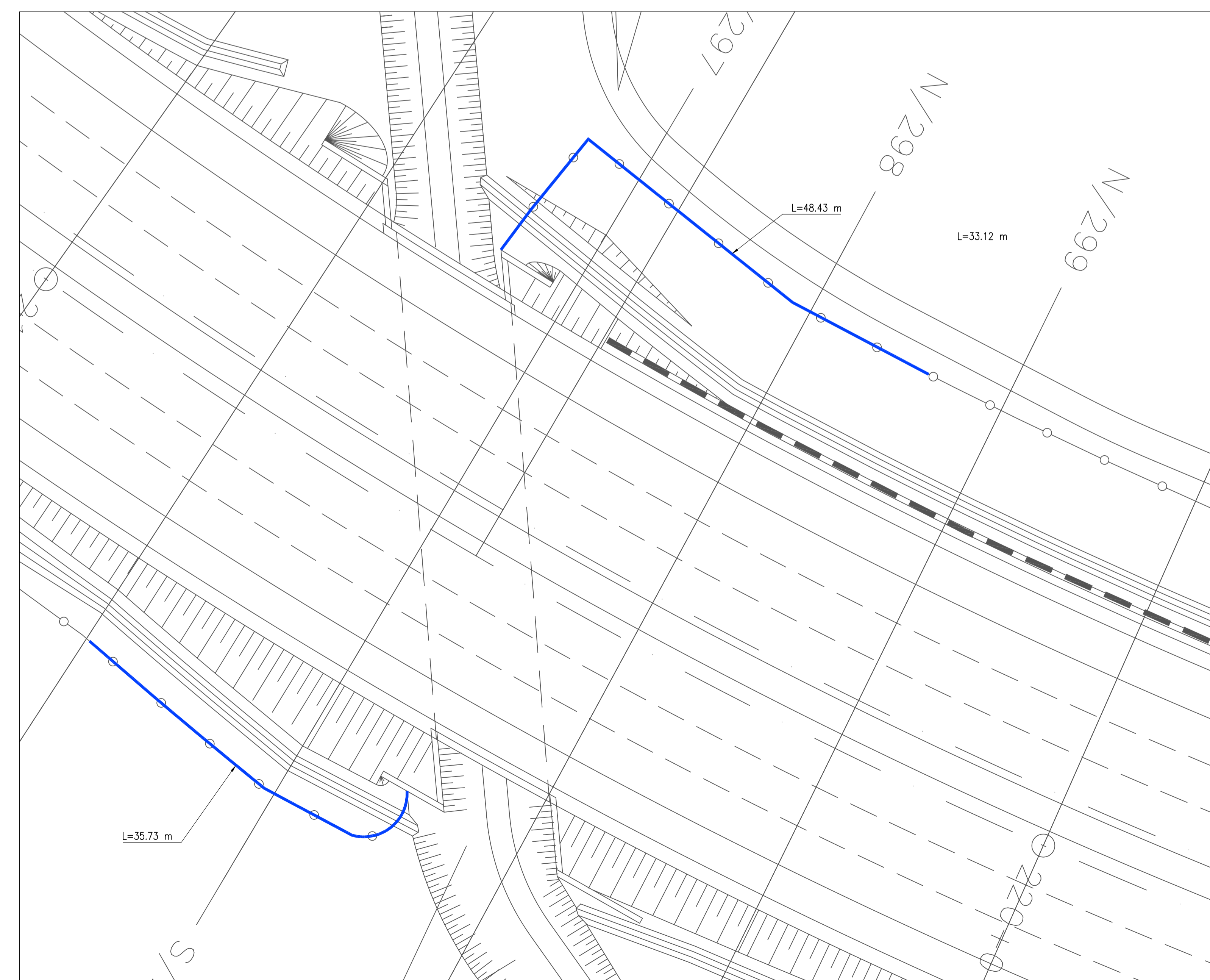
OPERE DI MITIGAZIONE AMBIENTALE PONTICELLO L=9,50 m (Opera 33) Progr. km 219+944 Scala 1:250
