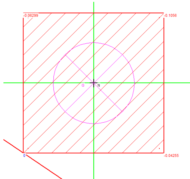
Fig. 63 – Verifica SLU - pressioni sul terreno - combinazione FZ min
