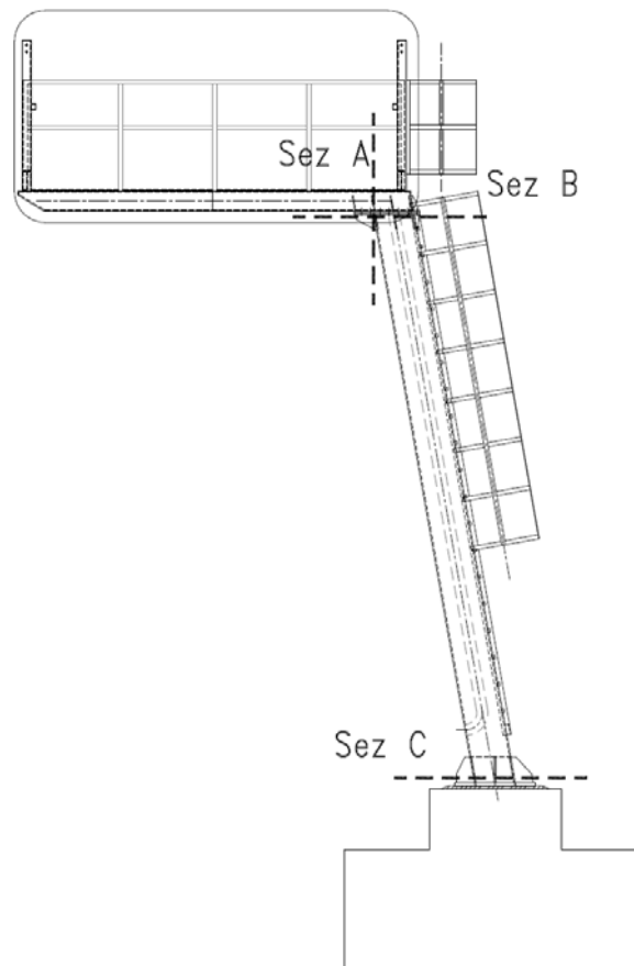
Fig. 41 – Sezioni di verifica
