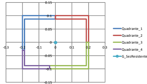
Geometria della sezione resistente
