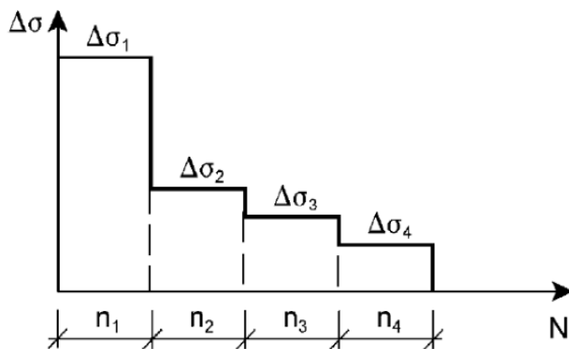
Fig. 53 – Spettro di variazione delle tensioni
