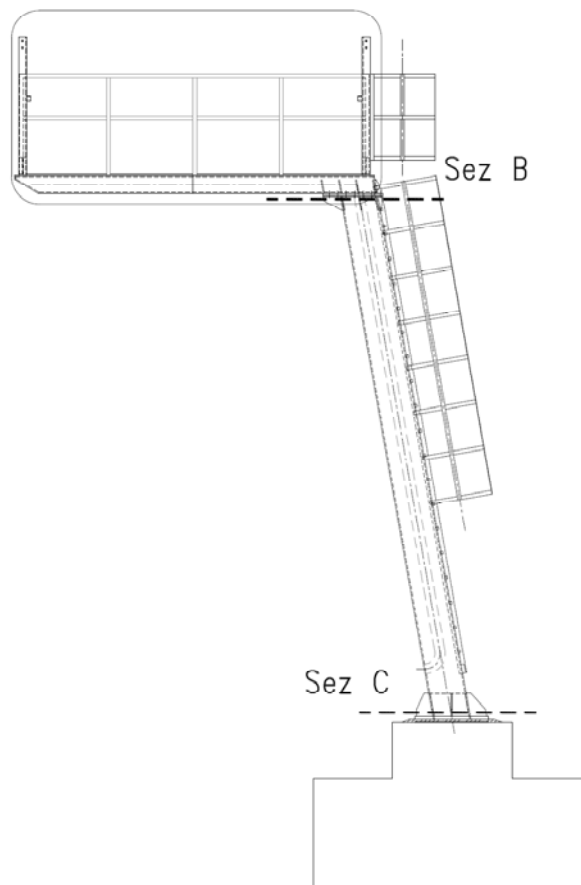
Fig. 44 – Sezioni di verifica - giunzioni bullonate
