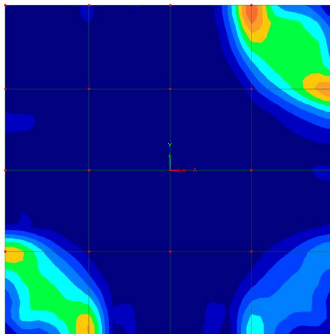
Fig. 51 – Mappatura tensionale
