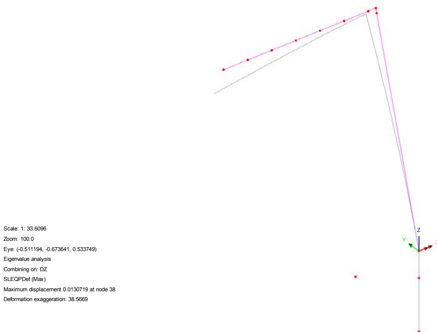
Fig. 39 – Spostamenti verticali massimi
