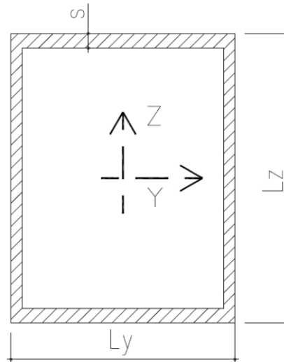
Fig. 42 – Geometria delle sezioni di verifica
