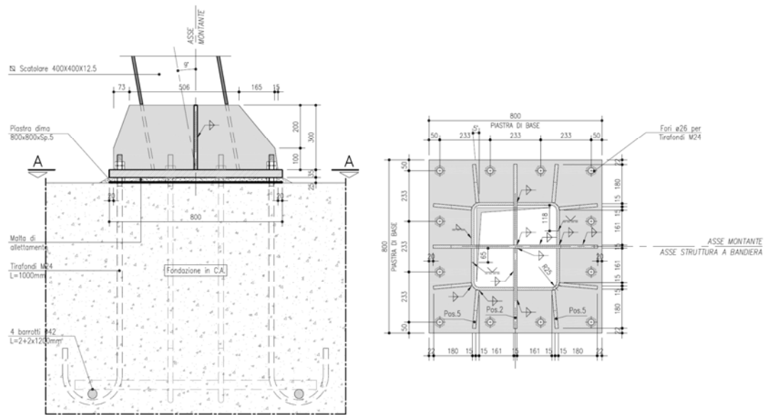
Fig. 3 – Dettaglio della connessione alla base quadrata
