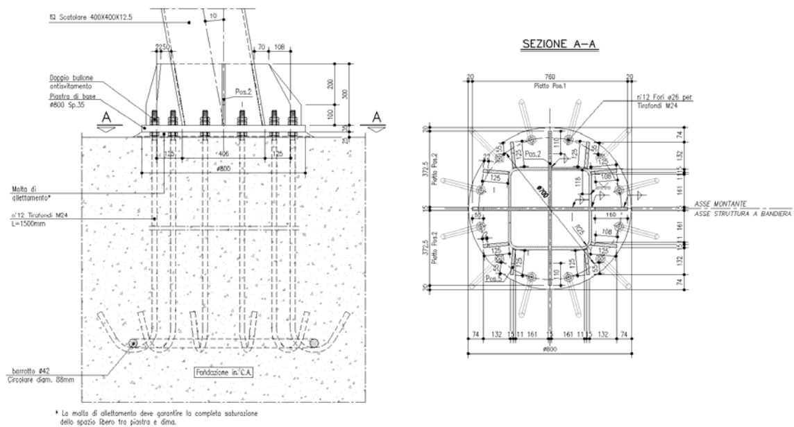
Fig. 4 – Dettaglio della connessione alla base circolare
