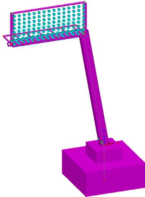
Fig. 11 – Azione di Buffeting - Corsia 1
