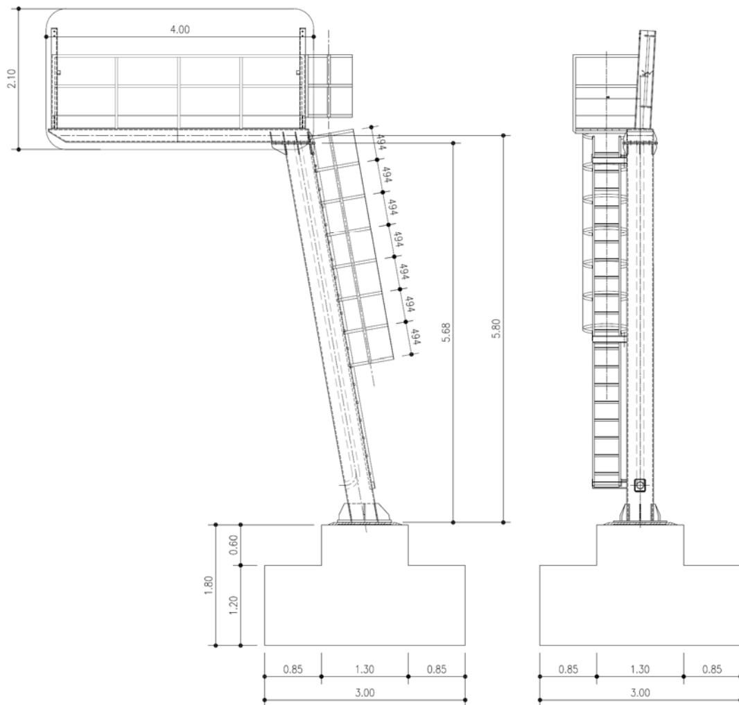
Fig. 2 – Vista frontale e laterale del portale
