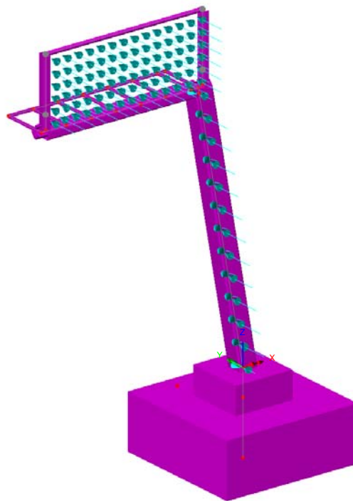
Fig. 7 – Azioni del vento sulla struttura
