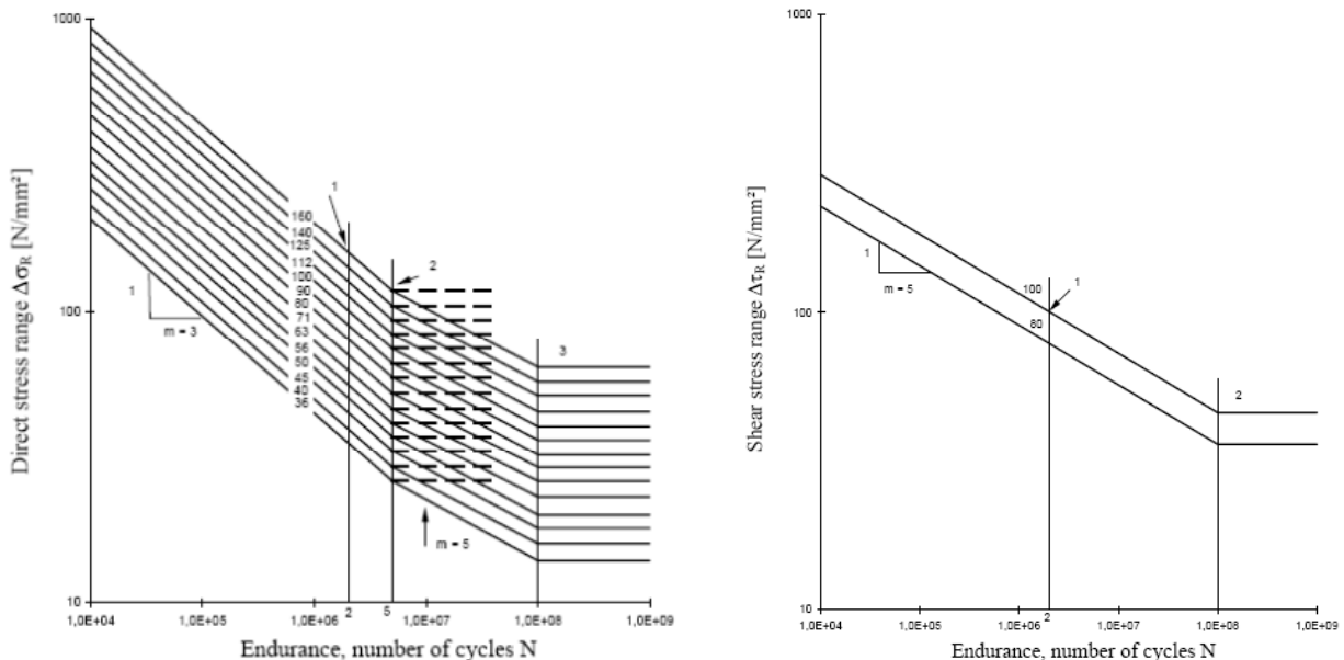
Fig. 54 – Curve di resistenza a fatica S-N per tensioni normali e tangenziali
