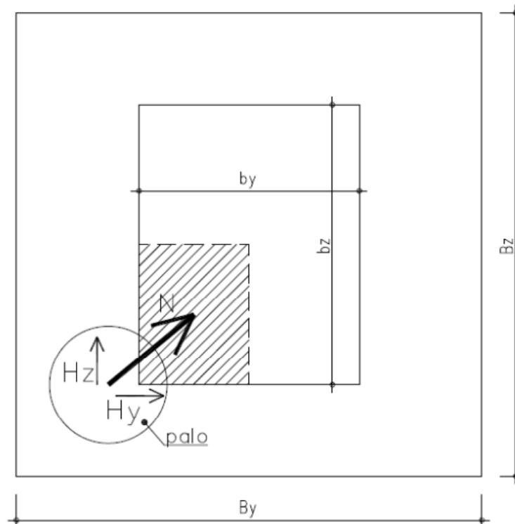
Fig. 65 – Individuazione qualitativa in pianta del puntone
