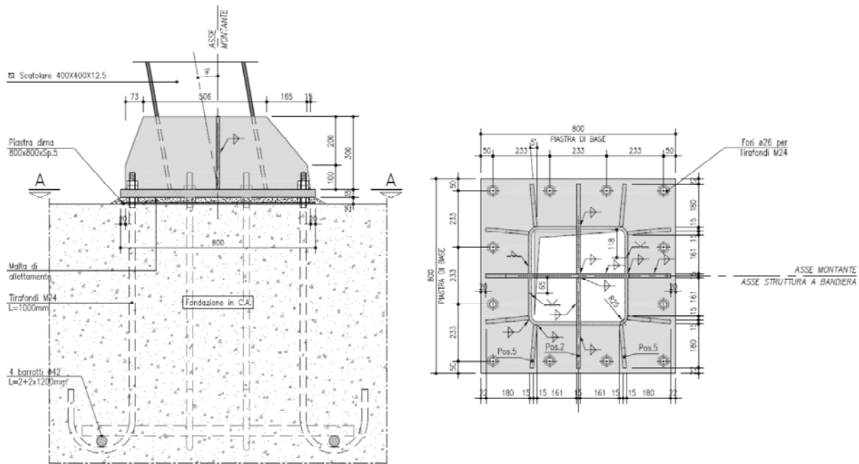
Fig. 52 – Giunto di base - Sez C
