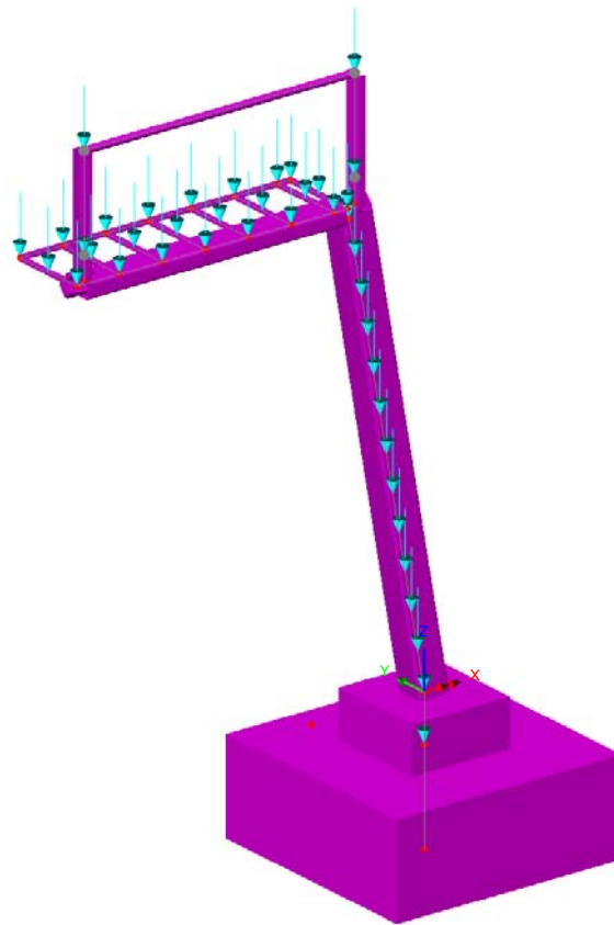
Fig. 6 – Pesì permanenti portati
