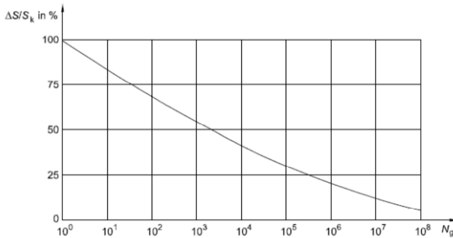
Fig. 56 – Numero di cicli di carico da raffica per un effetto \Delta S/S_k
