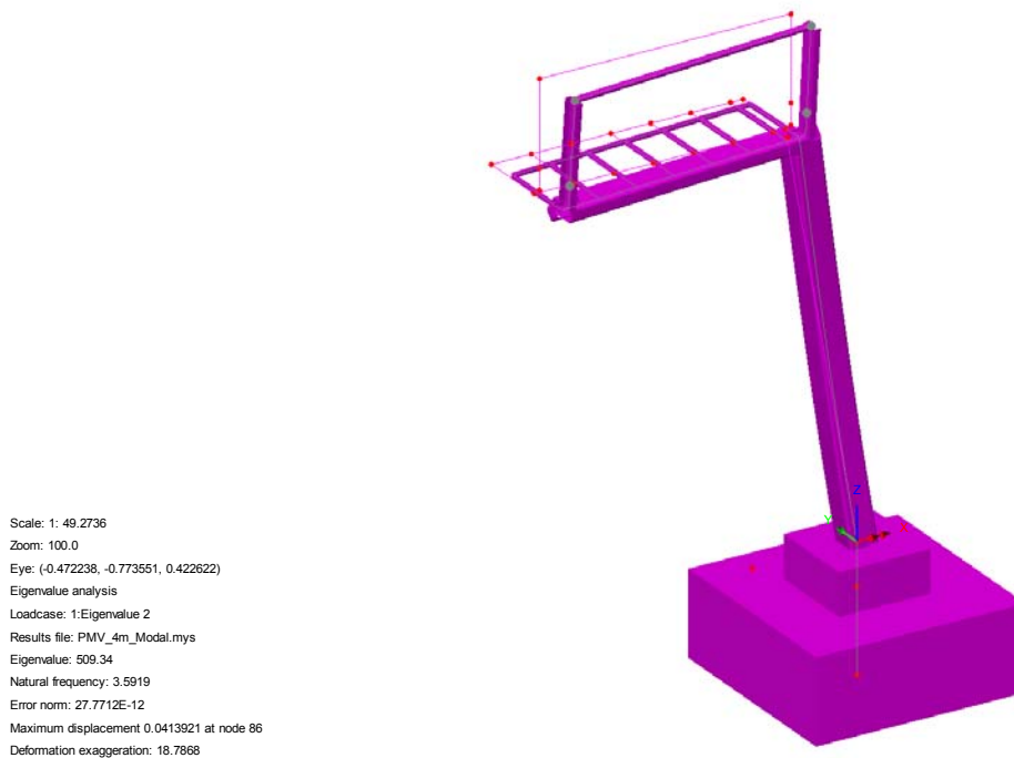
Fig. 8 – Analisi modale della struttura
