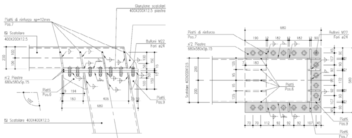
Fig. 45 – Giunto bullonato - Sez B
