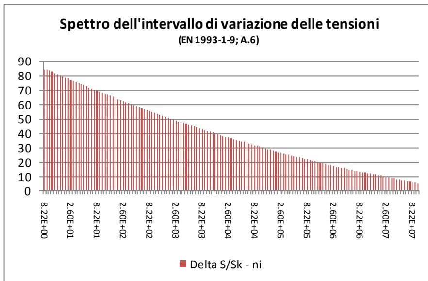
Fig. 57 – Numero di cicli di carico da raffica (cumulata) per un effetto \Delta S/S_k
