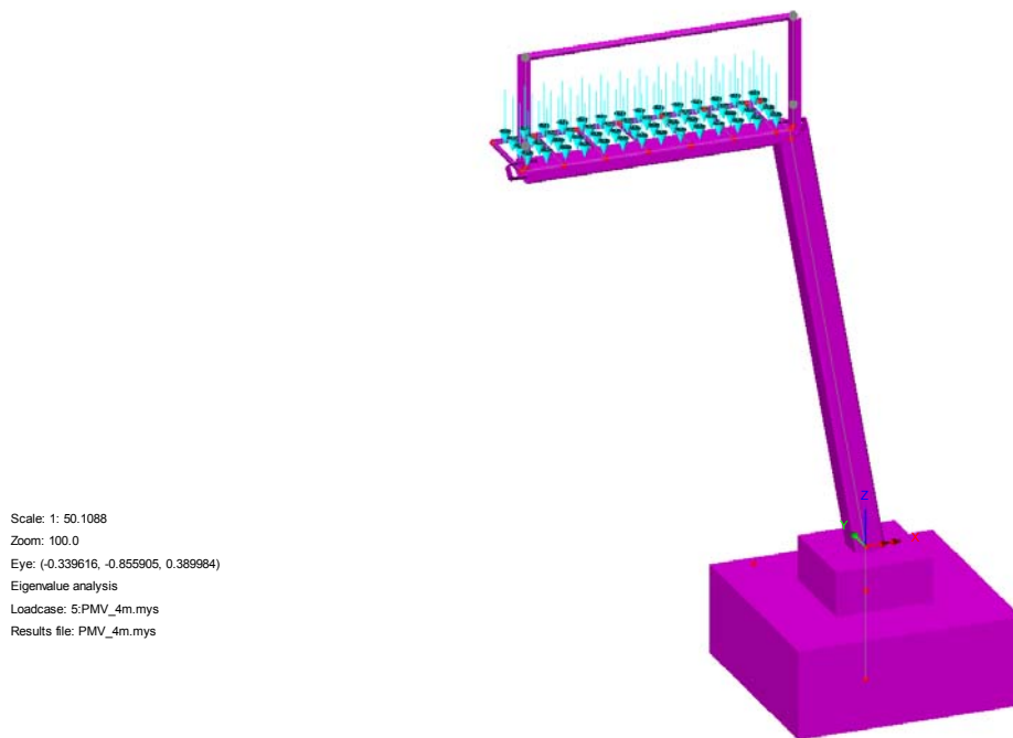
Fig. 12 – Carico da neve
