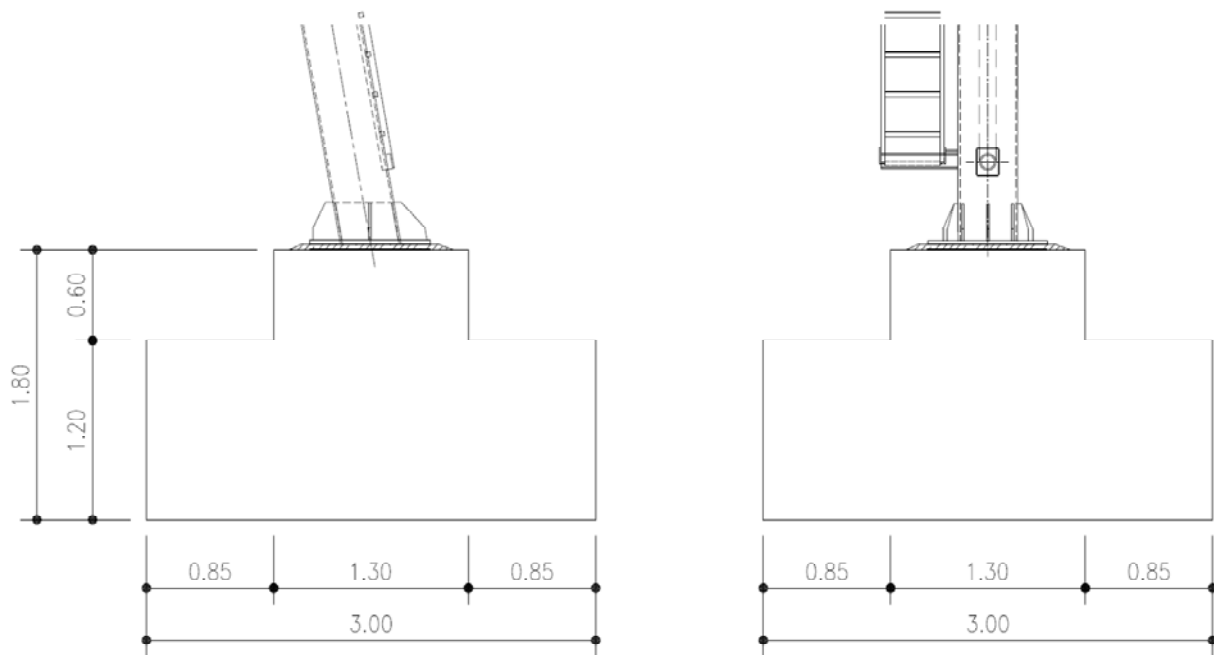
Fig. 58 – Sezioni del plinto di fondazione
