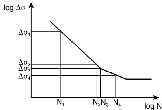
Fig. 55 – Determinazione del numero di cicli a rottura per \Delta\sigma assegnato
