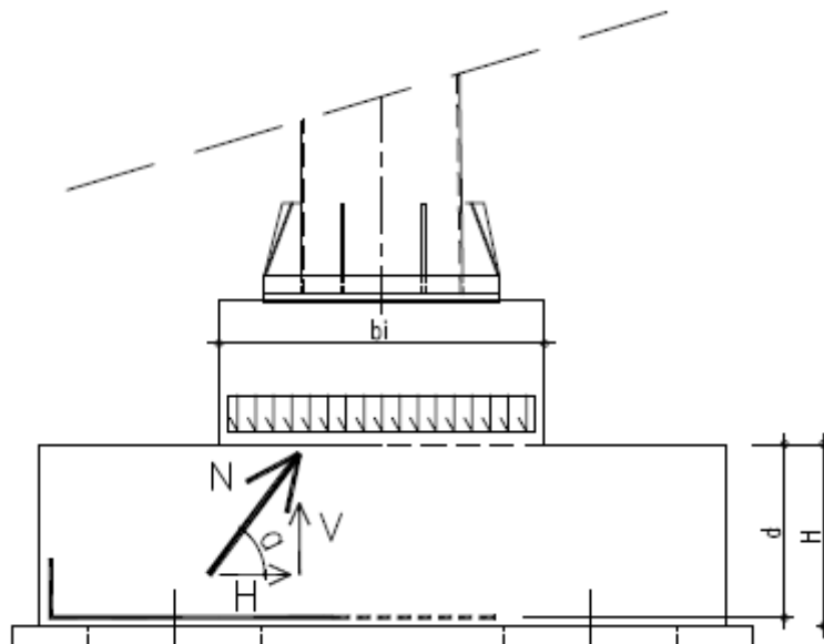
Fig. 64 – Meccanismo resistente a Tirante-puntone
