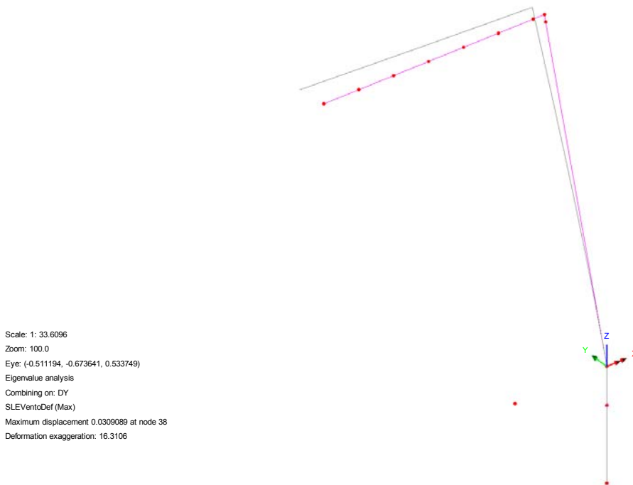
Fig. 40 – Spostamenti orizzontali massimi
