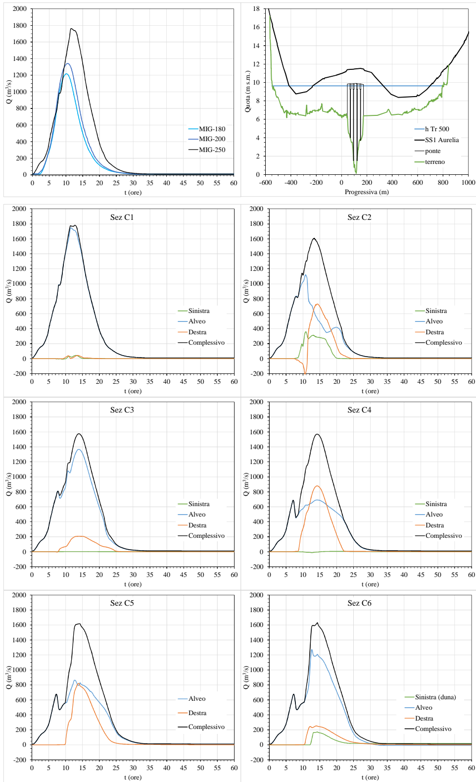
Figura A3.58. Portate e livelli a monte e portate a valle della SS1 Aurelia ( afusTr500M )
