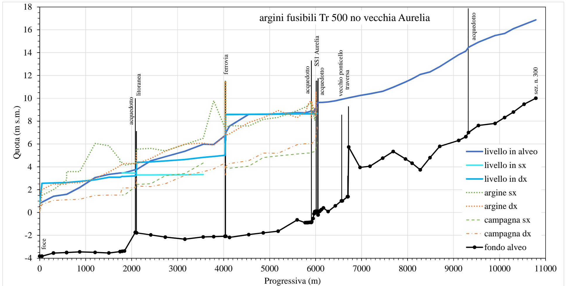
Figura A3.59. Massimi profili idrici ( afusTr500N )
