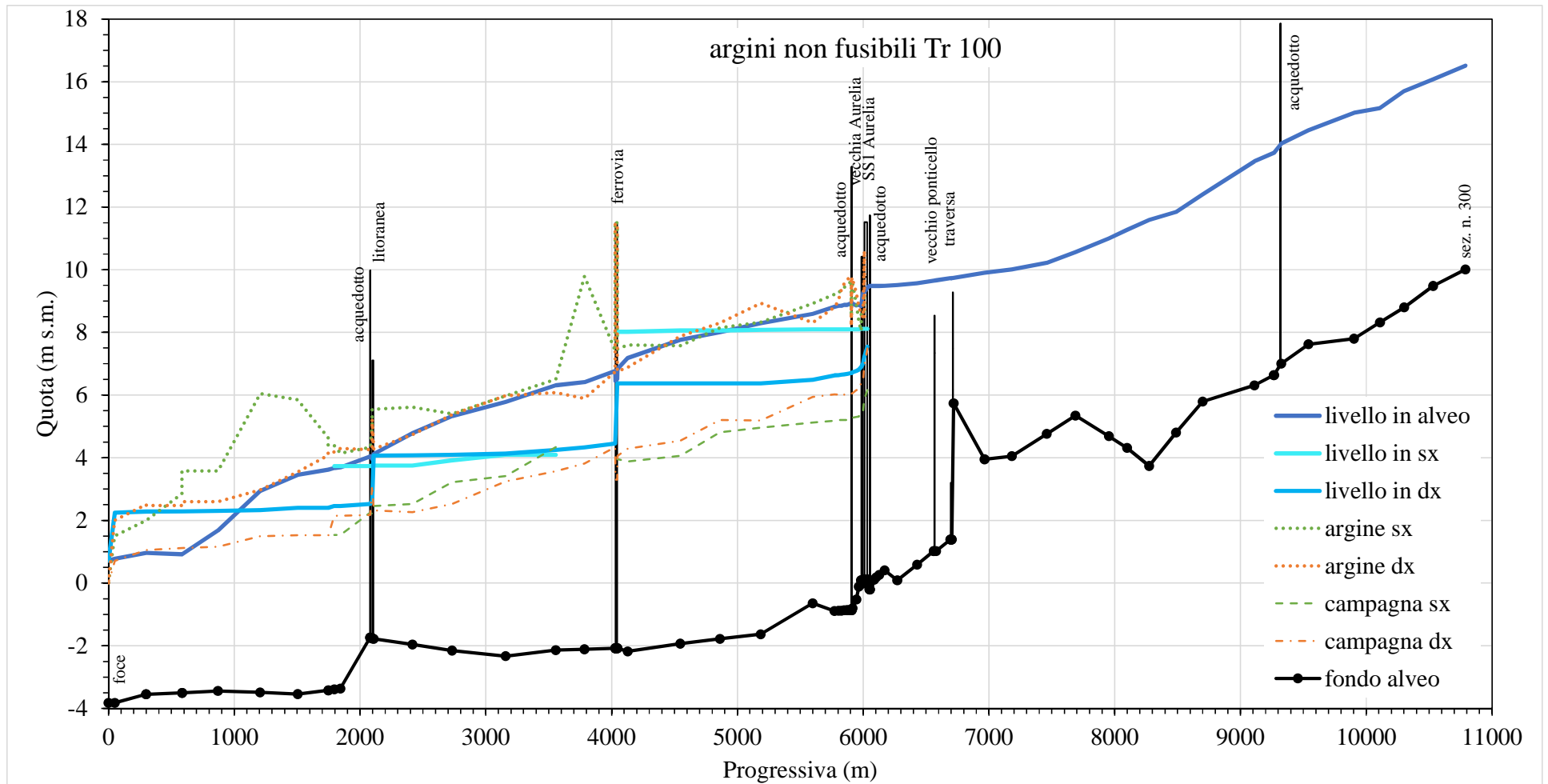
Figura A3.23. Massimi profili idrici ( anofusTr100 )
