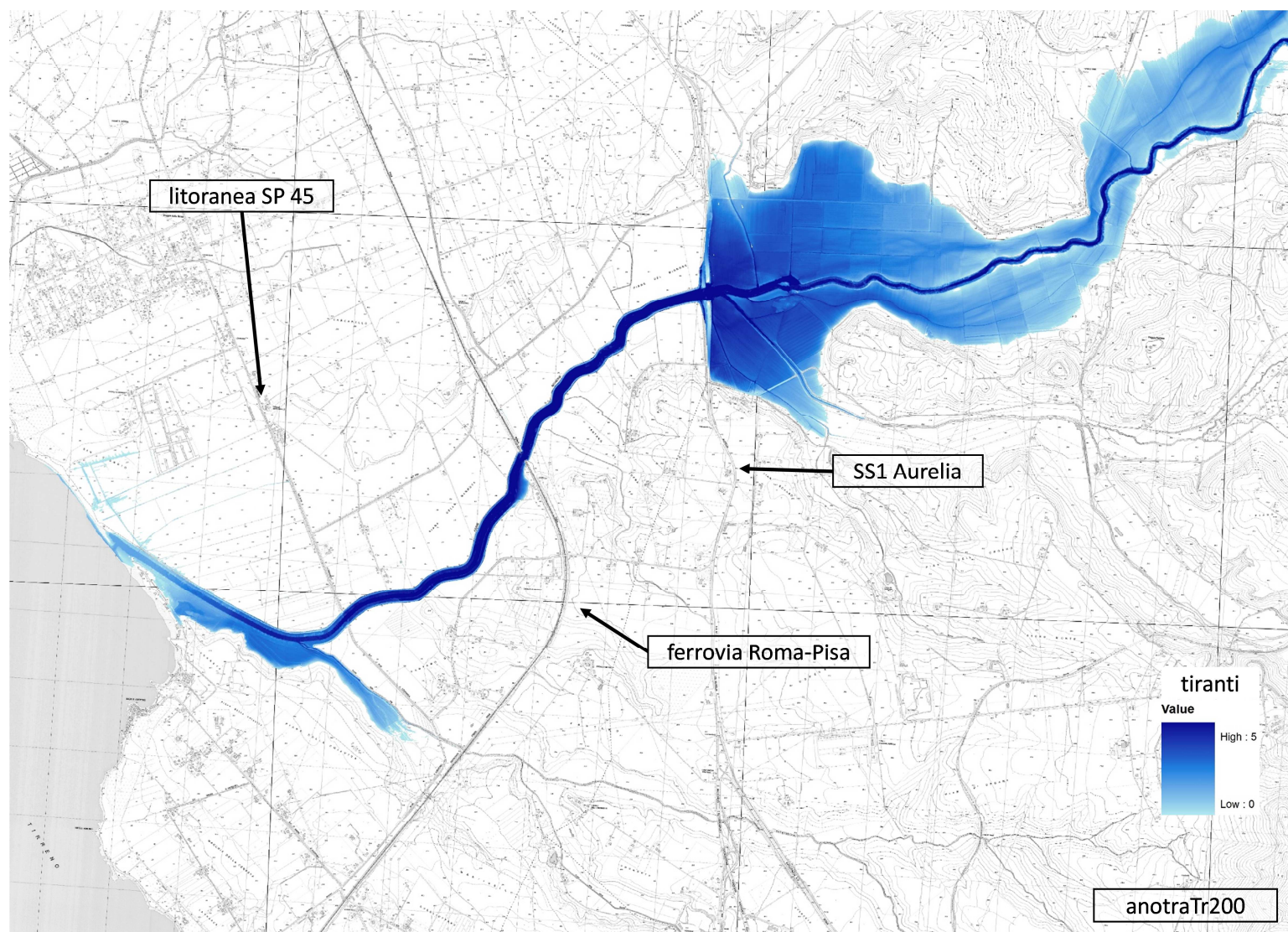
Figura A3.42. Aree inondabili e tiranti idrici ( anotraTr200 )
