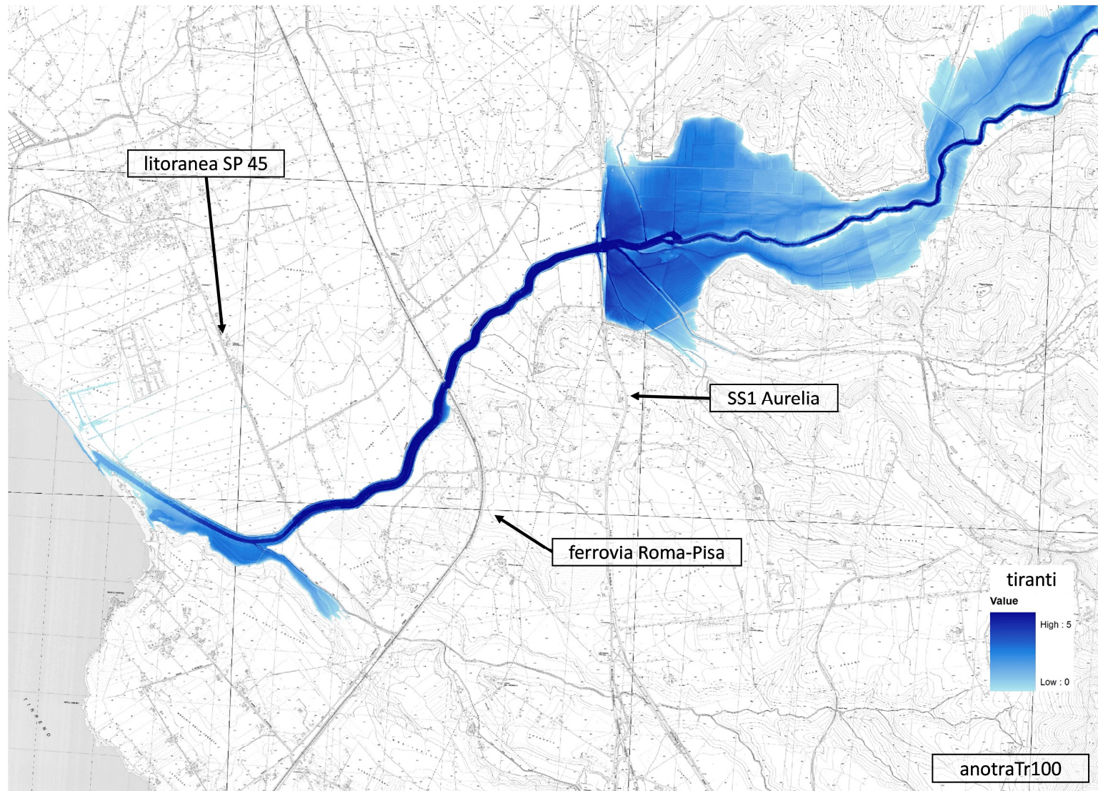
Figura A3.39. Aree inondabili e tiranti idrici ( anotraTr100 )
