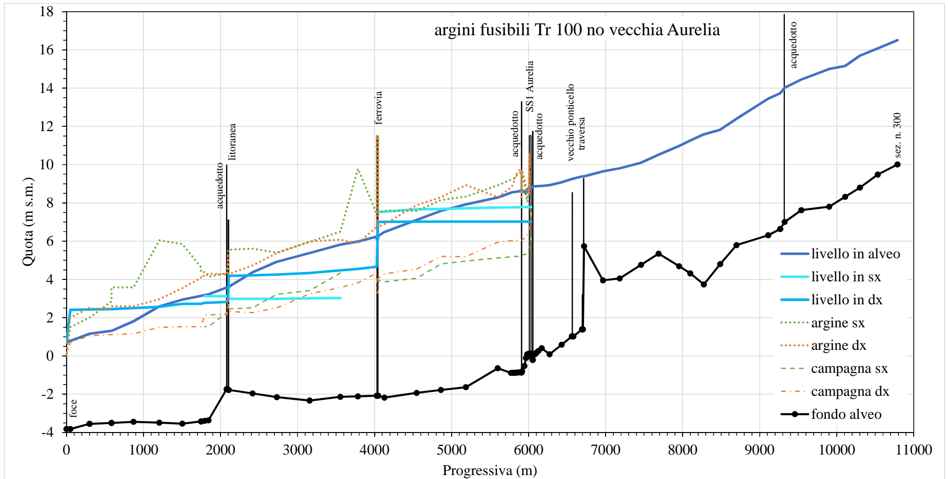
Figura A3.53. Massimi profili idrici ( afusTr100N )
