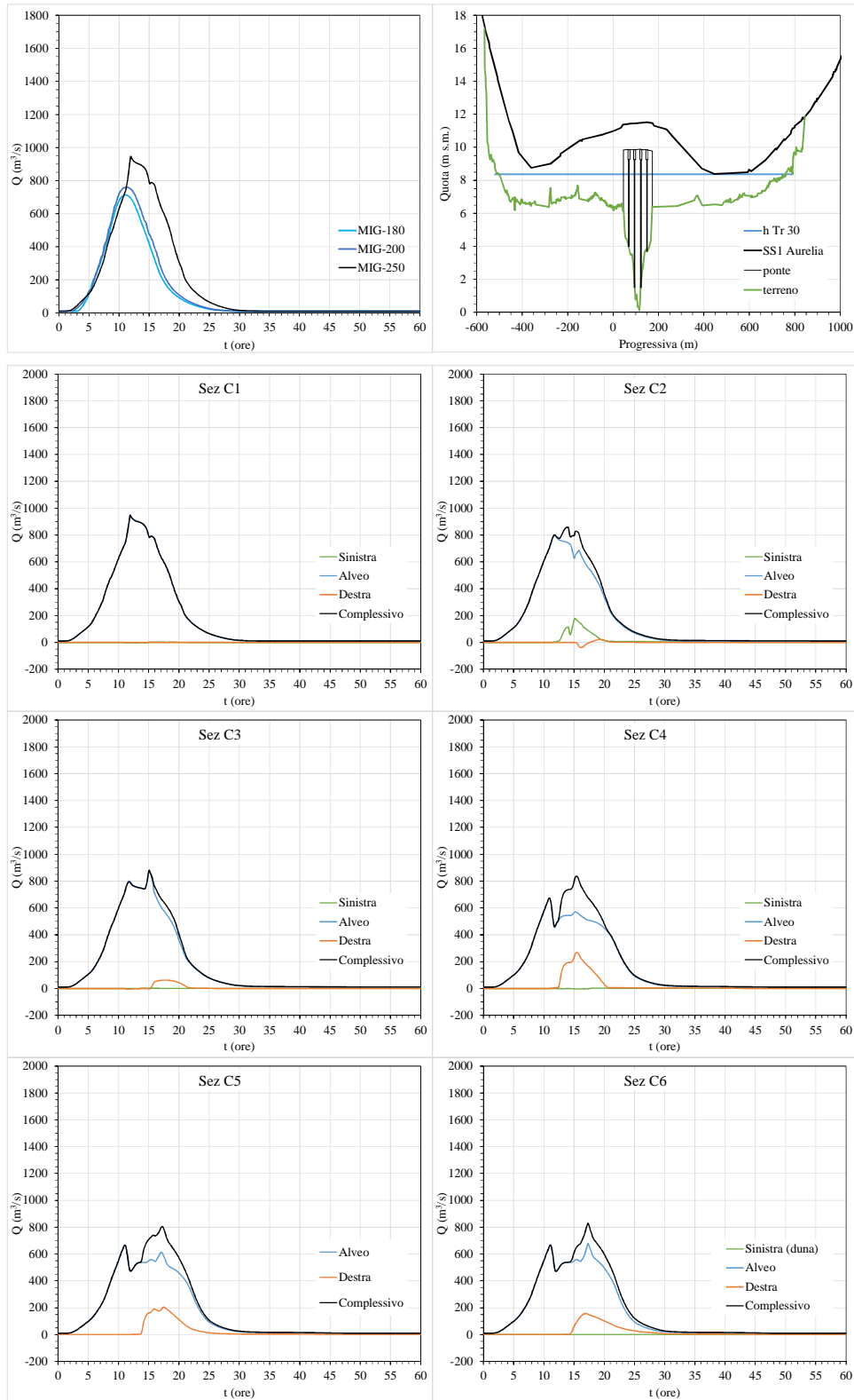
Figura A3.46. Portate e livelli a monte e portate a valle della SS1 Aurelia ( afusTr030N )
