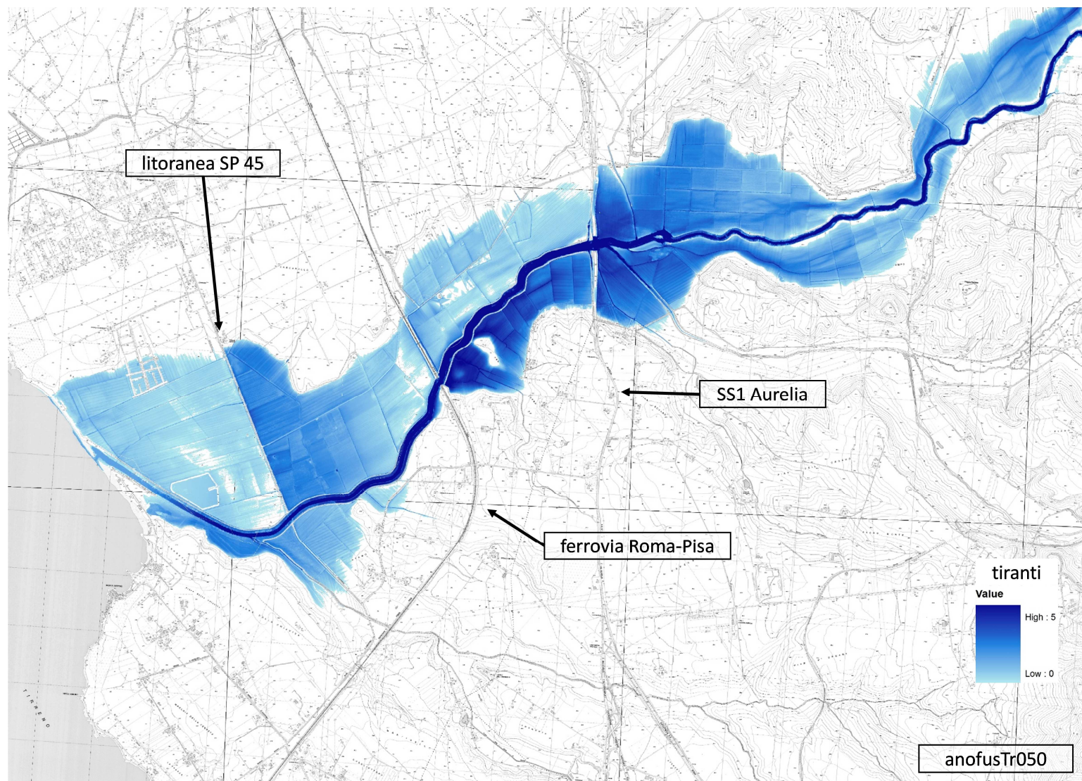
Figura A3.21. Aree inondabili e tiranti idrici ( anofusTr050 )
