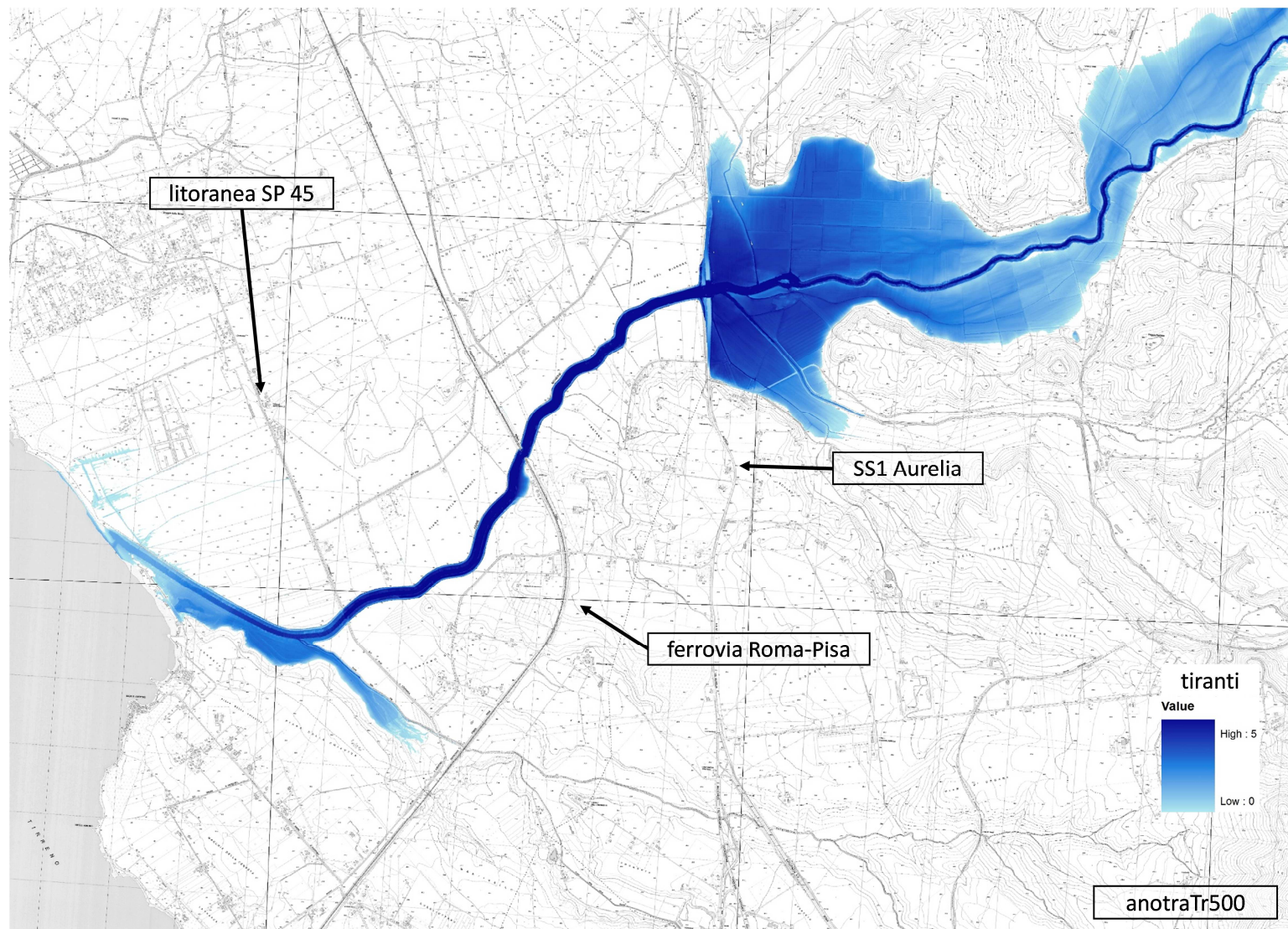
Figura A3.45. Aree inondabili e tiranti idrici ( anotraTr500 )
