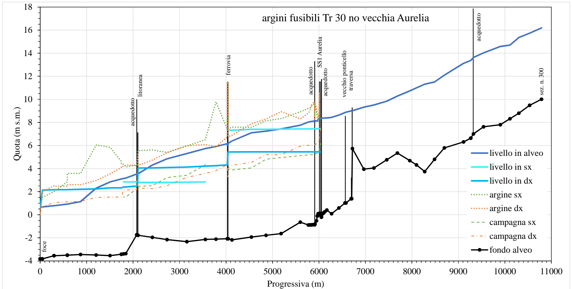
Figura A3.47. Massimi profili idrici ( afusTr030N )
