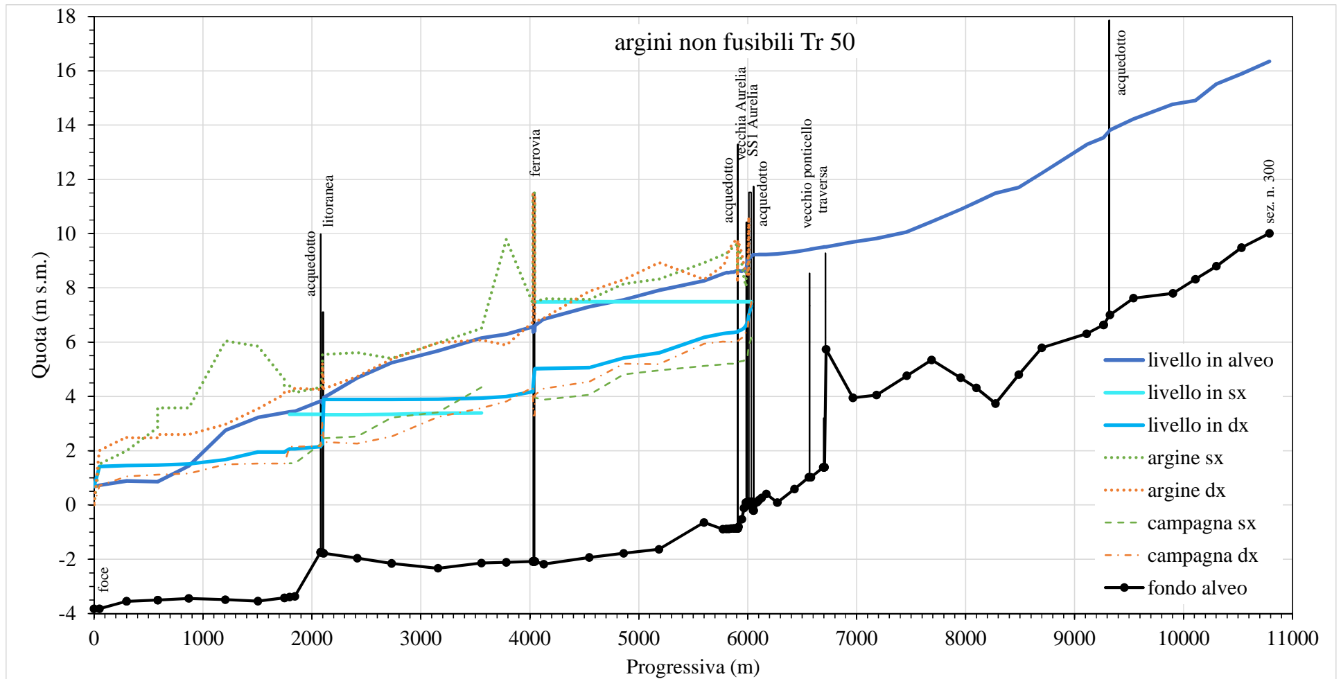
Figura A3.20. Massimi profili idrici ( anofusTr050 )
