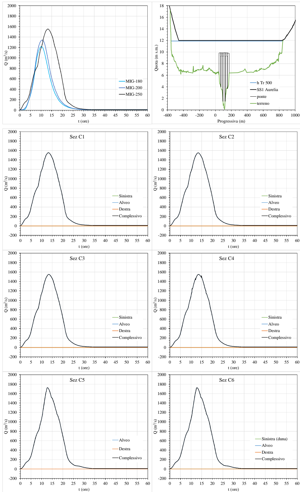
Figura A3.43. Portate e livelli a monte e portate a valle della SS1 Aurelia ( anotraTr500 )
