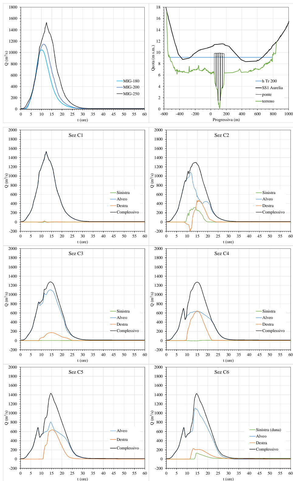
Figura A3.55. Portate e livelli a monte e portate a valle della SS1 Aurelia ( afusTr200M )
