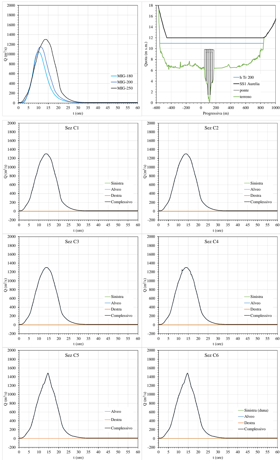
Figura A3.40. Portate e livelli a monte e portate a valle della SS1 Aurelia ( anotraTr200 )
