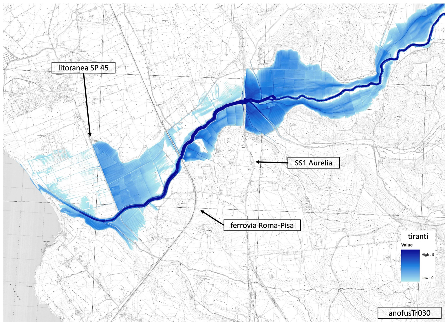
Figura A3.18. Aree inondabili e tiranti idrici ( anofusTr030 )
