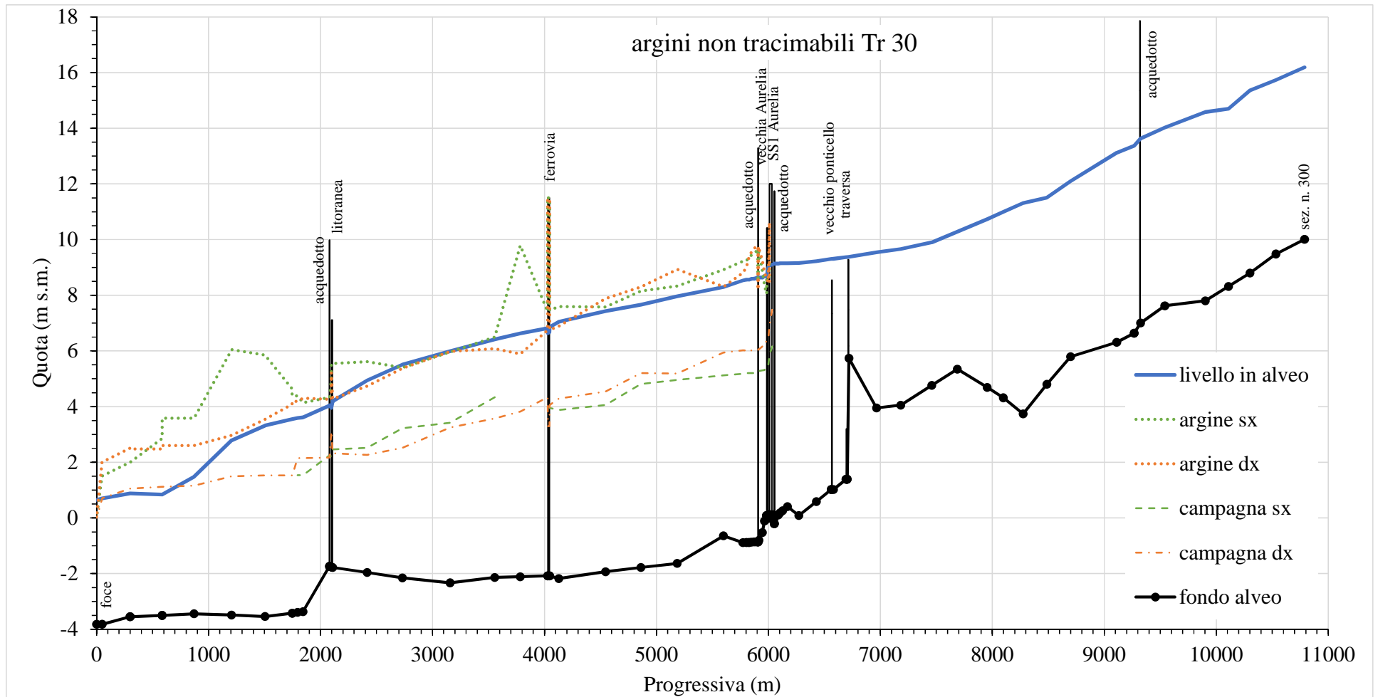
Figura A3.32. Massimi profili idrici ( anotraTr030 )
