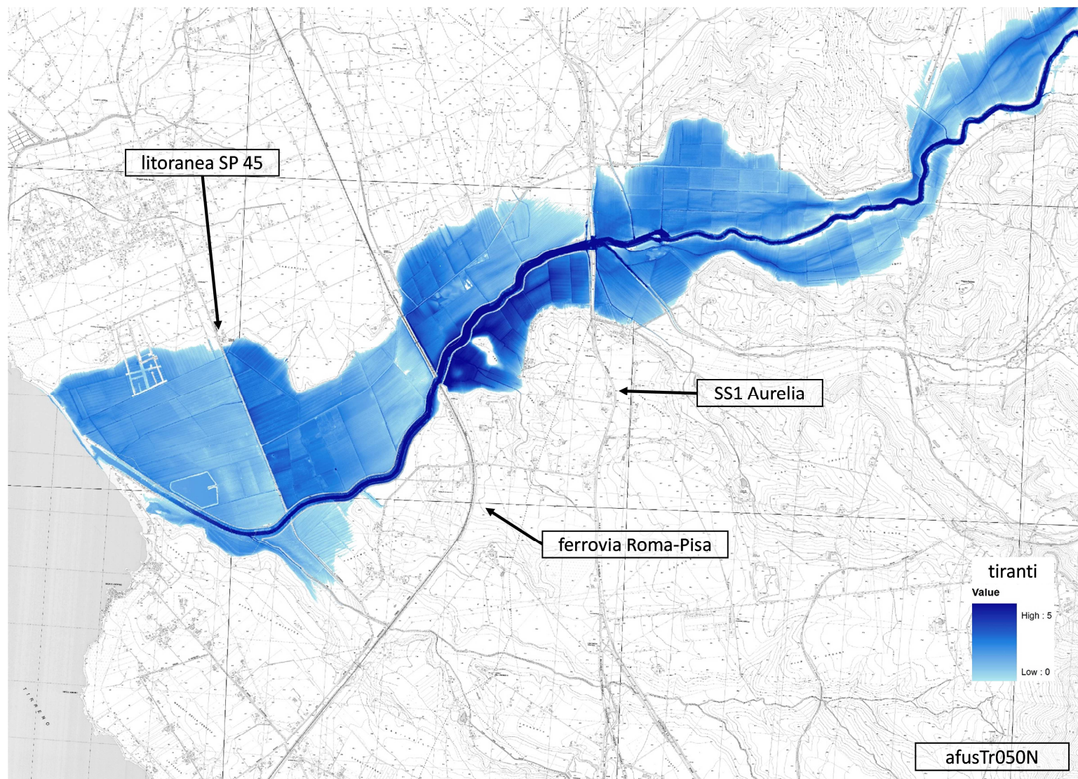
Figura A3.51. Aree inondabili e tiranti idrici ( afusTr050N )
