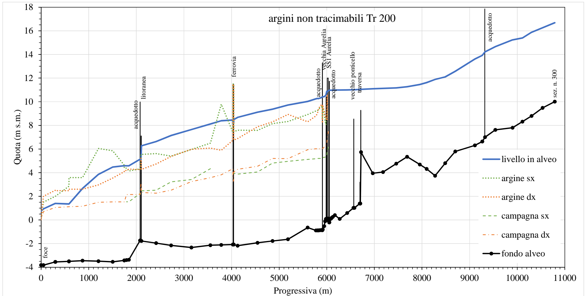
Figura A3.41. Massimi profili idrici ( anotraTr200 )
