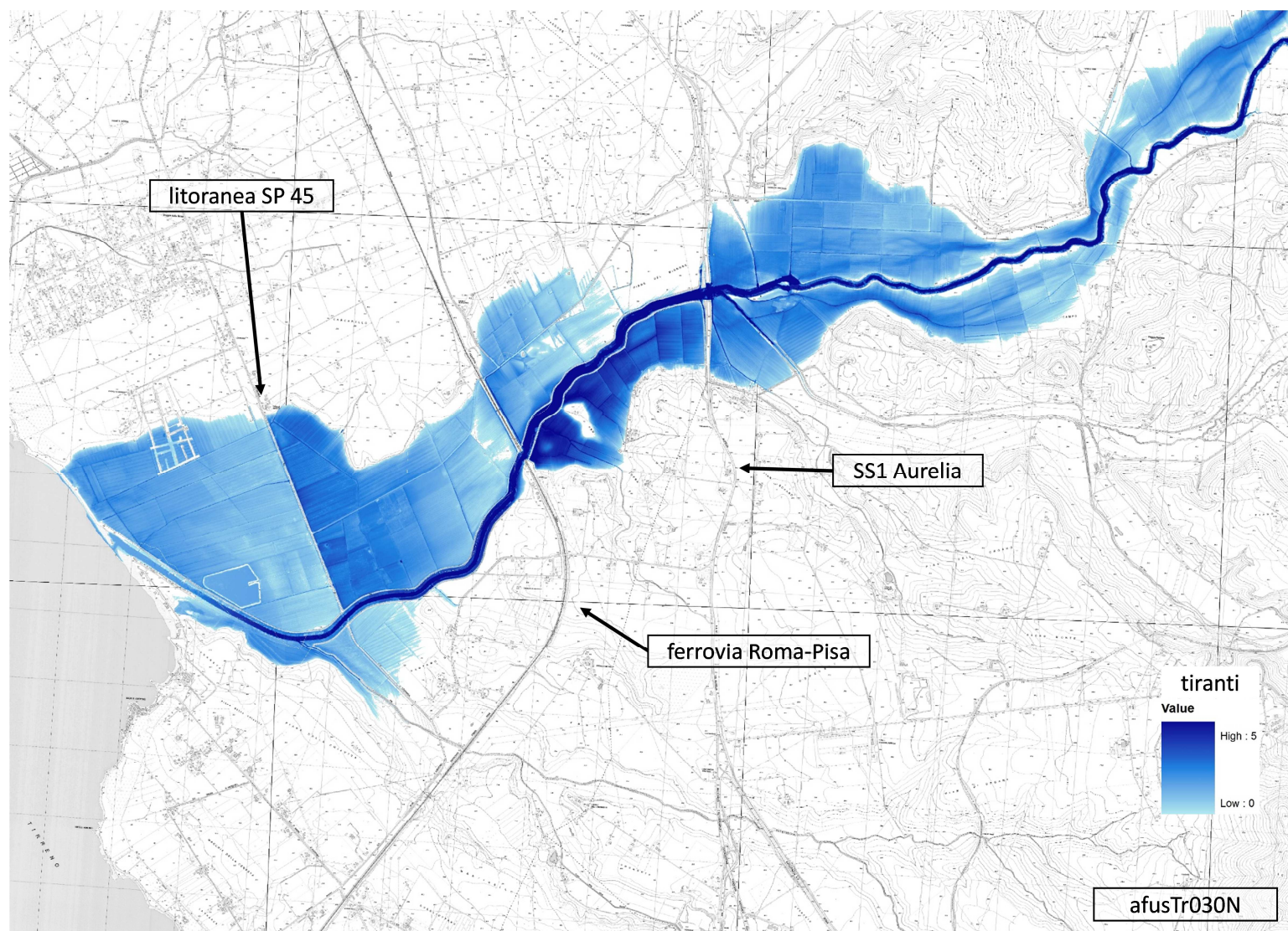
Figura A3.48. Aree inondabili e tiranti idrici ( afusTr030N )
