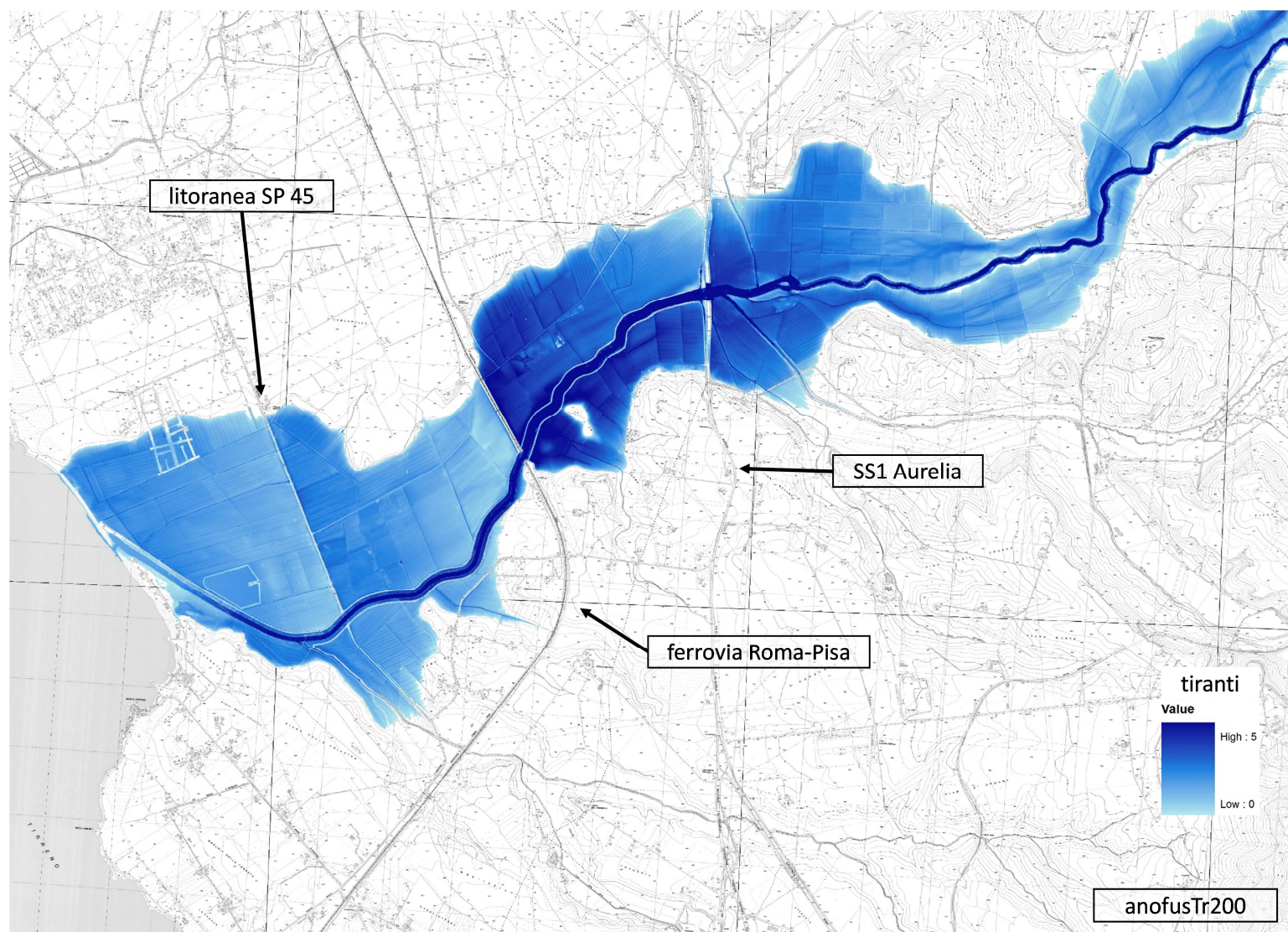
Figura A3.27. Aree inondabili e tiranti idrici ( anofusTr200 )
