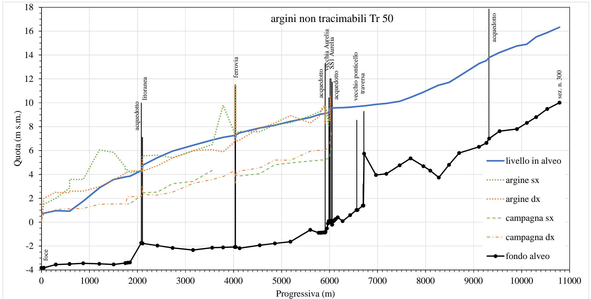
Figura A3.35. Massimi profili idrici ( anotraTr050 )
