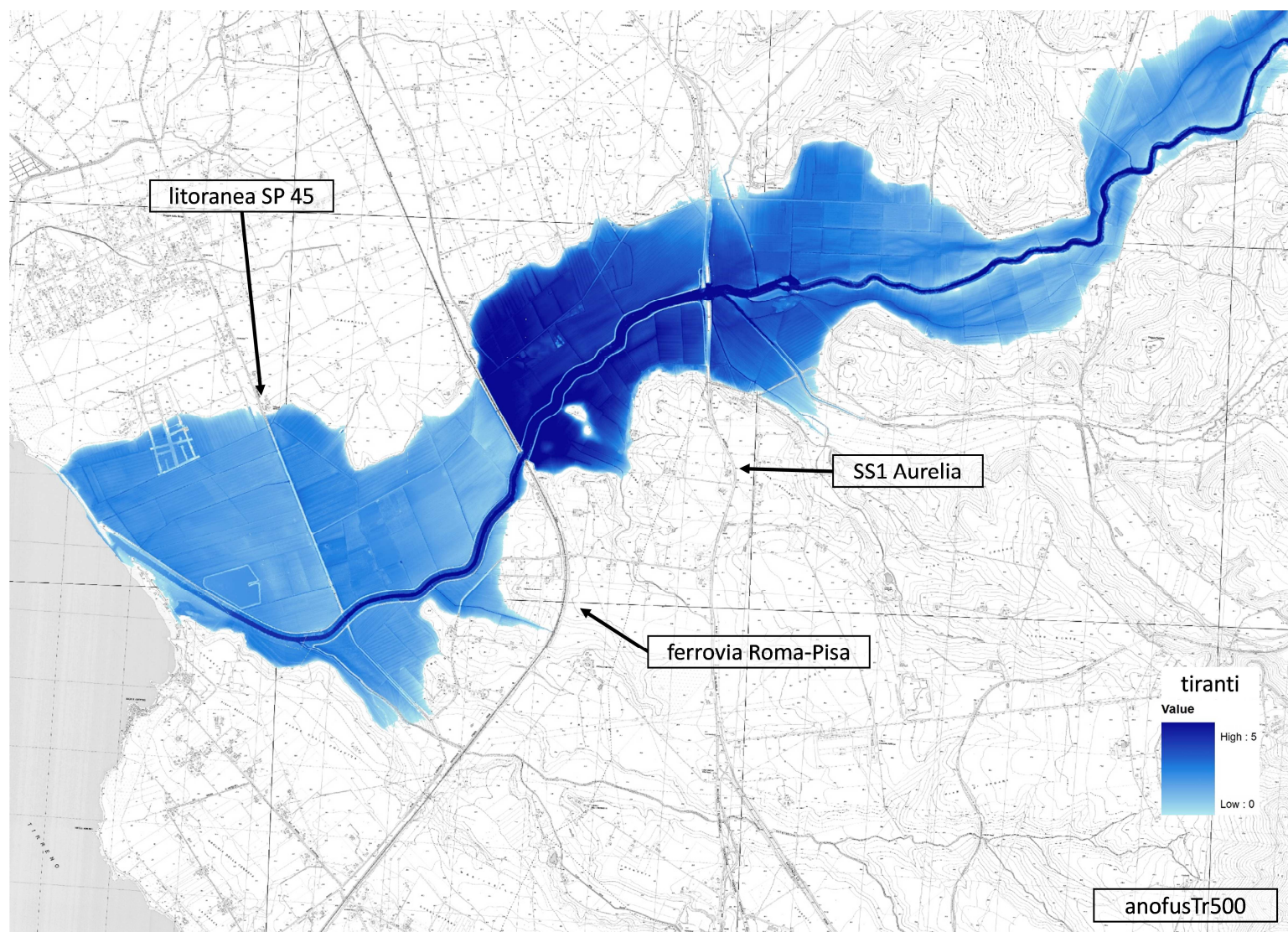
Figura A3.30. Aree inondabili e tiranti idrici ( anofusTr500 )
