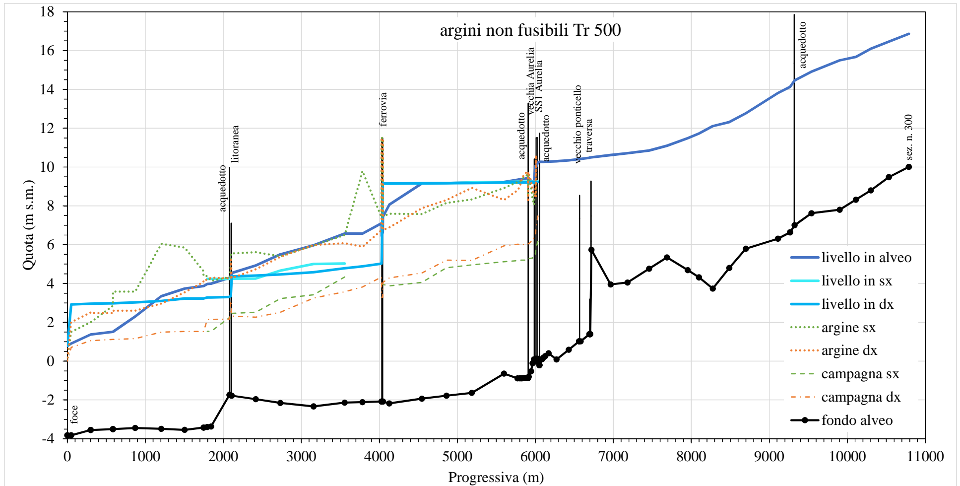
Figura A3.29. Massimi profili idrici ( anofusTr500 )
