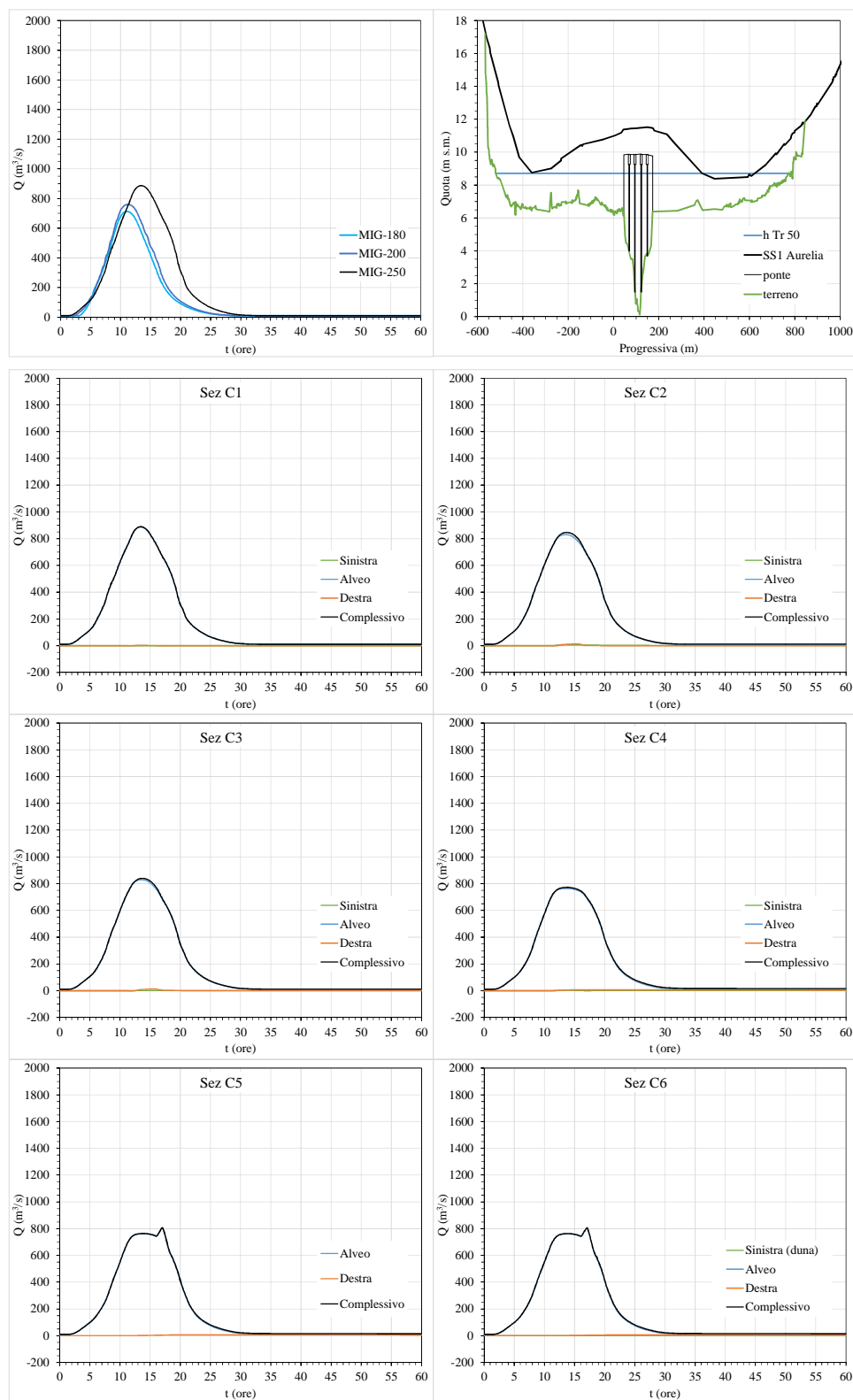
Figura A3.61. Portate e livelli a monte e portate a valle della SS1 Aurelia ( anofusTr030M )
