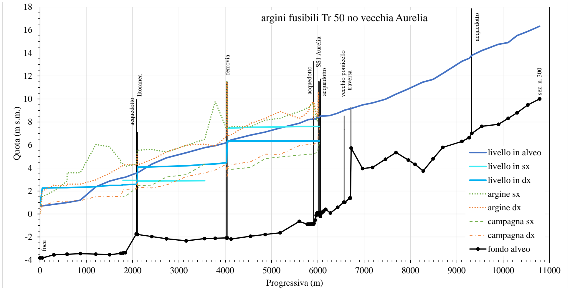
Figura A3.50. Massimi profili idrici ( afusTr050N )
