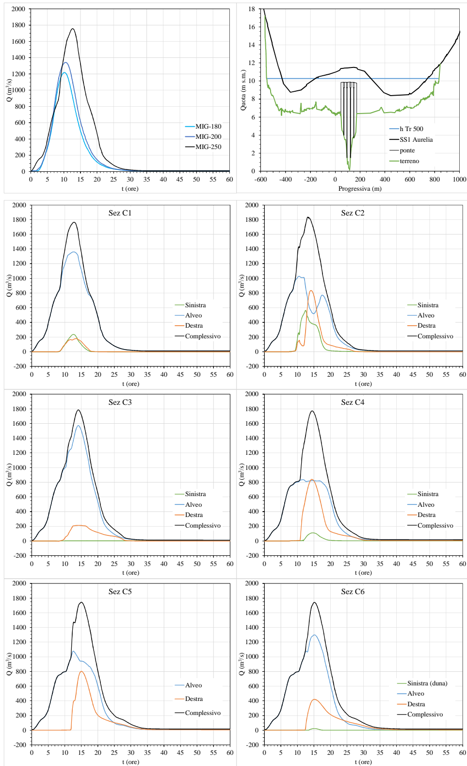
Figura A3.28. Portate e livelli a monte e portate a valle della SS1 Aurelia ( anofusTr500 )
