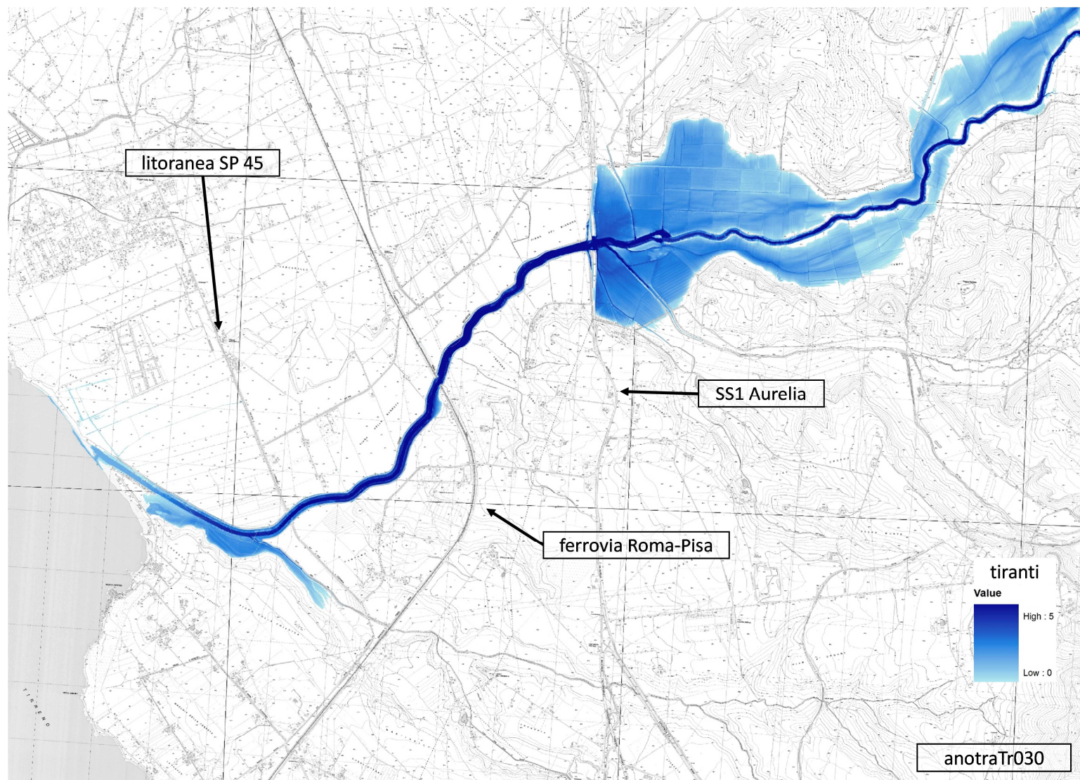
Figura A3.33. Aree inondabili e tiranti idrici ( anotraTr030 )
