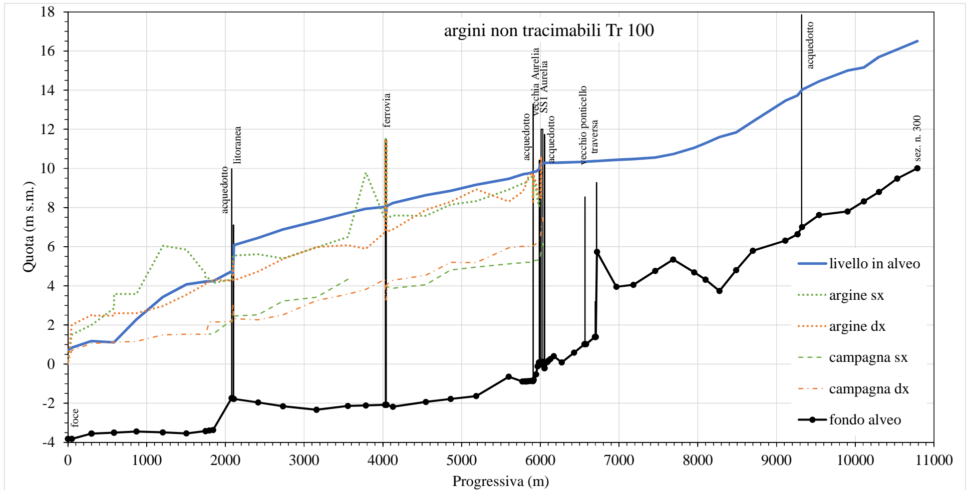
Figura A3.38. Massimi profili idrici ( anotraTr100 )
