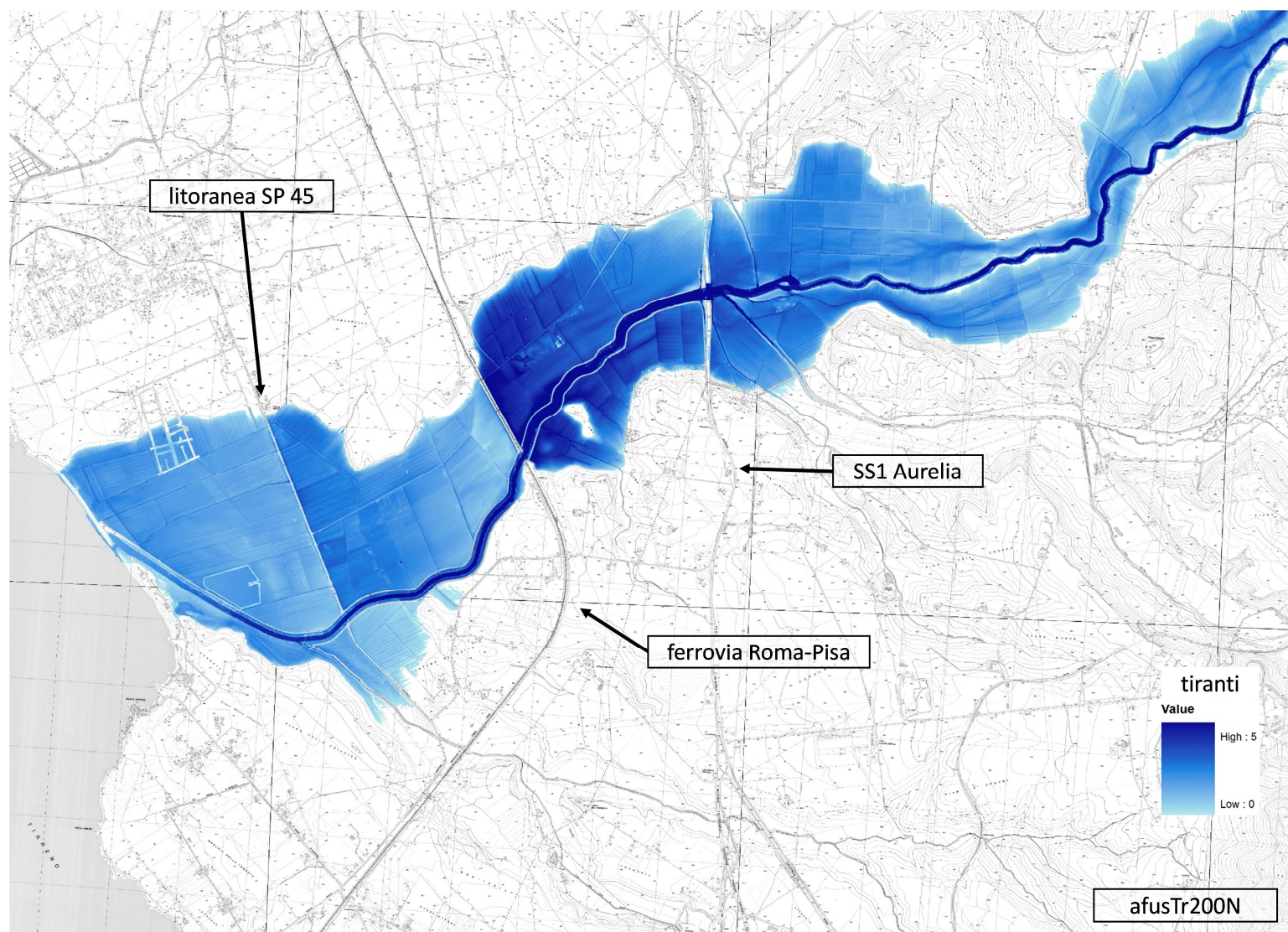
Figura A3.57. Aree inondabili e tiranti idrici ( afusTr200N )
