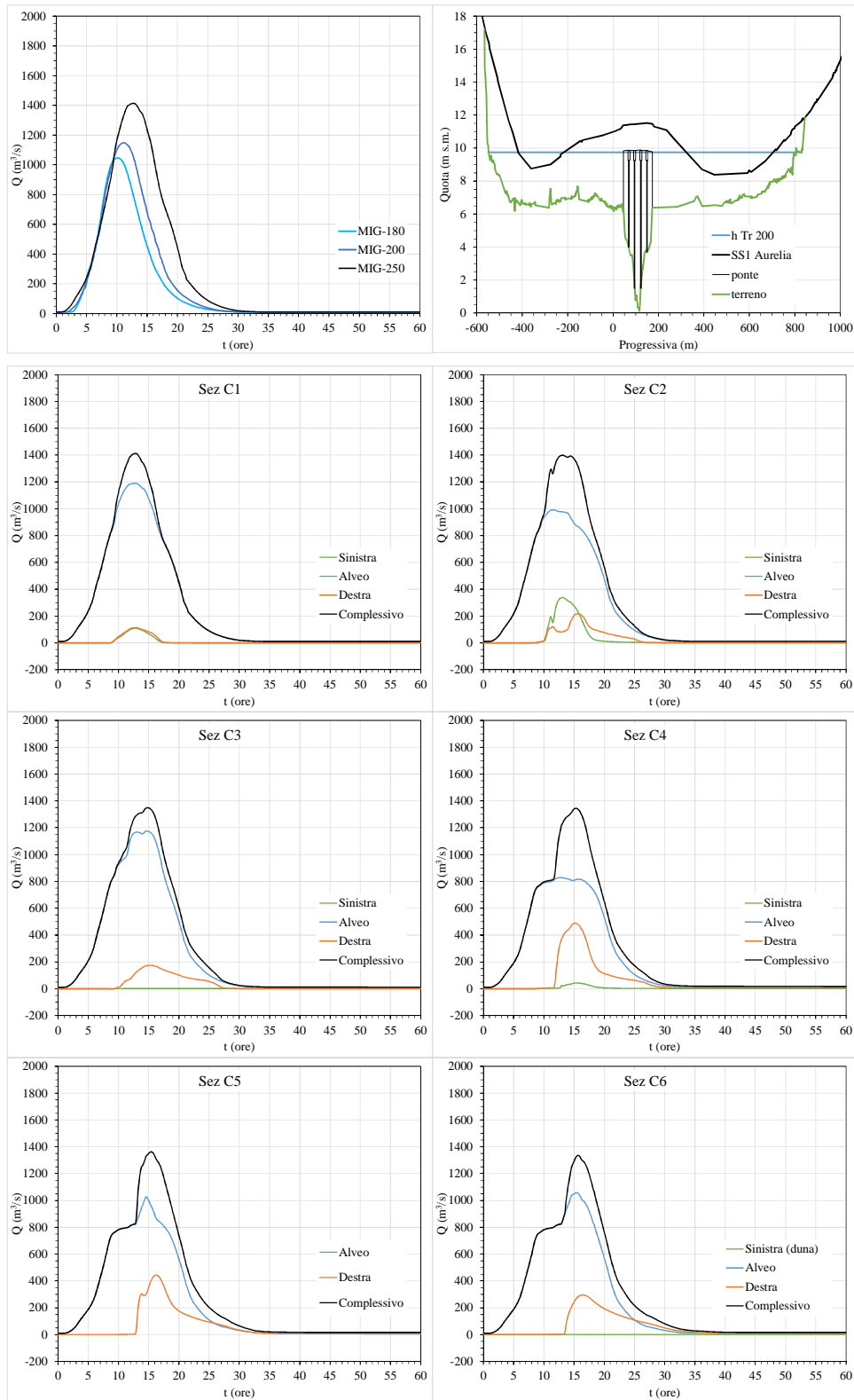
Figura A3.25. Portate e livelli a monte e portate a valle della SS1 Aurelia ( anofusTr200 )
