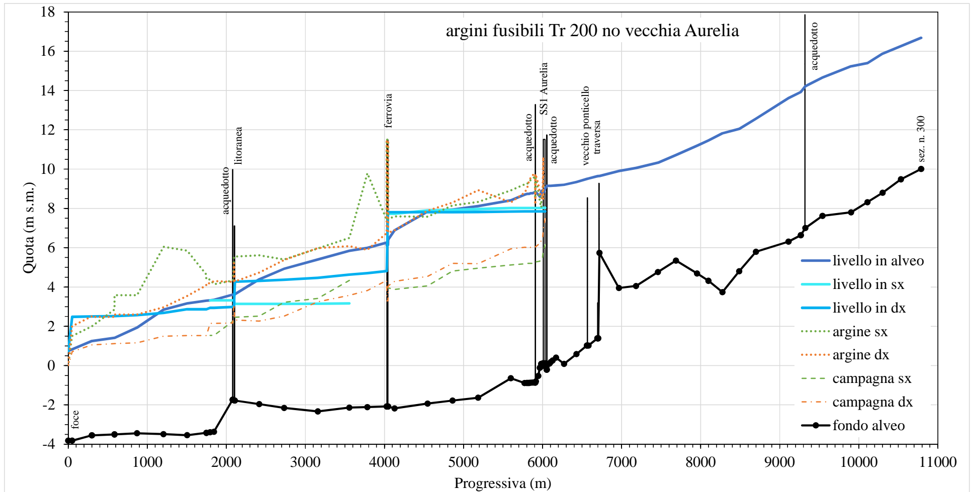
Figura A3.56. Massimi profili idrici ( afusTr200N )
