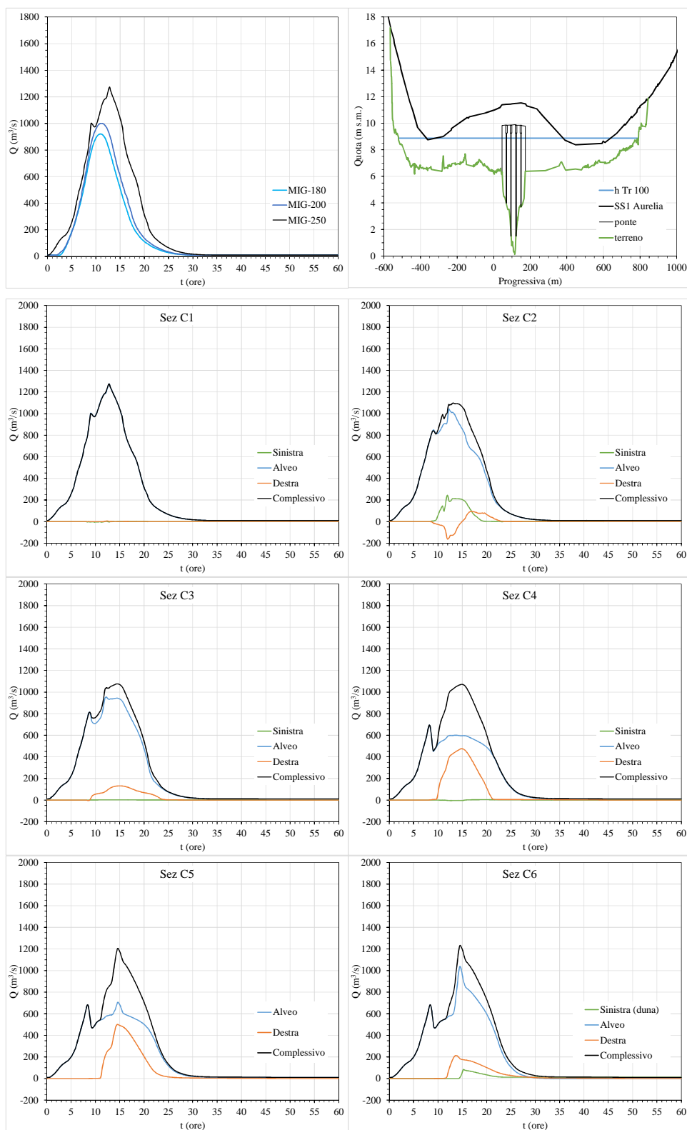
Figura A3.52. Portate e livelli a monte e portate a valle della SS1 Aurelia ( afusTr100M )
