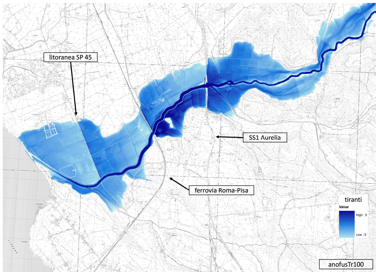
Figura A3.24. Aree inondabili e tiranti idrici ( anofusTr100 )
