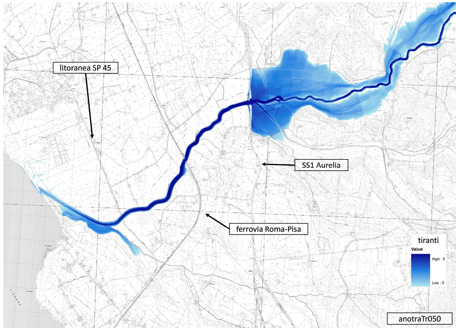
Figura A3.36. Aree inondabili e tiranti idrici ( anotraTr050 )
