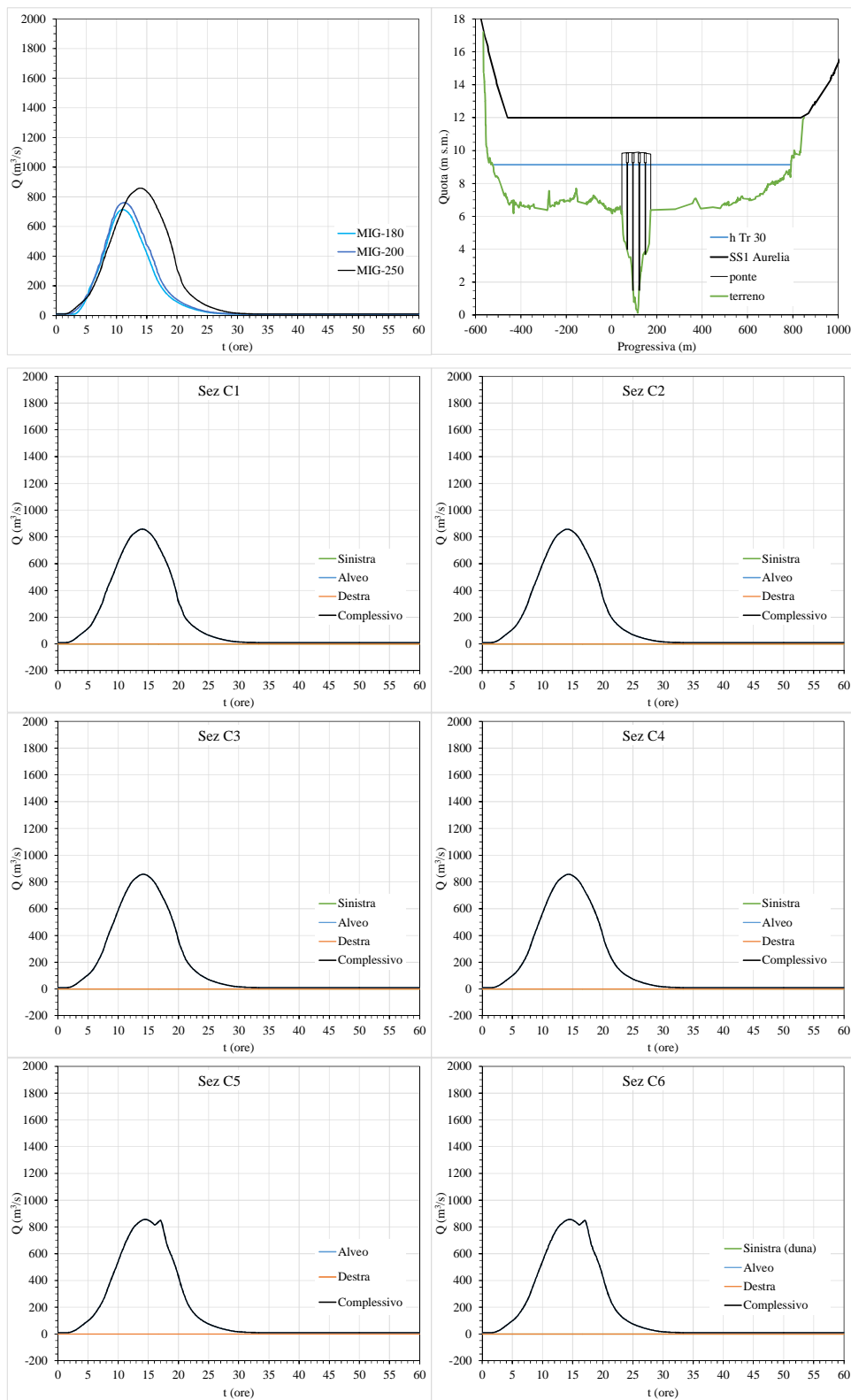
Figura A3.31. Portate e livelli a monte e portate a valle della SS1 Aurelia ( anotraTr030 )
