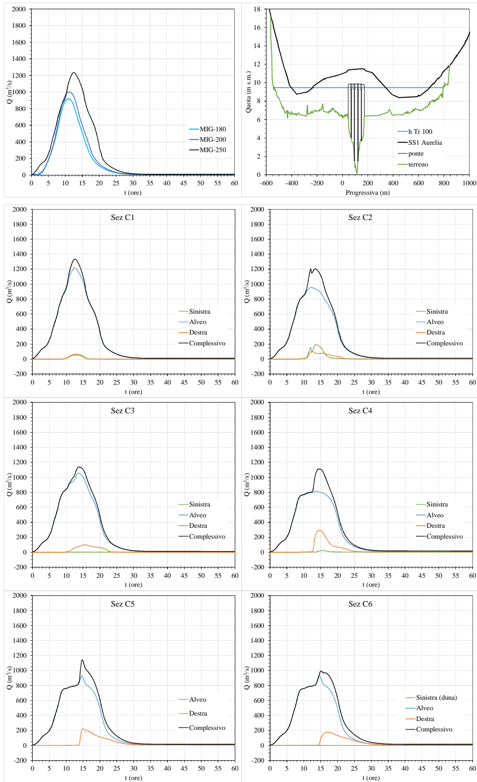
Figura A3.22. Portate e livelli a monte e portate a valle della SS1 Aurelia ( anofusTr100 )
