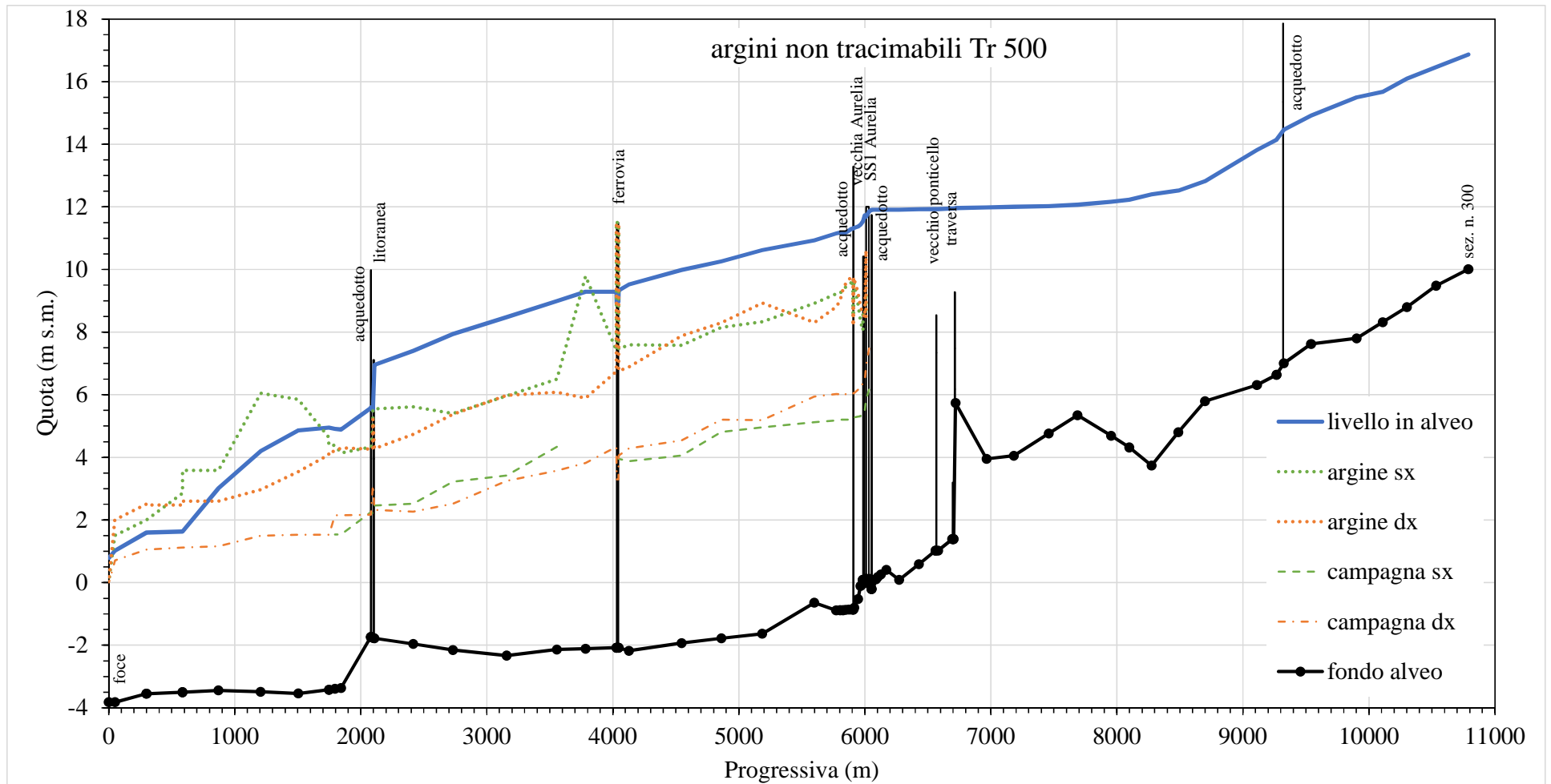
Figura A3.44. Massimi profili idrici ( anotraTr500 )
