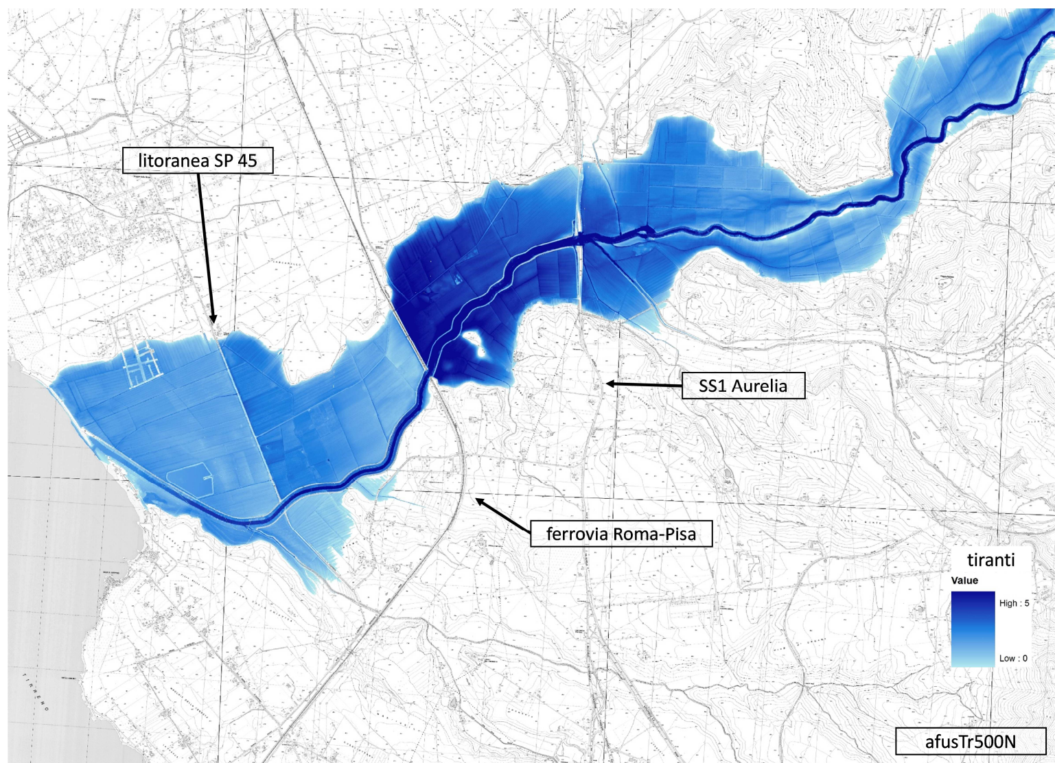
Figura A3.60. Aree inondabili e tiranti idrici ( afusTr500N )
