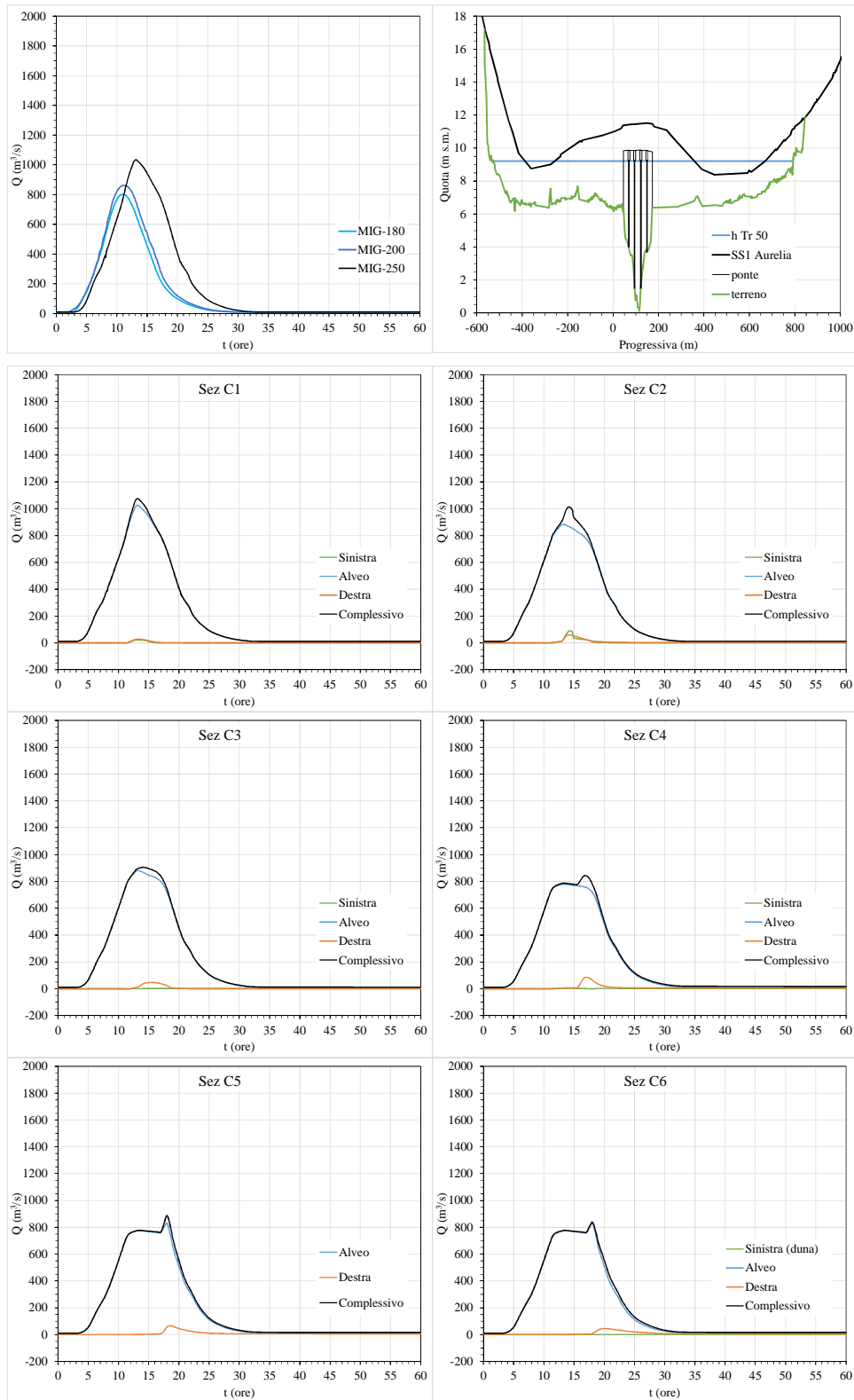
Figura A3.19. Portate e livelli a monte e portate a valle della SS1 Aurelia ( anofusTr050 )
