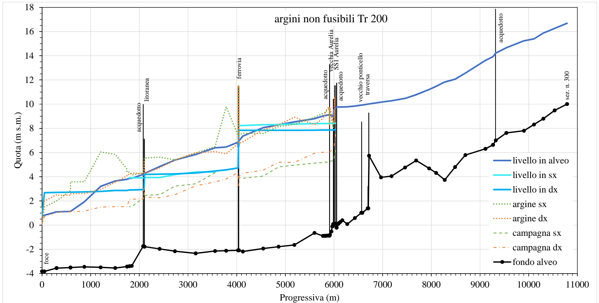
Figura A3.26. Massimi profili idrici ( anofusTr200 )
