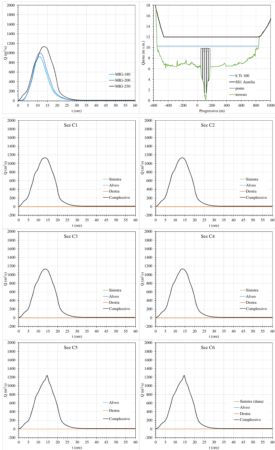
Figura A3.37. Portate e livelli a monte e portate a valle della SS1 Aurelia ( anotraTr100 )
