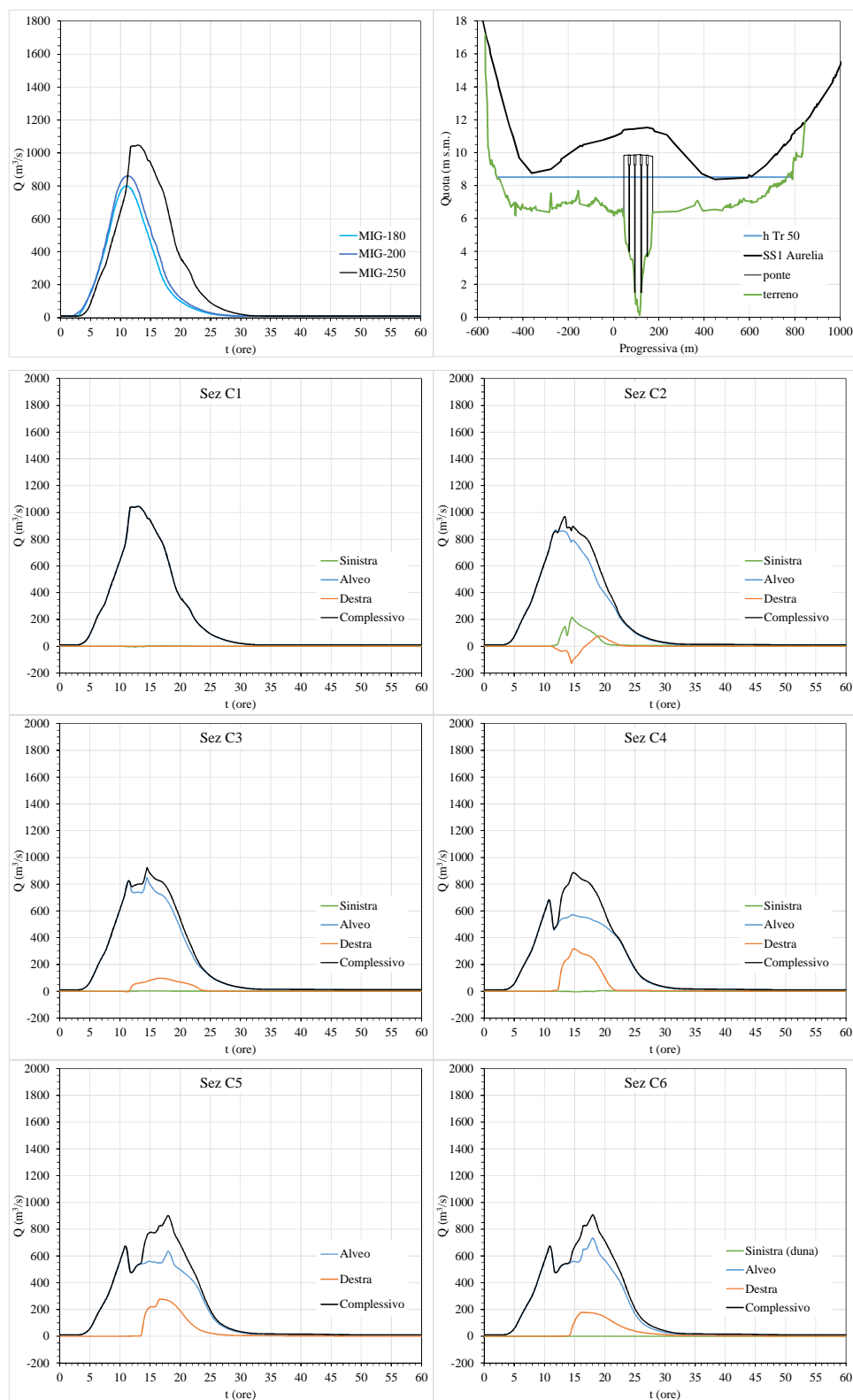
Figura A3.49. Portate e livelli a monte e portate a valle della SS1 Aurelia ( afusTr050M )
