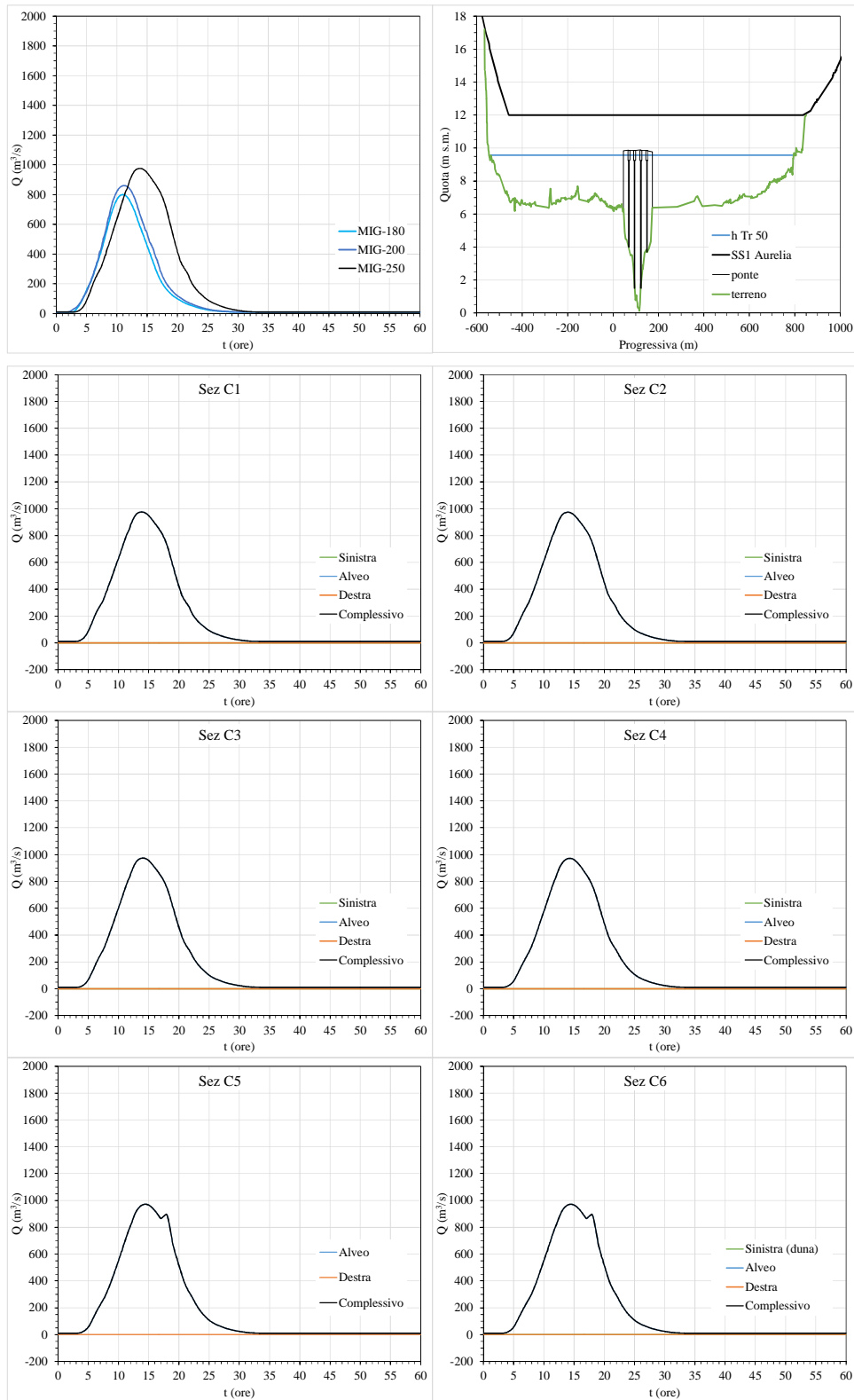
Figura A3.34. Portate e livelli a monte e portate a valle della SS1 Aurelia ( anotraTr050 )
