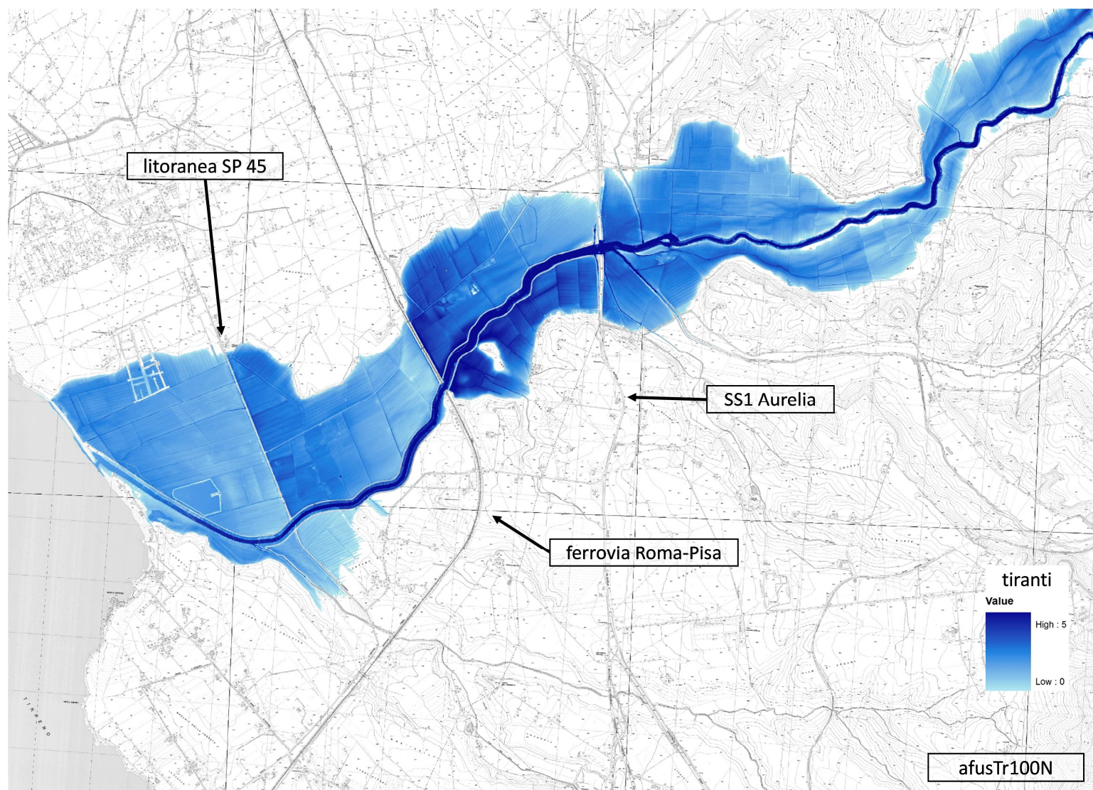
Figura A3.54. Aree inondabili e tiranti idrici ( afusTr100N )
