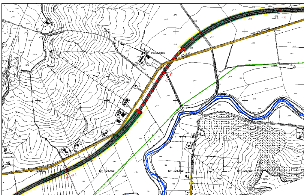
Planimetria di progetto tra i km 10+500 e 13+500
