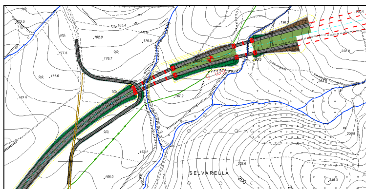
Planimetria di progetto tra i km 4+500 e 5+500
