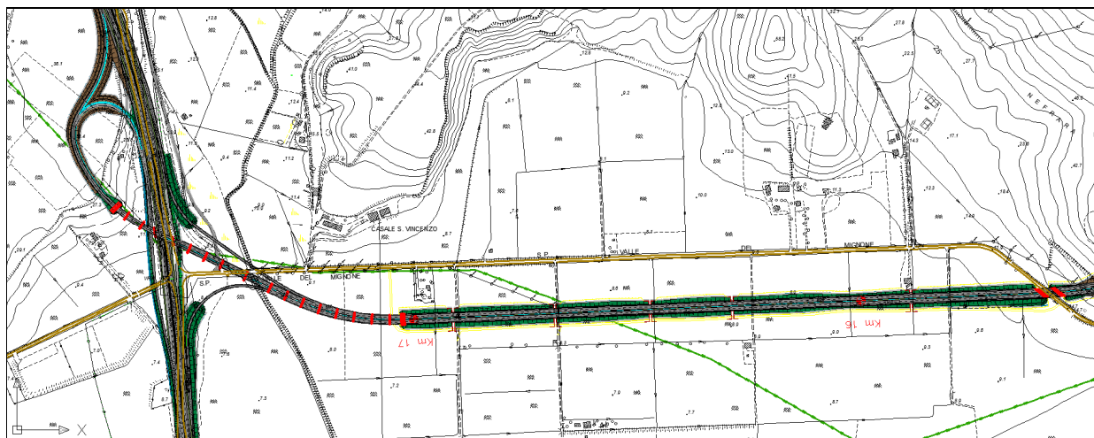
Planimetria di progetto dal km 15+500 in poi
