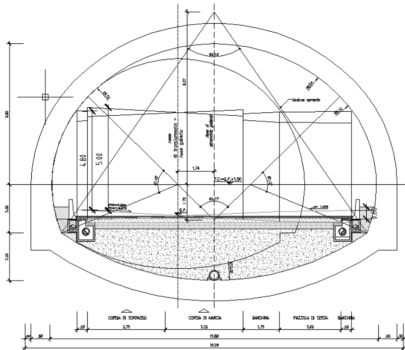
Sezione Tipo in galleria in corrispondenza dell'allargamento per la piazzola di sosta.
