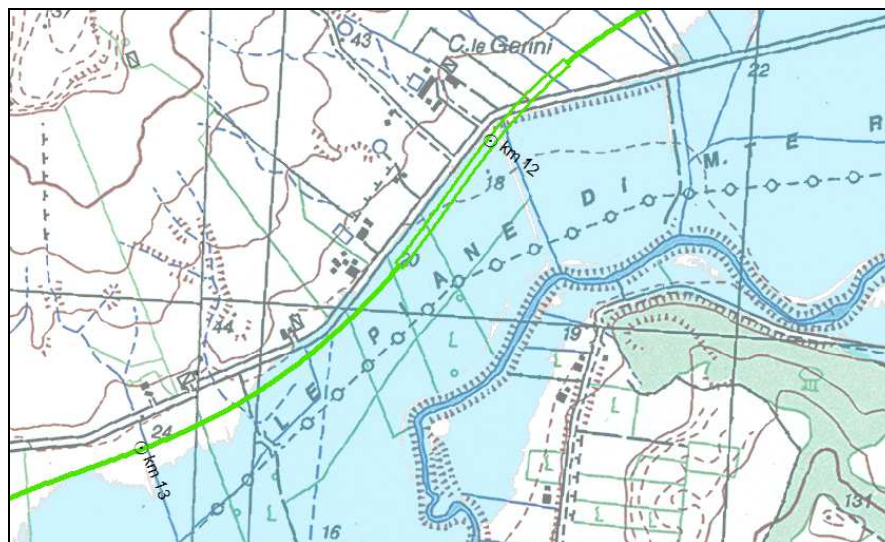
Fascia di esondazione del Mignone tra i km 12+000 e 13+000
