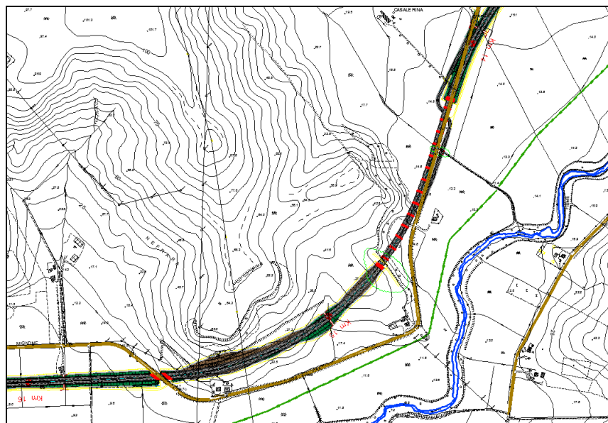
Planimetria di progetto tra i km 14+000 e 16+000
