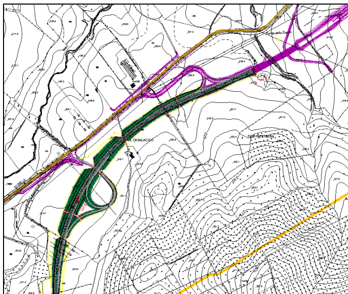
Planimetria di progetto inizio intervento
