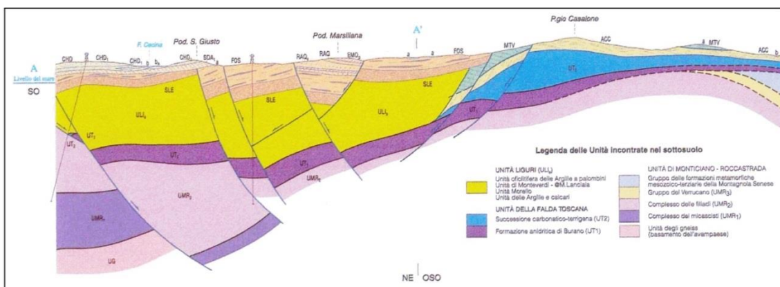
Figura 1-3. Sezione geologica a direzione est-ovest della zona di Radicondoli (dal Foglio 296 Siena della carta geologica d'Italia in scala 1:50.000). La traccia della sezione è mostrata in Figura 1-2.
