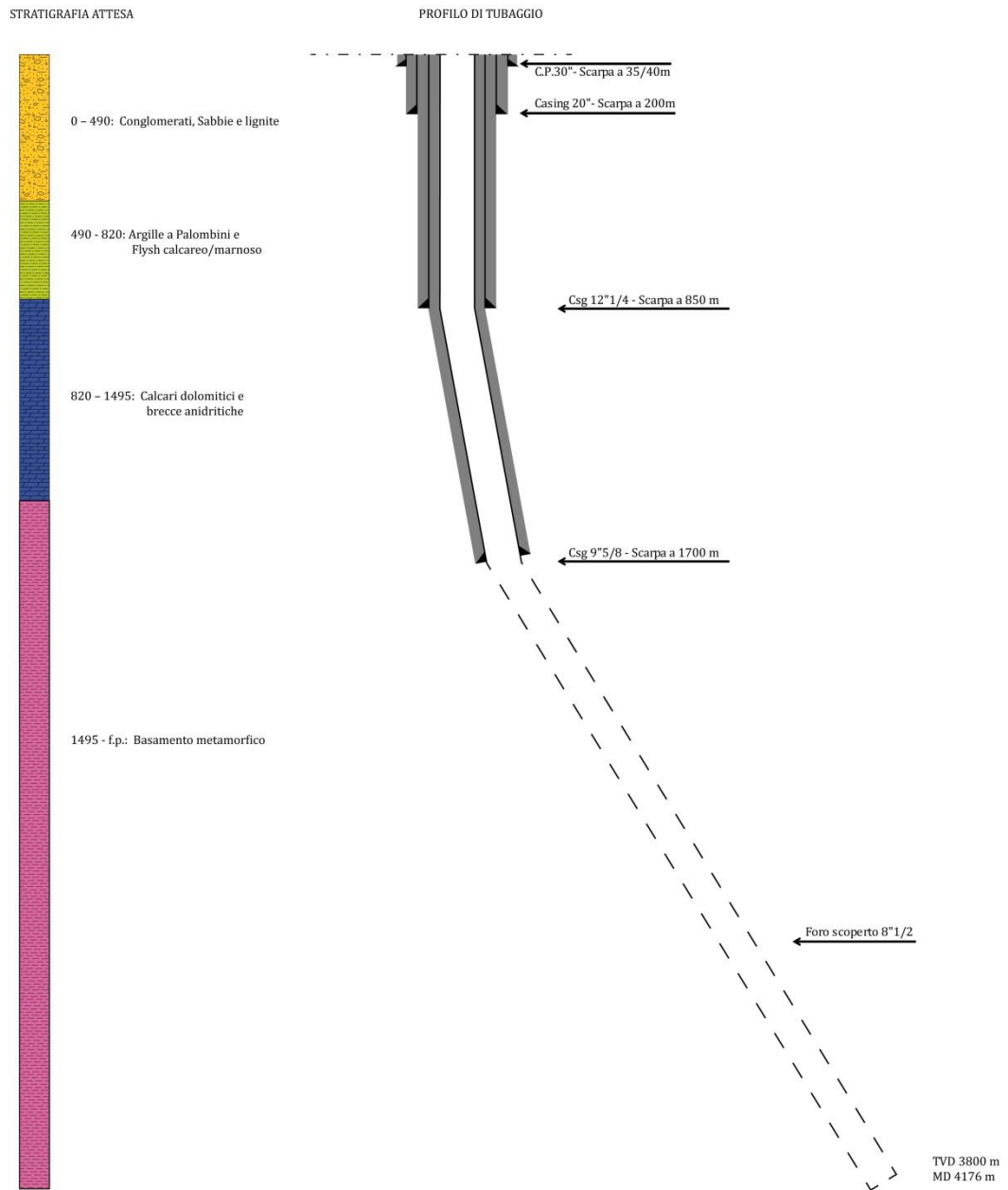
Figura 3-23: Profilo tecnico del pozzo direzionato del polo di reiniezione.
