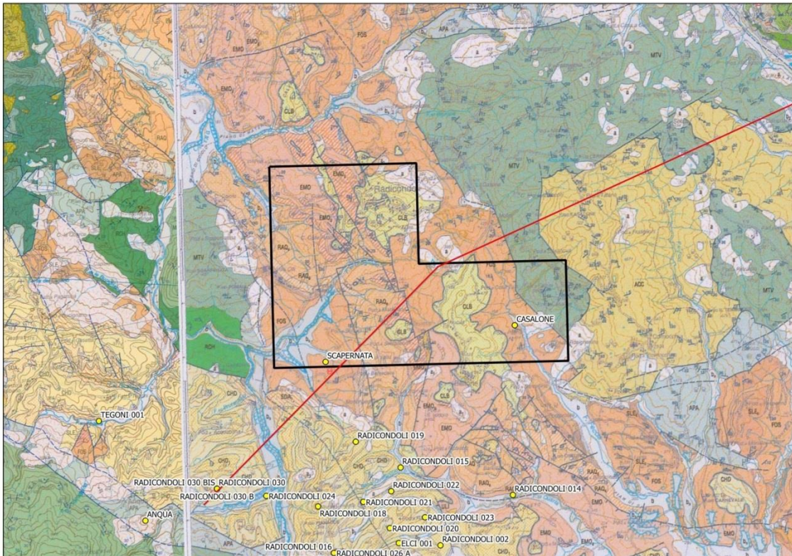
Figura 1-2. Dettaglio sulla zona in esame, del Foglio 295-Pomarance della Carta Geologica d'Italia in scala 1:50.000 (Lazzarotto A. coord., 2002). Sono mostrate inoltre le ubicazioni dei pozzi (Banca dati Nazionale Geotermica) e della sezione geologica di Figura 1-4.
