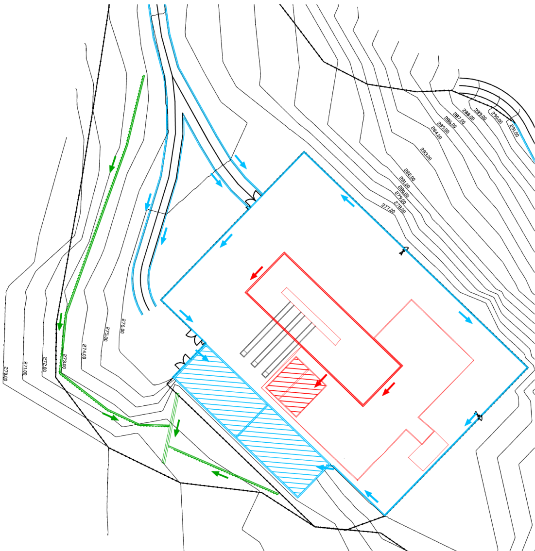
Figura 3-5: Schema della regimazione delle acque all'interno del polo di produzione.
