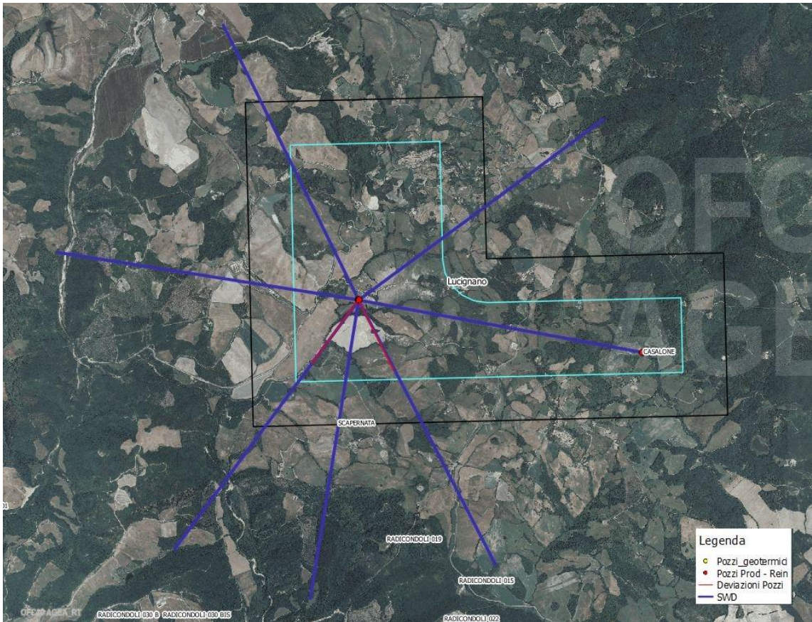
Figura 3-24. Tracce previste per l'acquisizione SWD.
