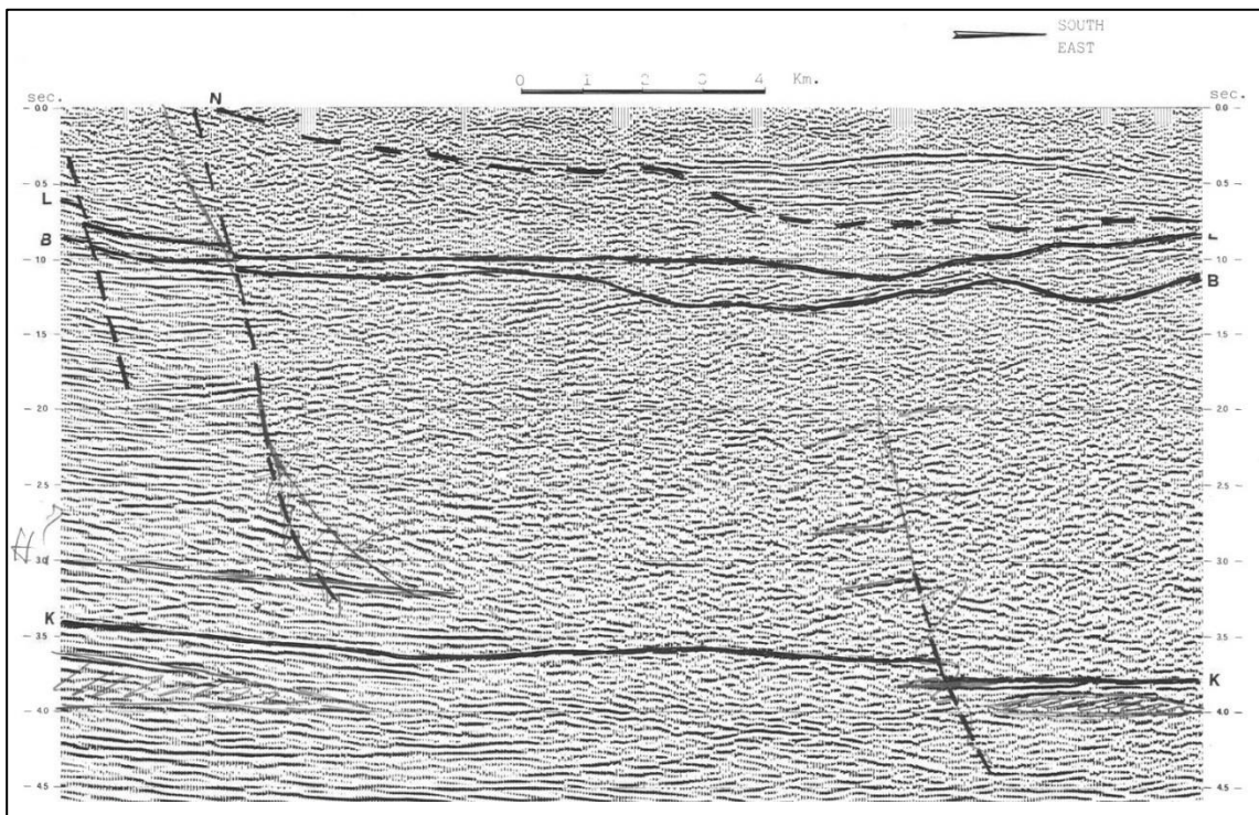
Figura 1-6 Linea LAR7 migrata interpretata (Batini e Nicolich, 1984).
