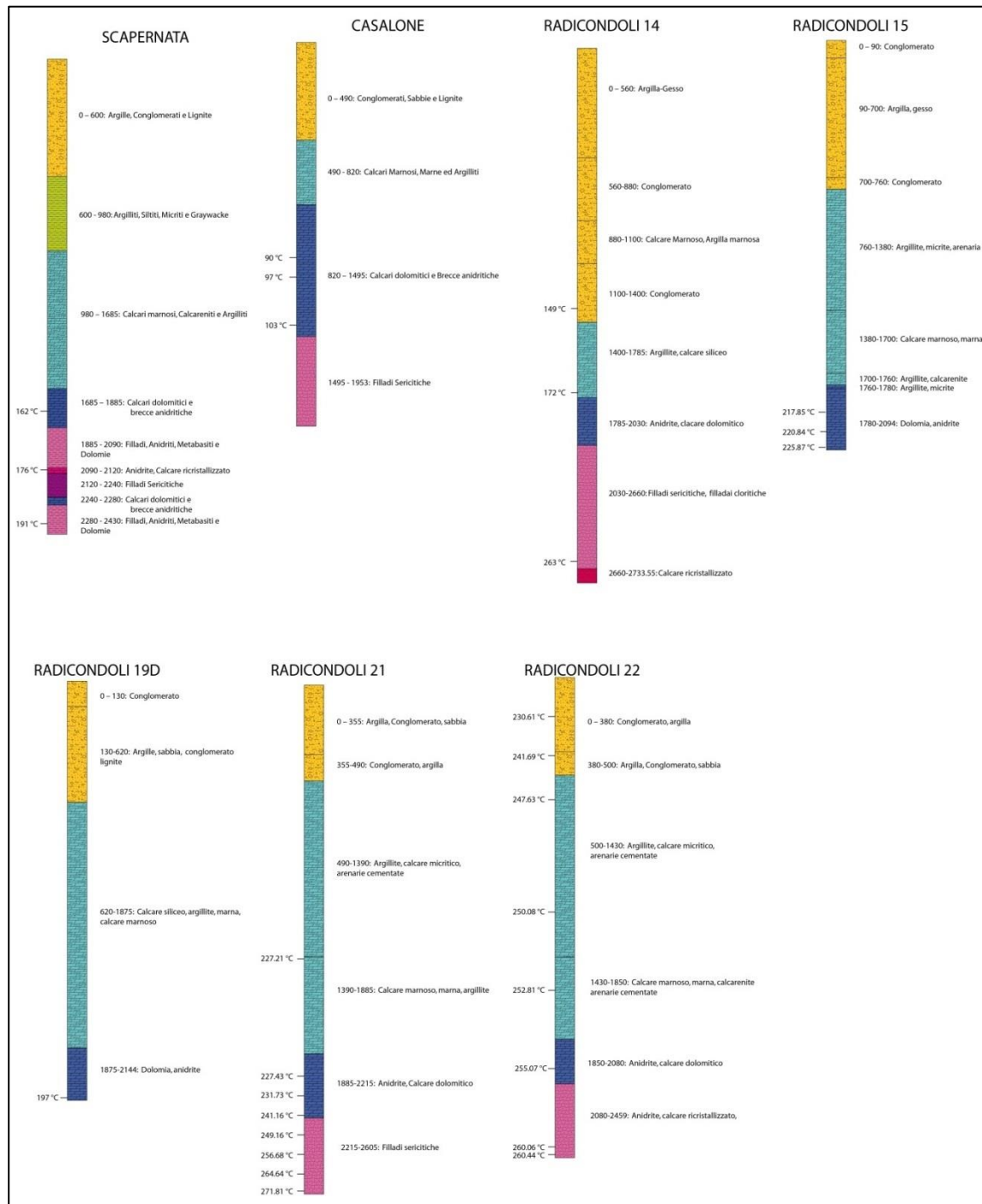
Figura 1-4. Stratigrafia dei pozzi perforati da ENEL (Inventario delle Risorse Geotermiche Nazionali, UNMIG), presenti nell'area del Permesso di Ricerca e nelle zone limitrofe. Le ubicazioni sono mostrate in Figura 1-2.
