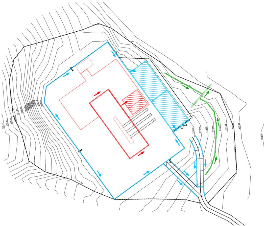
Figura 3-8: Schema della regimazione delle acque all'interno del Polo di Reiniezione.
