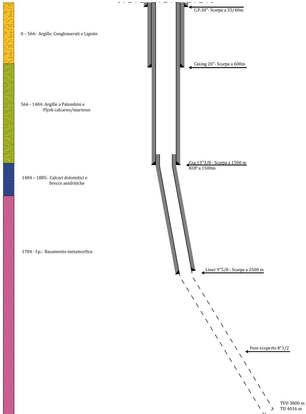
Figura 3-21. Profilo tecnico del pozzo direzionale del polo di produzione.
