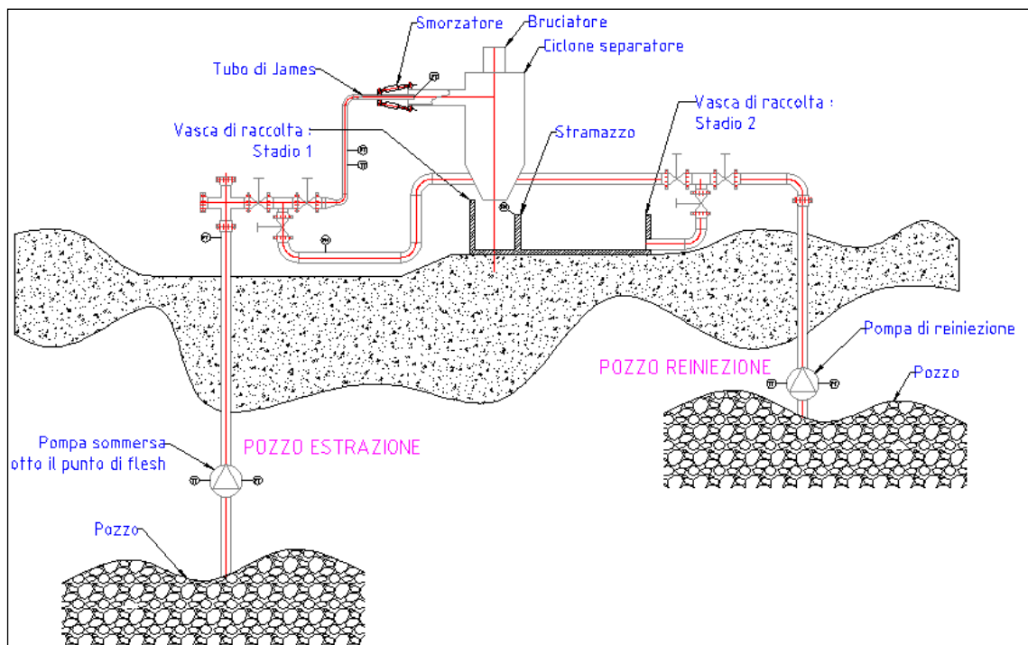
Figura 3-31. Schema di massima impianto per la caratterizzazione dei pozzi geotermici.
