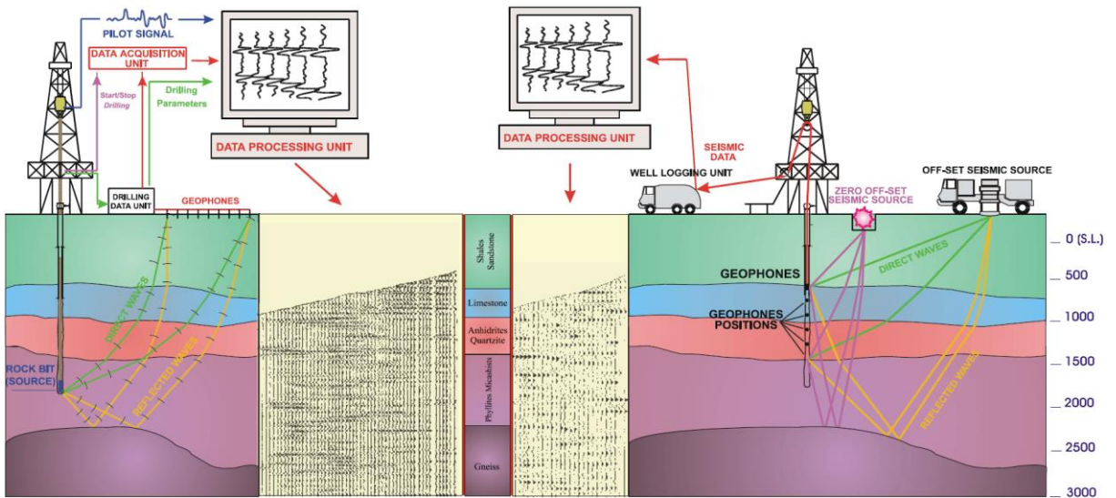
Figura 3-25. Schema esemplificativo di SWD e WSP.
