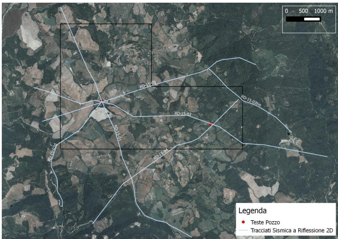
Figura 1-10. Ubicazione dei tracciati delle linee sismiche da acquisire tramite vibroseis.
