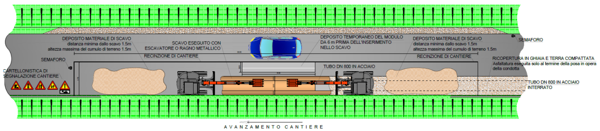
Figura 3-10. Esempio di planimetria di un cantiere mobile.
