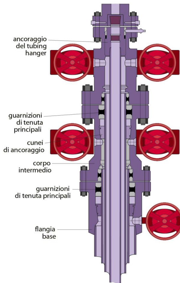
Figura 3-16. Testa pozzo (Enciclopedia degli Idrocarburi, ediz. Treccani).
