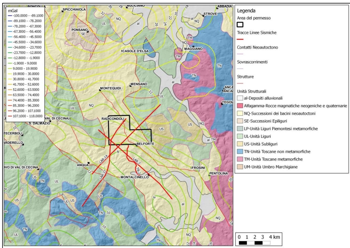
Figura 1-5. Carta dell’anomalia di bouguer (Dettaglio della Carta gravimetrica d’Italia 1:250.000, ISPRA). Vengono inoltre riportate le tracce delle linee sismiche presenti nell’area del Permesso (Fiordelisi et al., 2005; Bertini et al., 2005; Batini e Nicolich, 1984; Batini e Nicolich, 1985).
