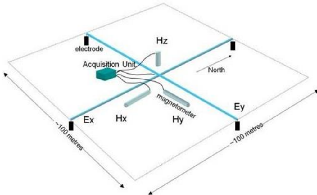
Figura 1-11. Layout di acquisizione di una stazione MT.
