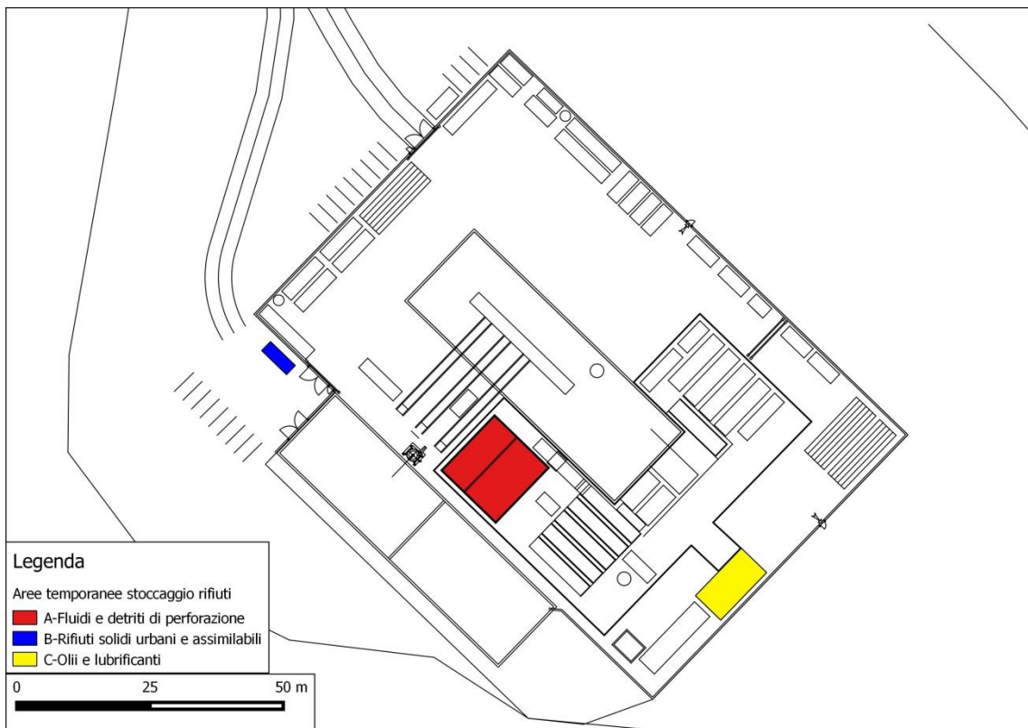
Figura 3-33. Ubicazione delle aree di stoccaggio temporaneo dei rifiuti nel cantiere di perforazione Lucignano 1.
