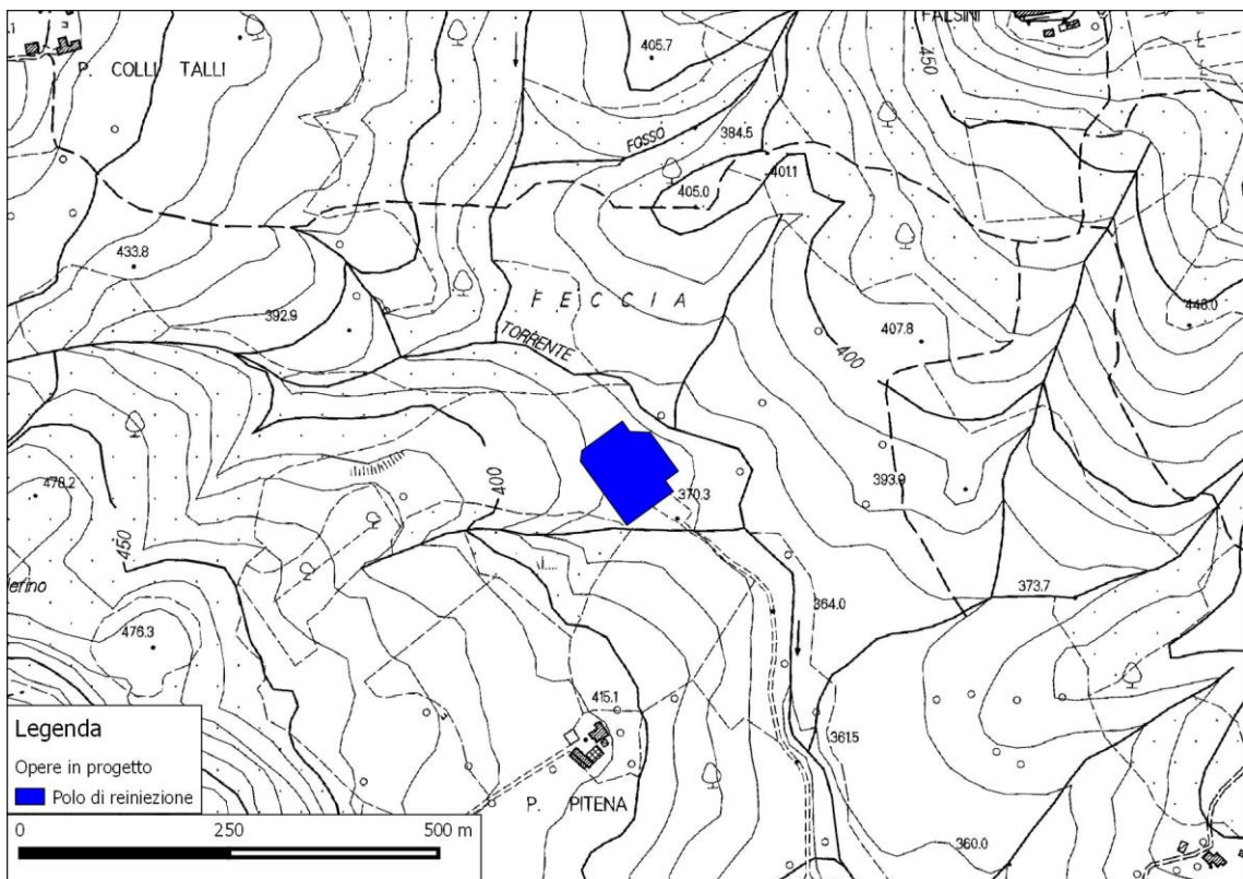
Figura 2-13. Ubicazione su CTR del polo di reiniezione LUCIGNANO 2.
