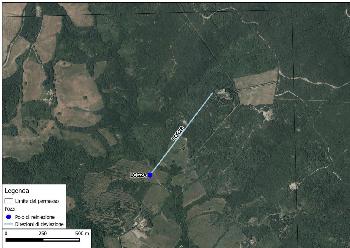
Figura 3-12. Ubicazione dei pozzi di reiniezione con le direzioni di deviazioni proposte.
