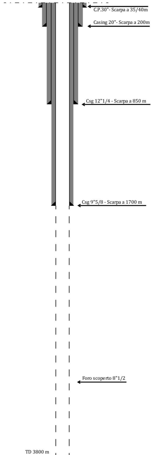
Figura 3-22. Profilo tecnico del pozzo verticale del polo di reiniezione.
