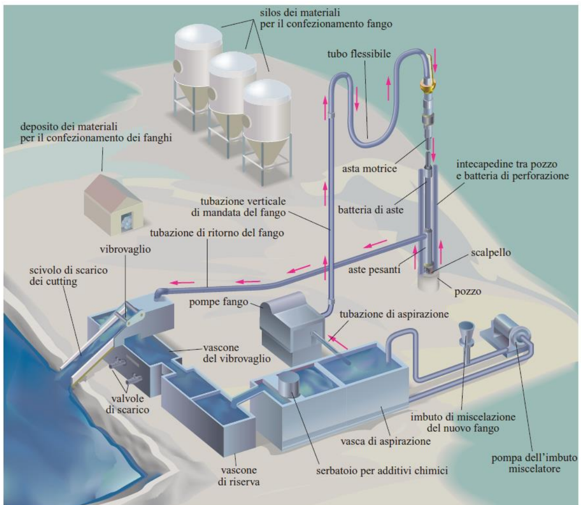
Figura 3-15. Schema di circolazione del fango (Enciclopedia degli Idrocarburi, ediz. Treccani).
