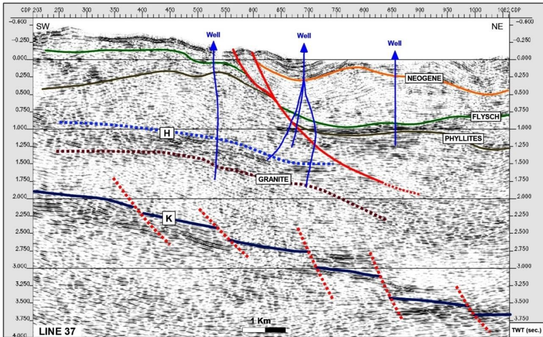
Figura 1-7. Linea LAR37 riprocessata, migrata e interpretata con l'ausilio di alcuni pozzi (Fiordelisi et al., 2005).
