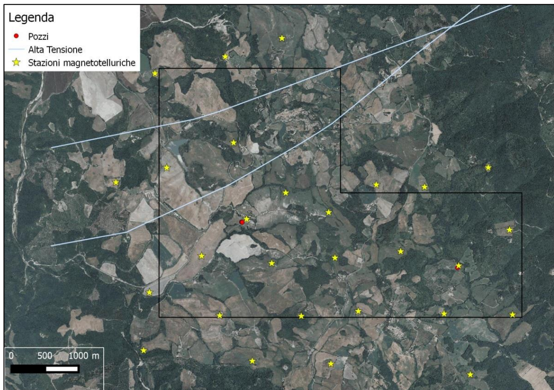
Figura 1-12. Ubicazione delle stazioni di acquisizione MT.
