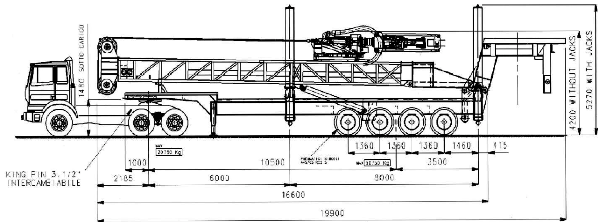
Figura 3-32. Schema del mezzo di trasporto della sonda.
