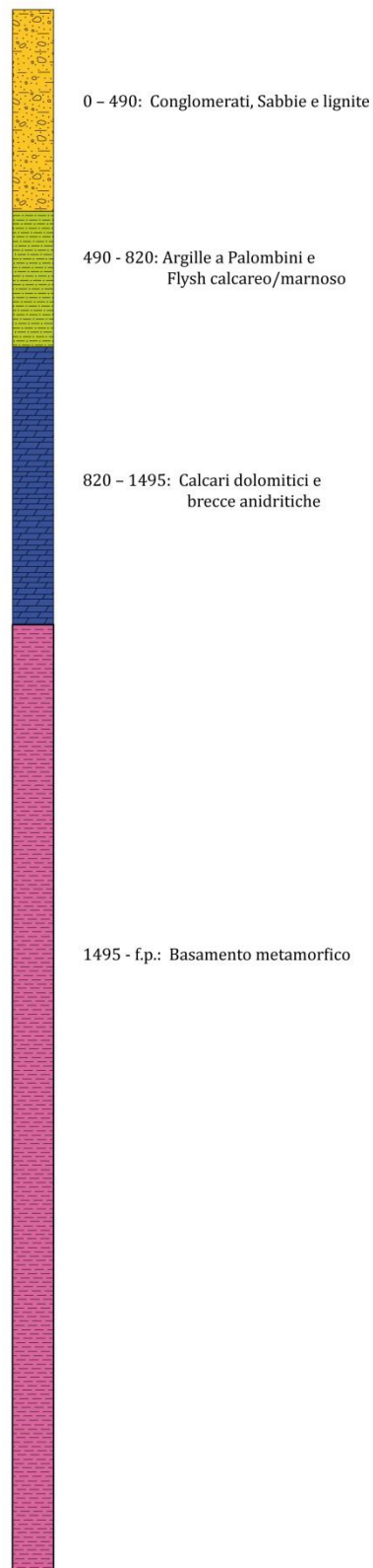
Figura 3-22. Profilo tecnico del pozzo verticale del polo di reiniezione.
