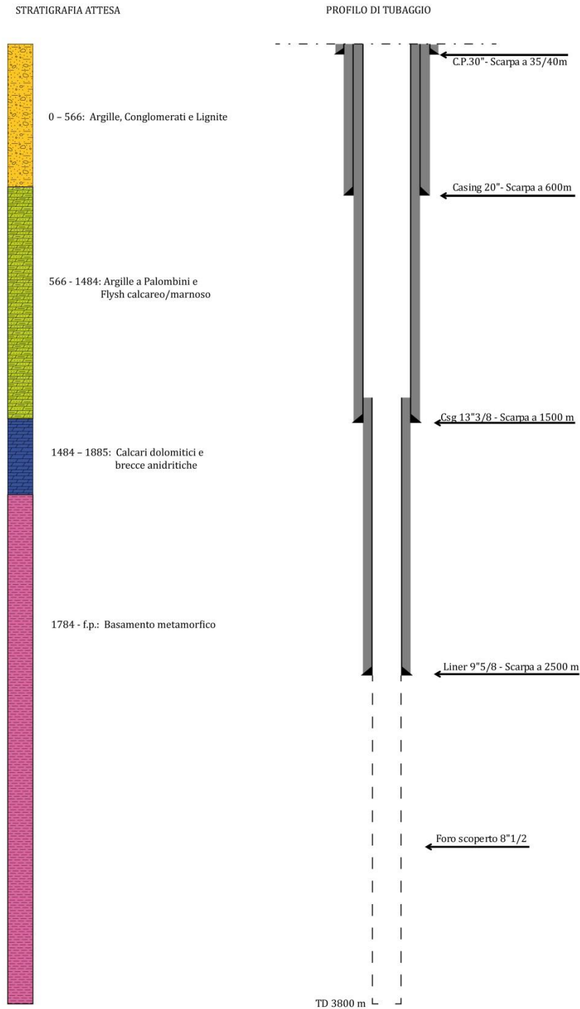
Figura 3-20. Profilo tecnico del pozzo verticale del polo di produzione.
