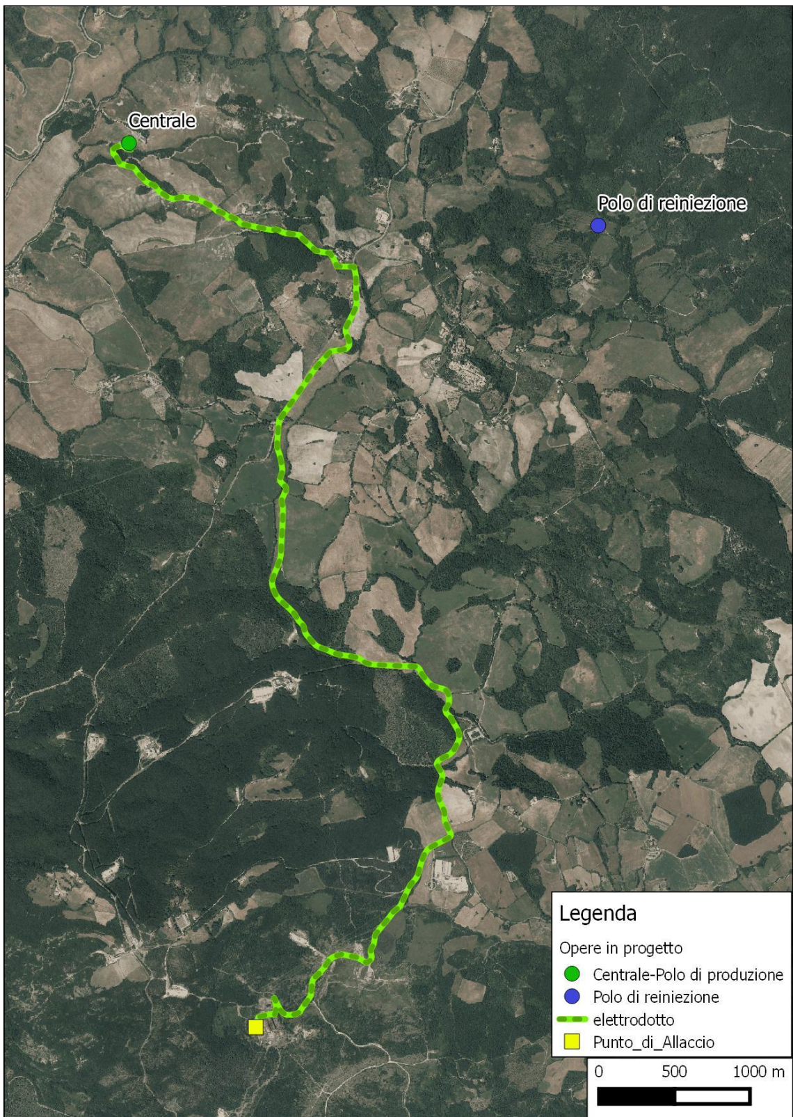
Figura 2-16. Tracciato dell'elettrodotto su ortofoto.
