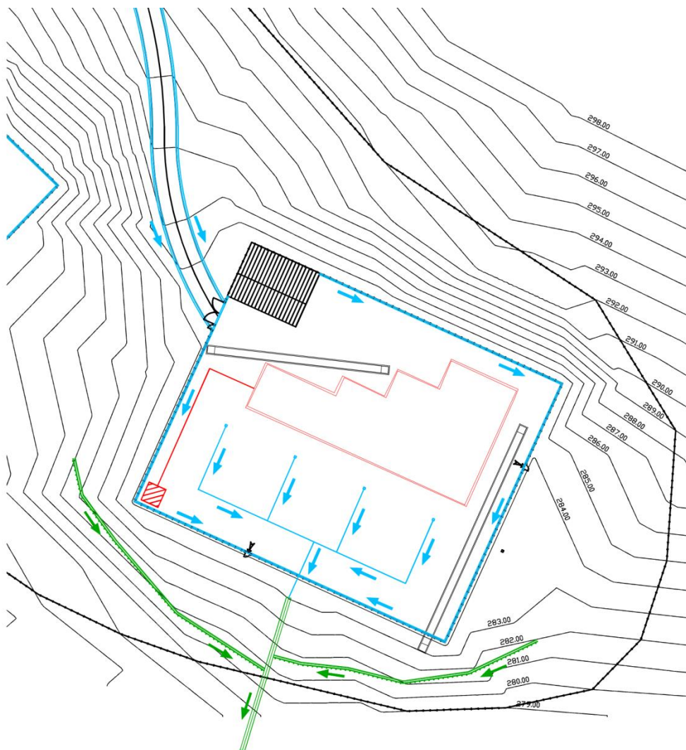
Figura 3-2. Sistema di regimazione idrica dell'area dell'impianto di produzione.
