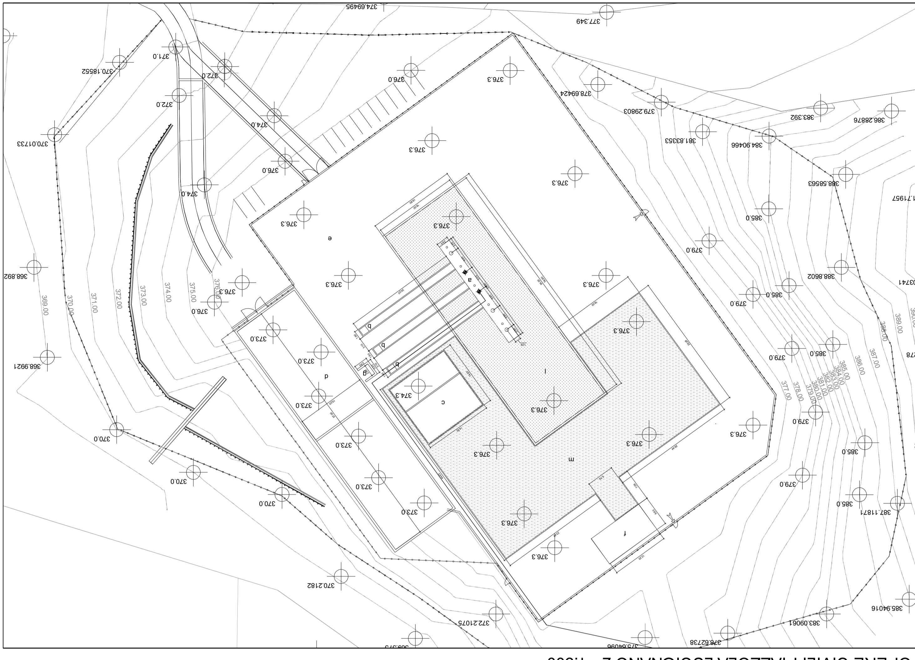
OPERE CIVILI PIAZZOLA LUCIGNANO 2 - 1:500
