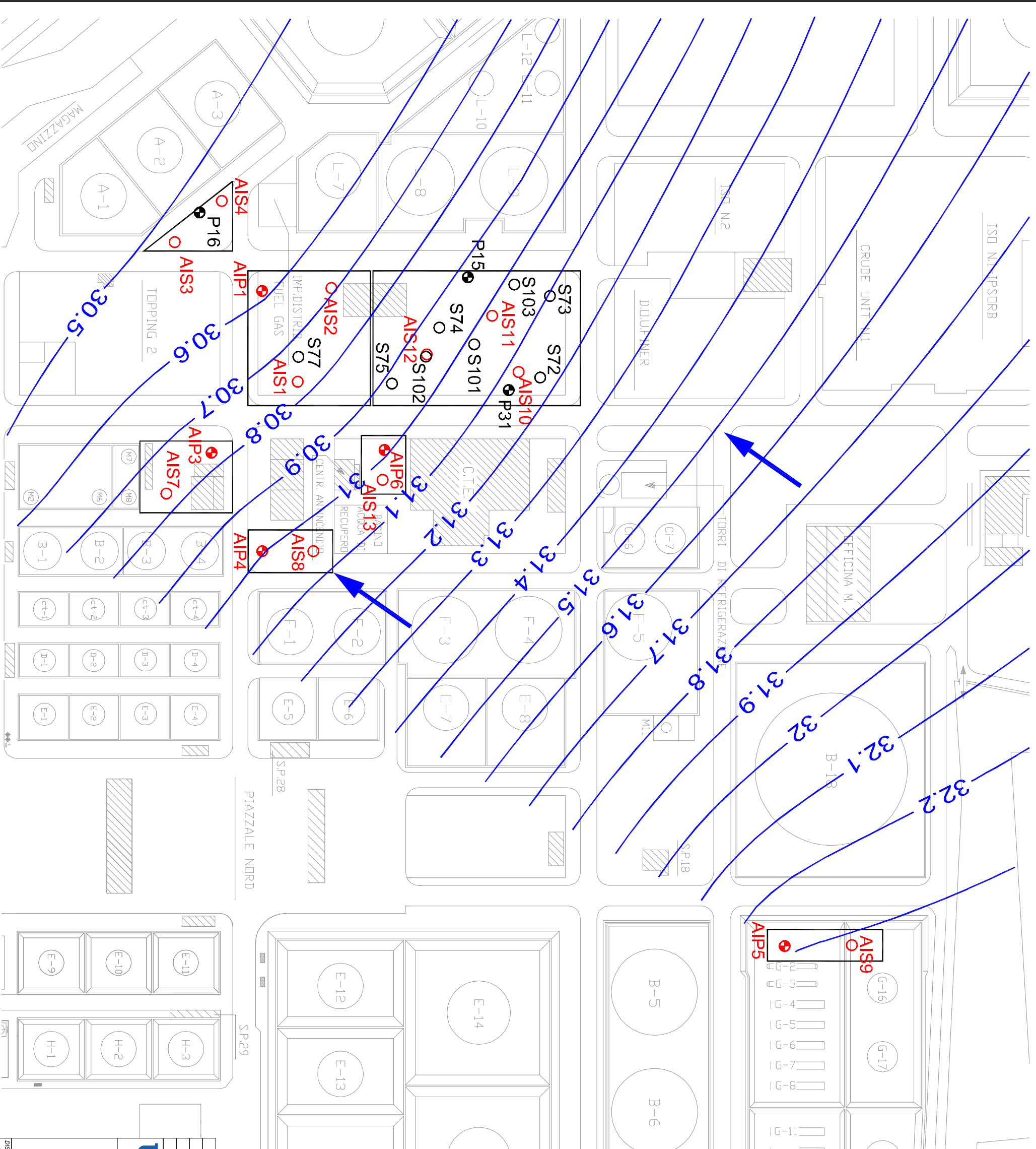
FIGURA 03: MAPPA DELLE ISOFREATICHE (MARZO 07)
