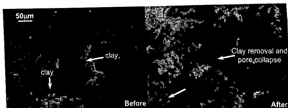
Figura 1. Monitoraggio della variazione della microstruttura di un'arenaria argillosa prima (sinistra) e dopo (destra), l'iniezione di un fluido ricco in CO 2 . L'arenaria è caratterizzata da una media porosità e bassi valori elasto-meccanici. L'iniezione del fluido è eseguita sotto condizioni di temperatura e pressioni (litostatiche e pressione di fluido di poro) tipiche di reservoir (da Vanorio, 2015)
