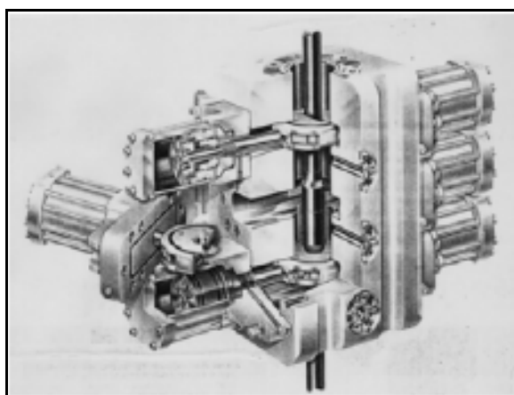
Figura 5: esempio di B.O.P. a ganasce
