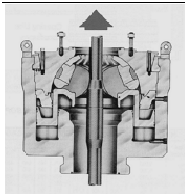
Figura 4: esempio di B.O.P. anulare
