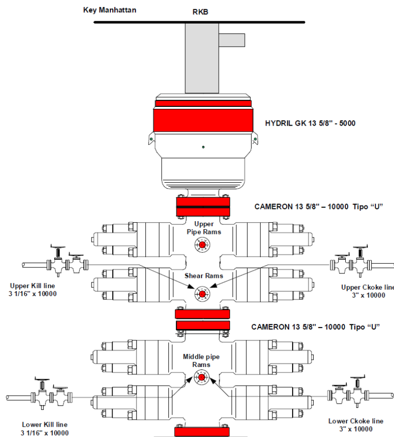
Figura 6 – BOP stack per fase 12 ¼" e 8 ½"
