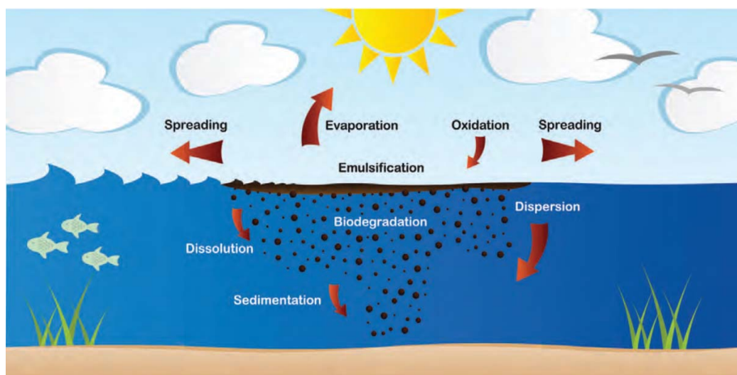
Figura 8 - Processi di degradazione ai quali sono sottoposti gli idrocarburi in ambiente marino
