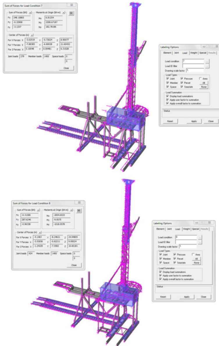
FIGURA 3. Modello di verifica della Torre per effetto dell’azione da vento eseguito da DRILLMEC S.p.A.
