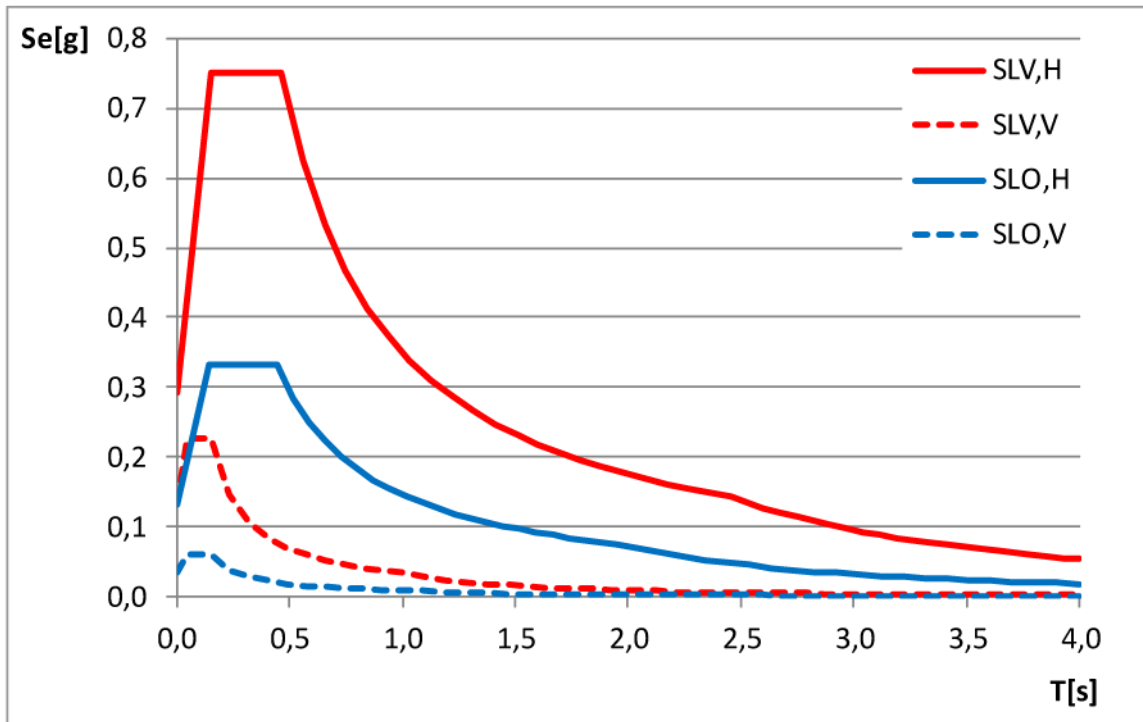
FIGURA 2. Spettri di risposta elastici S_e (componente orizzontali H e verticali V) in funzione del periodo di vibrazione T della struttura per gli Stati Limite di Salvaguardia della Vita (SLV) e di Operatività (SLO) per sottosuolo di classe C.
