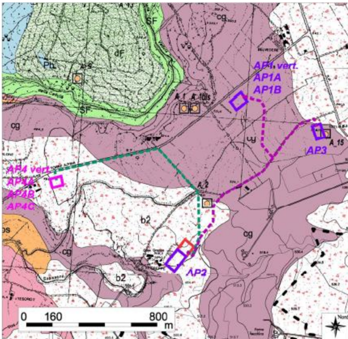
FIGURA 1. Planimetria dell'impianto geotermico pilota di Torre Alfina.
